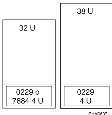
Figura 5. Codi de característica 7884: 9406-520 i 9111-520 en un bastidor
