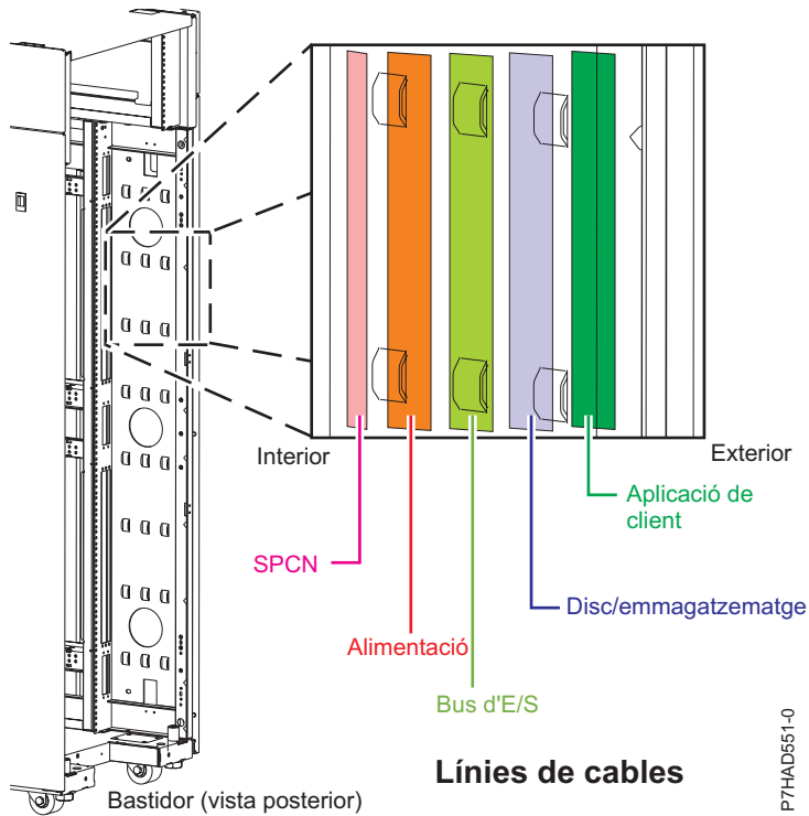
Figura 134. Ponts portacables
