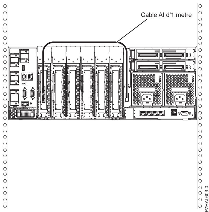
Figura 147. Adaptador SAS a les ranures de disc SAS internes mitjançant el port SAS extern del sistema
