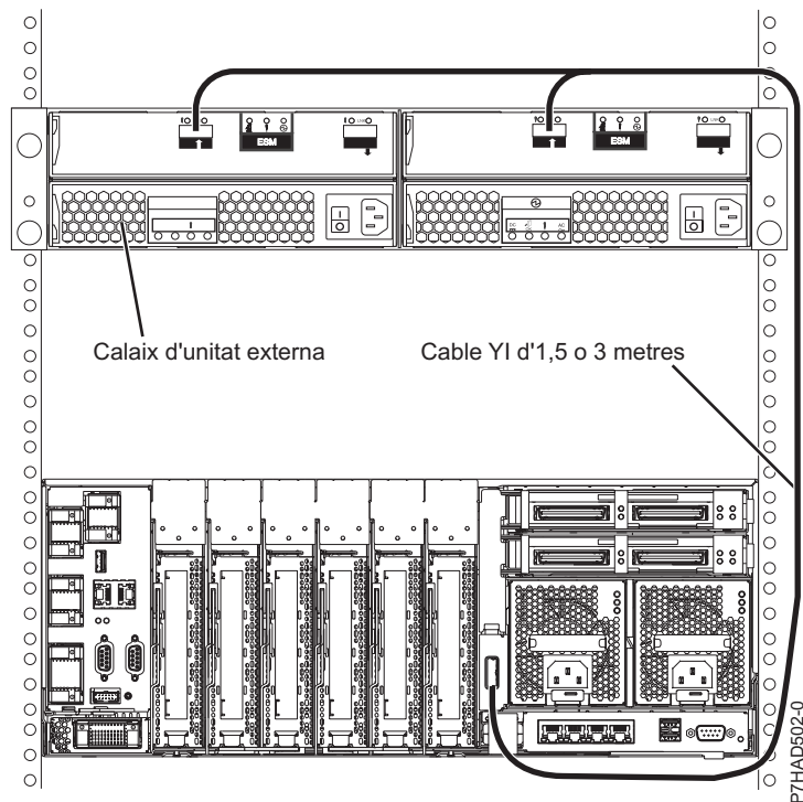
Figura 146. Un port d'adaptador SAS extern del sistema a un calaix d'expansió de discs (models 9117-MMB i 9179-MHB)
