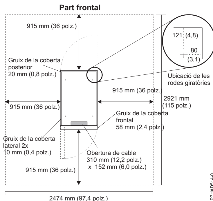
Figura 27. Ubicació de les rodes giratòries i espais lliures per al servei tècnic dels bastidors 7014-T00, 7014-T42 i 0553
