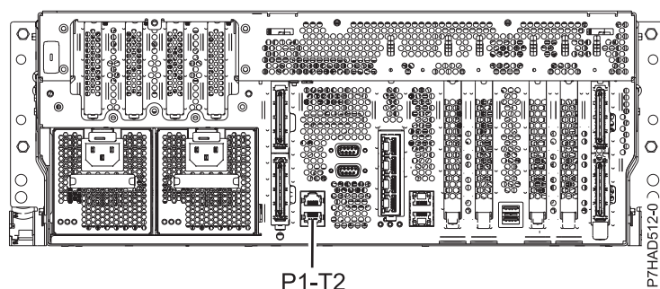
Figura 137. Vista posterior del model 8202-E4B, 8202-E4C, 8202-E4D, 8205-E6B, 8205-E6C i 8205-E6D amb la ubicació d'instal·lació dels cables
