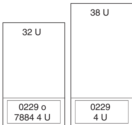
Figura 10. Codi de característica 7884: 9406-520 i 9111-520 en un bastidor
