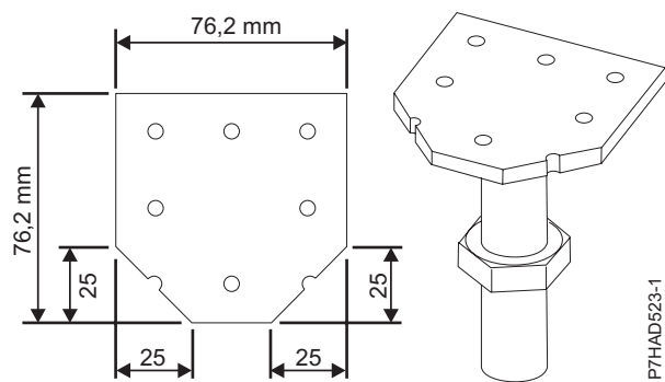
Figura 4. Dimensions de les obertures del pedestal
