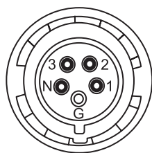
Figura 36. Patilla de connexió
