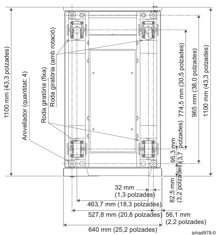
Figura 26. Ubicacions de rodes giratòries i anivelladors
