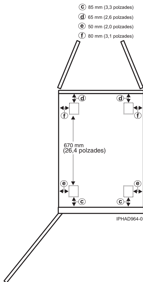
Figura 25. Ubicacions de les rodes giratòries del model 0555 i 7014-S25
