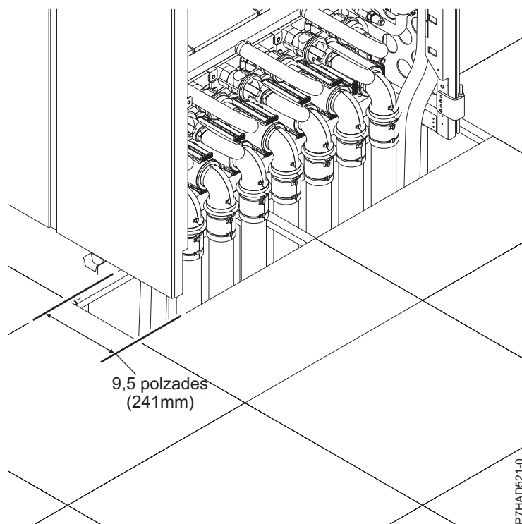
Figura 3. Obertura al terra
