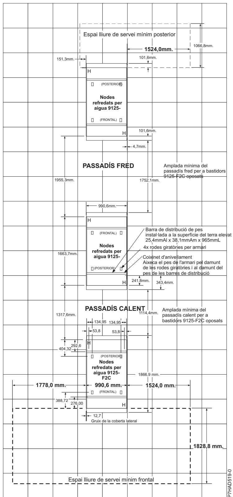
Figura 1. Espai lliure per al servei tècnic per a un sol bastidor - Passadís calent i passadís fred
