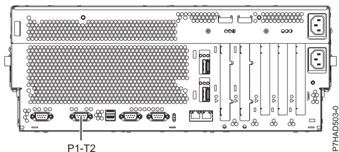
Figura 134. Vista posterior del model 8233-E8B i 8236-E8C amb la ubicació d'instal·lació dels cables
