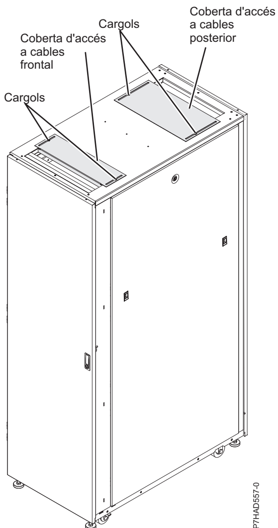
Figura 31. Tapes d'accés als cables
