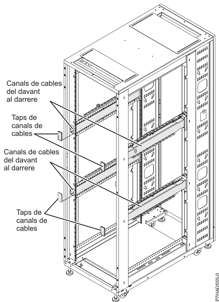
Figura 29. Connexió dels cables al bastidor
