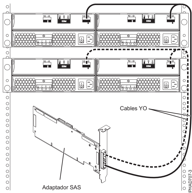
Figura 146. Un adaptador SAS a dos calaixos d'expansió de discs
