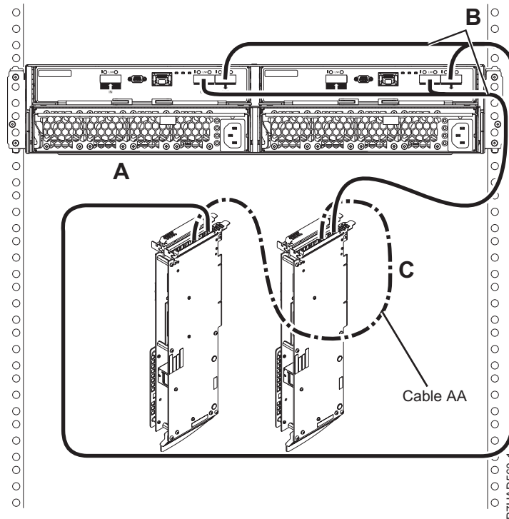
Figura 172. Connexió de mode 1 d'un calaix 5887 utilitzant cables YO a adaptadors SAS duals
