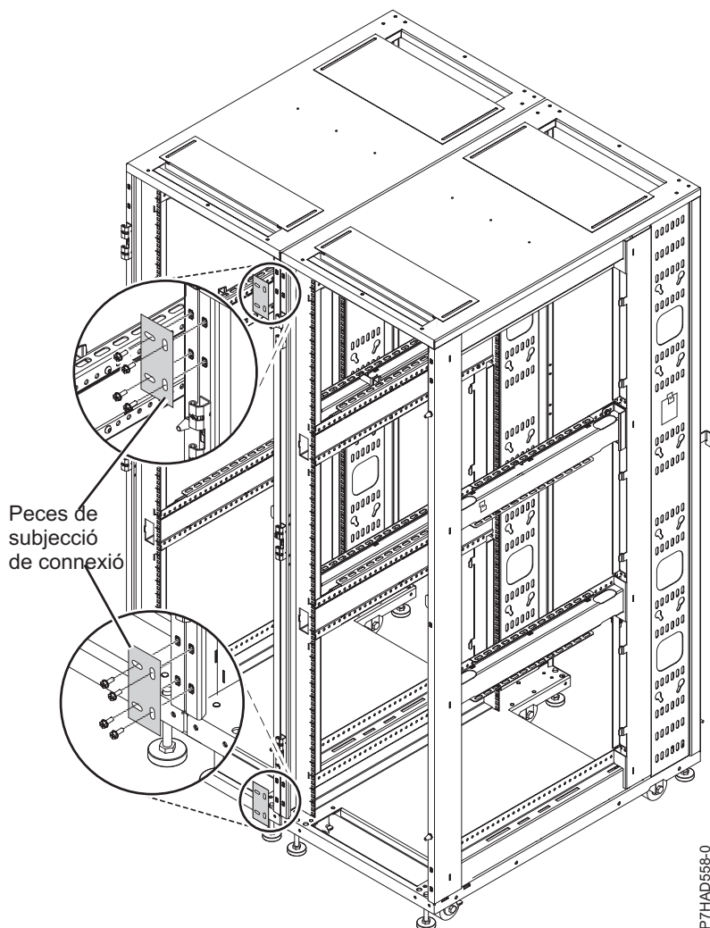
Figura 33. Peces de subjecció de connexió
