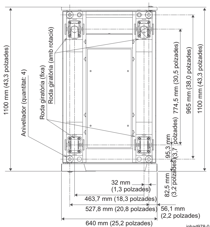
Figura 9. Ubicacions de rodes giratòries i anivelladors
