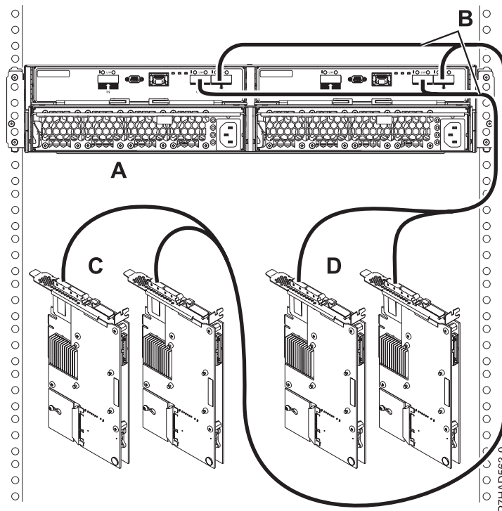
Figura 170. Connexió de dos parells d'adaptadors FC 5805 o FC 5903 a un calaix 5887 a través del mode 2
