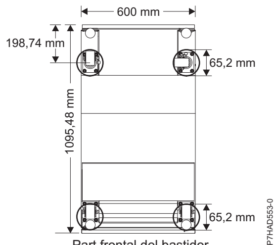
Figura 28. Ubicació de les rodes giratòries
