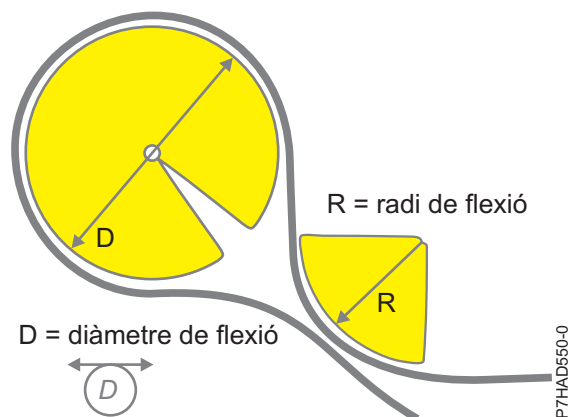
Figura 140. Radi flexionat del cable
