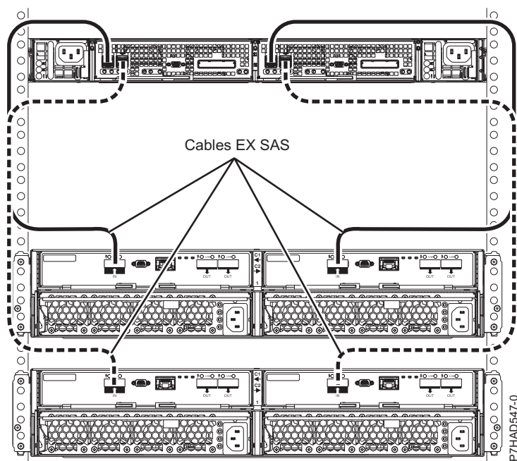
Figura 178. Connexió de dos calaixos 5887 mitjançant cables HD EX a un EDR1
