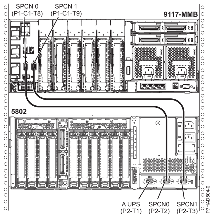
Figura 135. Vista posterior de la ubicació d'instal·lació dels cables per als models 8412-EAD, 9117-MMB, 9117-MMC, 9117-MMD, 9179-MHB, 9179-MHC, 9179-MHD i 5208 o 5877
