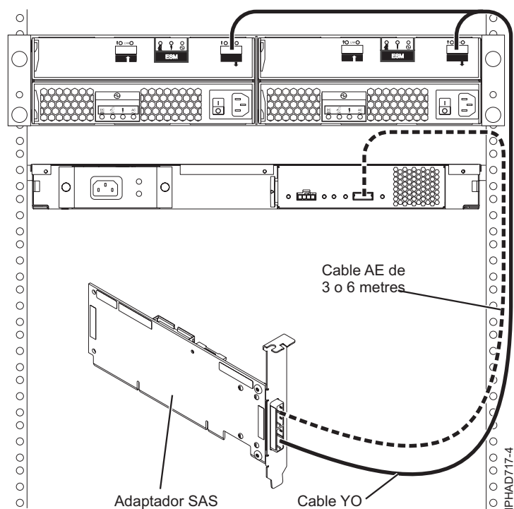
Figura 150. Un adaptador SAS a un calaix d'expansió de discs i a un calaix d'expansió de mitjans
