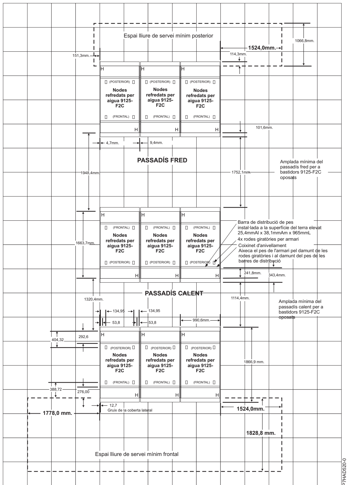
Figura 2. Espai lliure per al servei tècnic per a diversos bastidors - Passadís calent i passadís fred
