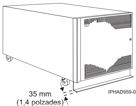
Figura 20. Model 0554 i 7014-S11 amb barra estabilitzadora
