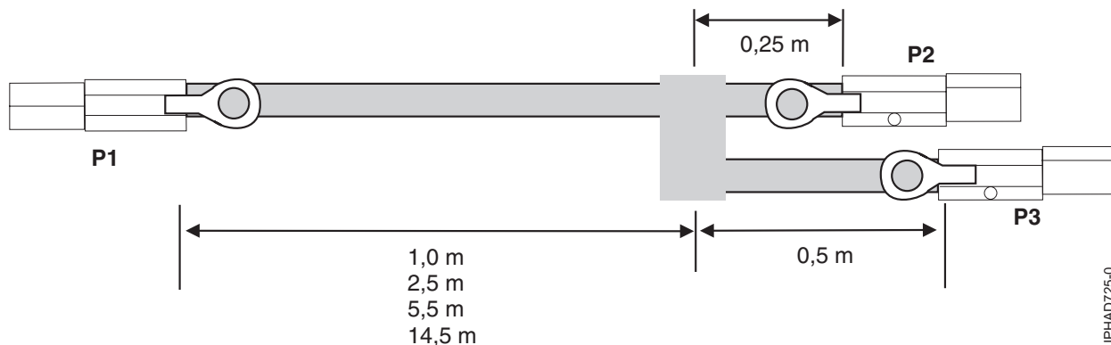
Figura 143. Longituds de cables de conjunt de cable YO SAS extern
