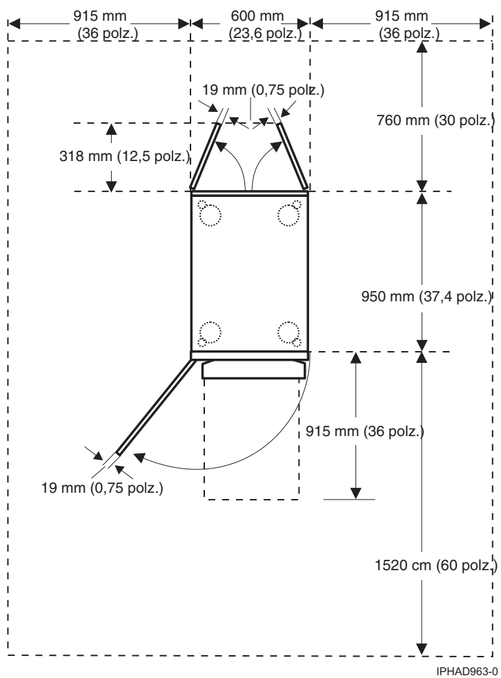
Figura 24. Vista del pla del model 0555 i 7014-S25
