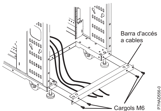
Figura 30. Barra d'accés als cables
