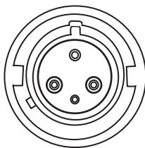
Figura 53. Tipus de receptacle IEC 60309 2P+E
