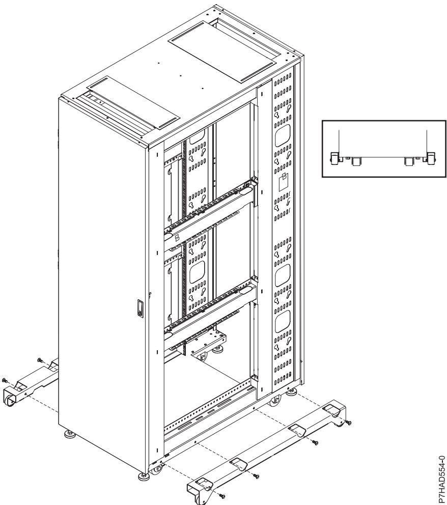
Figura 28. Ubicacions dels estabilitzadors
