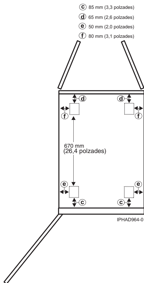
Figura 21. Ubicacions de les rodes giratòries del model 0555 i 7014-S25
