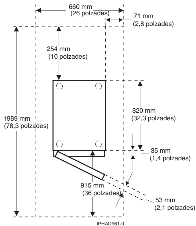
Figura 17. Vista del pla del model 0554 i 7014-S11
