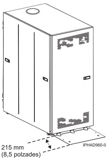
Figura 19. Model 0555 i 7014-S25 amb peu estabilitzador
