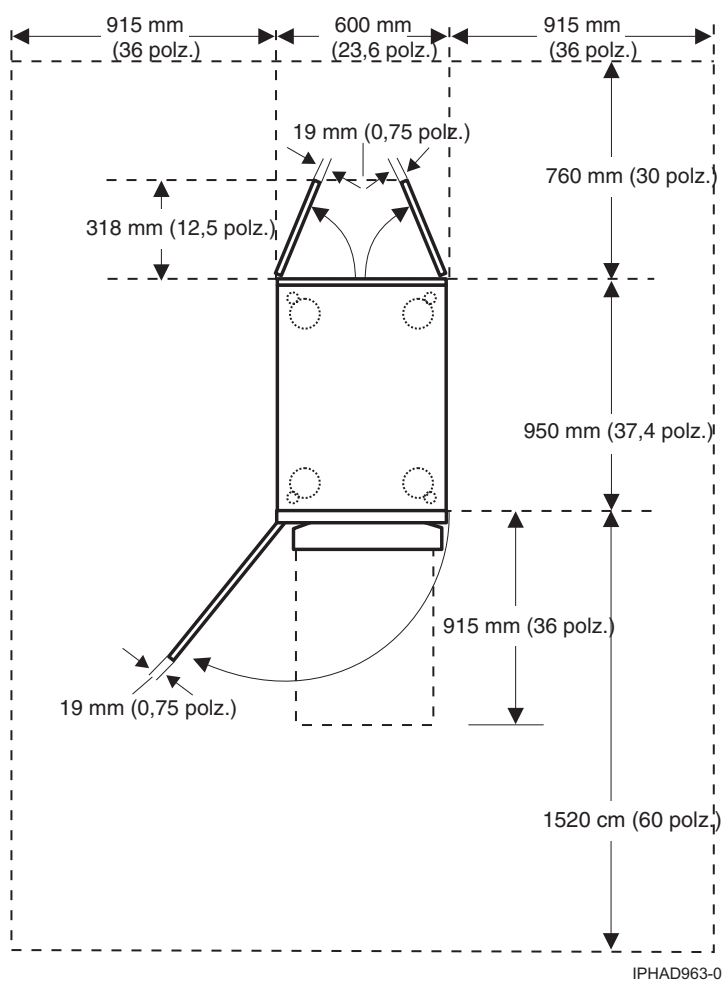
Figura 20. Vista del pla del model 0555 i 7014-S25
