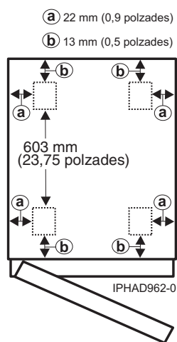
Figura 18. Ubicacions de les rodes giratòries del model 0554 i 7014-S11
