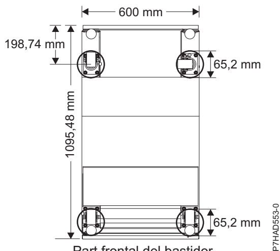
Figura 24. Ubicació de les rodes giratòries
