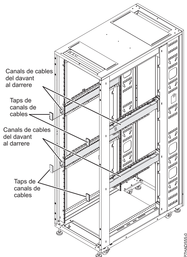
Figura 25. Connexió dels cables al bastidor
