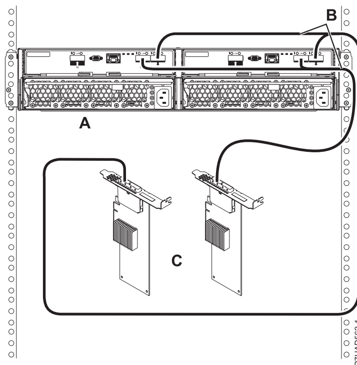
Figura 161. Connexió de mode 1 d'un calaix 5887 utilitzant cables YO a adaptadors SAS duals
