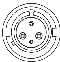
Figura 34. Tipus de receptacle IEC 60309 P+N+E
