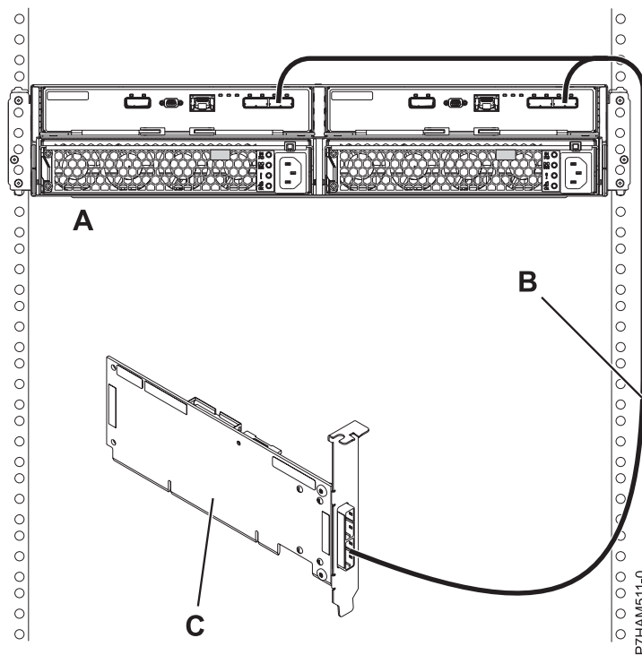
Figura 160. Connexió de mode 1 d'un calaix 5887 utilitzant un cable YO a un adaptador SAS únic
