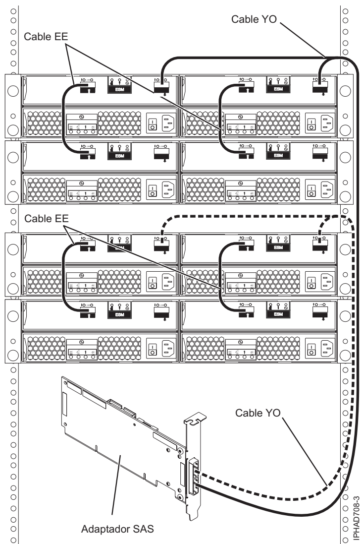
Figura 143. Un adaptador SAS a quatre calaixos d'expansió de discs
