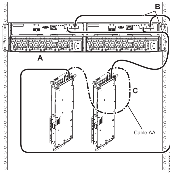
Figura 168. Connexió de mode 1 d'un calaix 5887 utilitzant cables YO a adaptadors SAS duals
