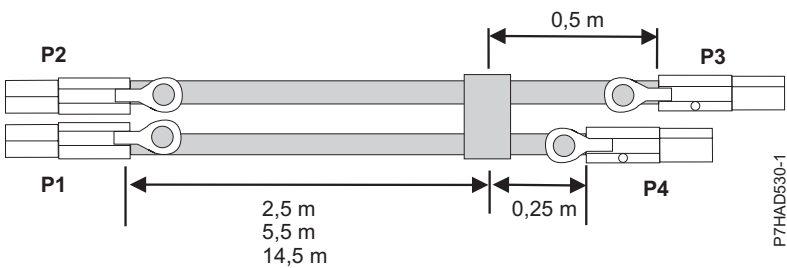
Figura 138. Longituds de cables de conjunt de cable X SAS extern
