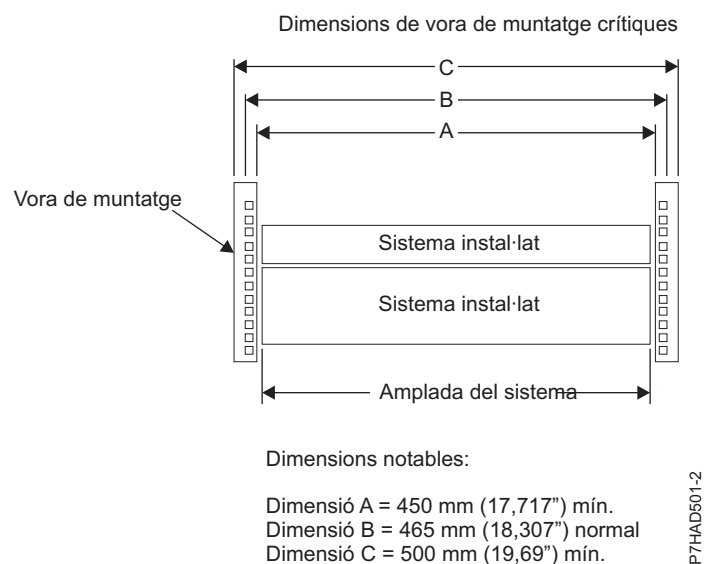
Figura 175. Dimensions de les vores de muntatge de gravetat
