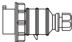
Figura 31. Tipus d'endoll IEC 60309 3P+N+E
