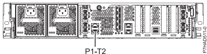
Figura 132. Vista posterior dels models 8231-E2B, 8231-E1C, 8231-E1D, 8231-E2C, 8231-E2D i 8268-E1D amb la ubicació d'instal·lació dels cables
