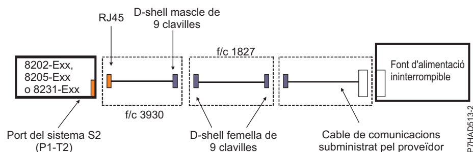
Figura 134. Cables de la font d'alimentació ininterrompible per als models 8202-E4B, 8202-E4C, 8205-E6B, 8205-E6C, 8231-E2B, 8231-E1C, 8231-E1D, 8231-E2C, 8231-E2D i 8268-E1D
