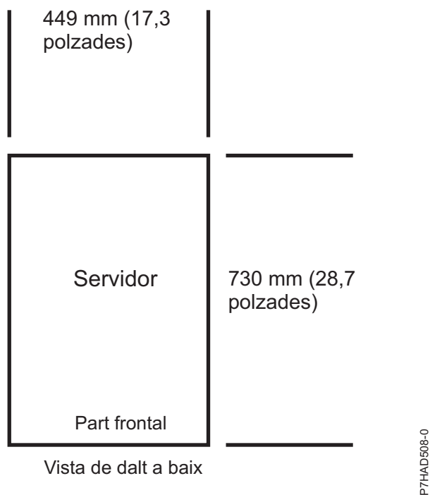
Figura 1. Vista de planta del model 8202-E4B, 8202-E4C, 8202-E4D, 8205-E6B, 8205-E6C i 8205-E6D (servidors muntats en bastidor)
