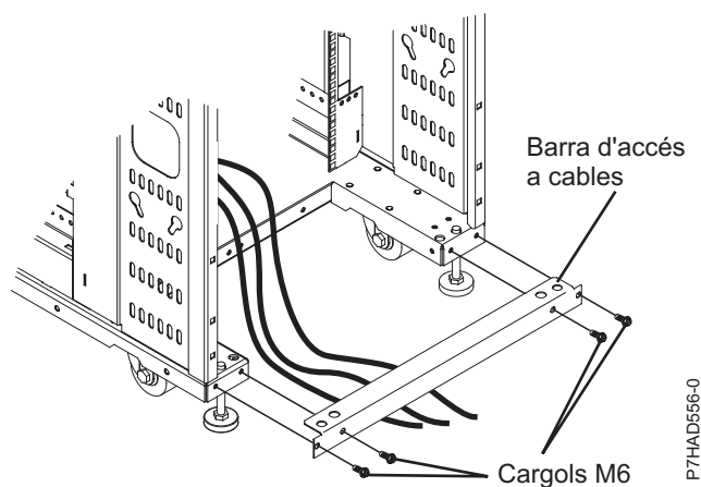
Figura 14. Barra d'accés als cables
