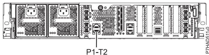
Figura 114. , 8246-L1C, 8246-L1D, 8246-L1S, 8246-L1T, 8246-L2C, 8246-L2D, 8246-L2S i 8246-L2T amb la ubicació d'instal·lació dels cables
