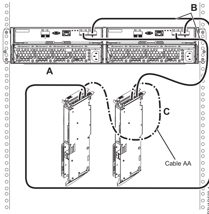
Figura 149. Connexió de mode 1 d'un calaix 5887 utilitzant cables YO a adaptadors SAS duals
