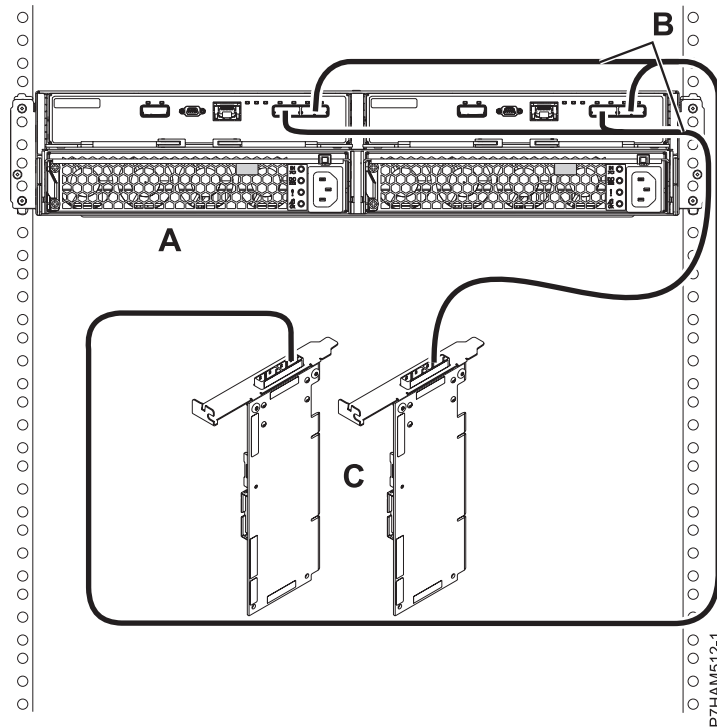
Figura 146. Connexió de mode 1 d'un calaix 5887 utilitzant cables YO a adaptadors SAS duals
