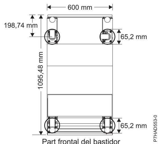
Figura 12. Ubicació de les rodes giratòries
