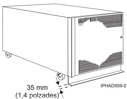
Figura 4. Model 0554 i 7014-S11 amb barra estabilitzadora
