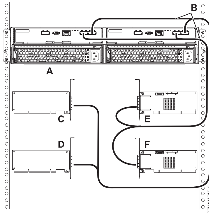
Figura 145. Connexió de mode 4 d'un calaix 5887 utilitzant cables X a quatre adaptadors SAS únics
