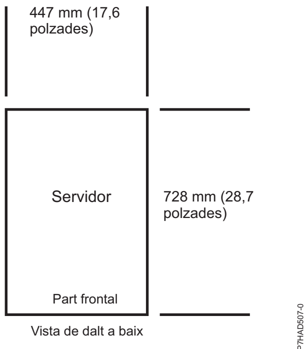
Figura 1. Vista de planta per als models 8246-L1C, 8246-L1D, 8246-L1S, 8246-L1T, 8246-L2C, 8246-L2D, 8246-L2S i 8246-L2T (servidor muntat en bastidor)
