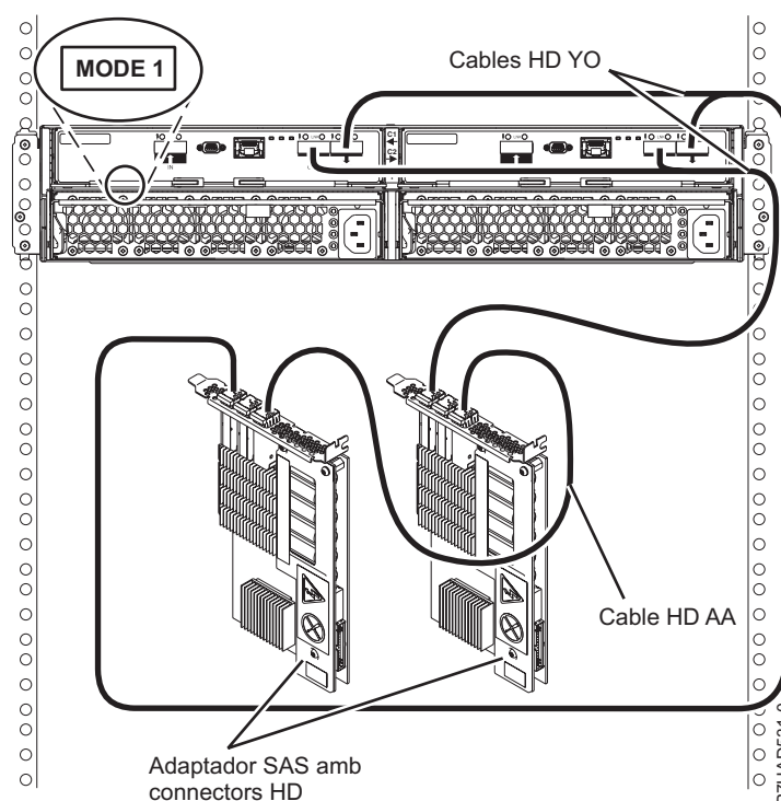
Figura 150. Connexió de mode 1 d'un calaix 5887 a dos adaptadors SAS amb connectors HD
