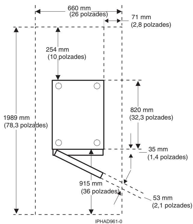
Figura 5. Vista del pla del model 0554 i 7014-S11
