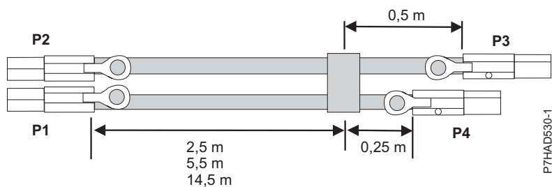
Figura 119. Longituds de cables de conjunt de cable X SAS extern
