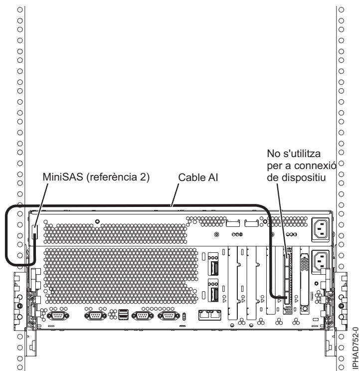
Figura 130. Adaptador FC5904 o FC5908 connectat a calaixos d'expansió de discs
