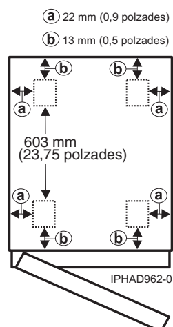
Figura 6. Ubicacions de les rodes giratòries del model 0554 i 7014-S11
