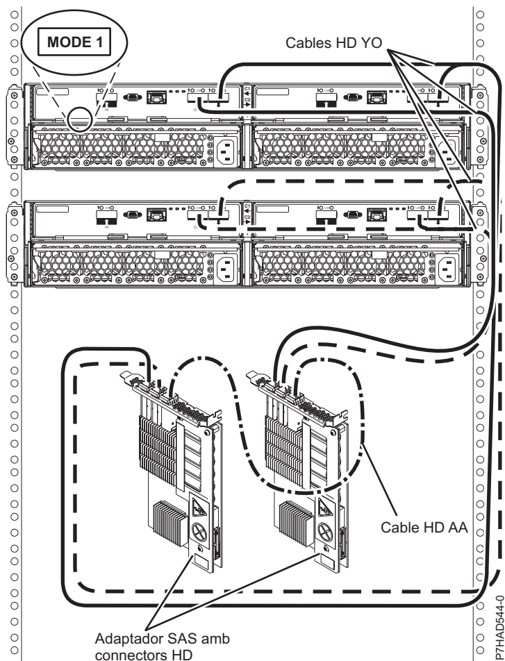
Figura 151. Connexió de mode 1 de dos calaixos 5887 utilitzant connectors HD a dos adaptadors SAS
