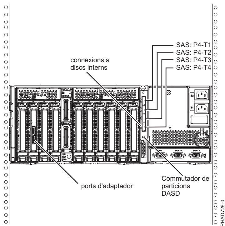
Figura 140. Dos adaptadors SAS RAID a un calaix d'expansió de discs en una configuració HA JBOD
