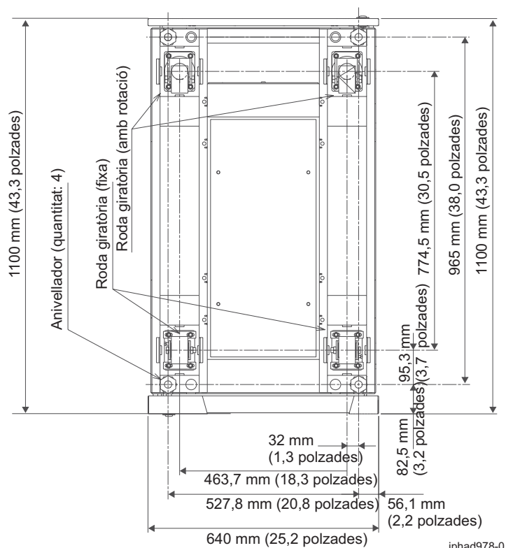
Figura 3. Ubicacions de rodes giratòries i anivelladors
