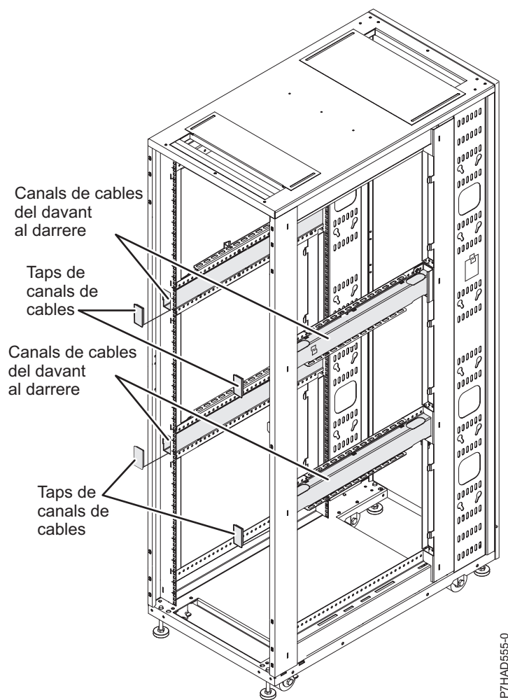
Figura 13. Connexió dels cables al bastidor
