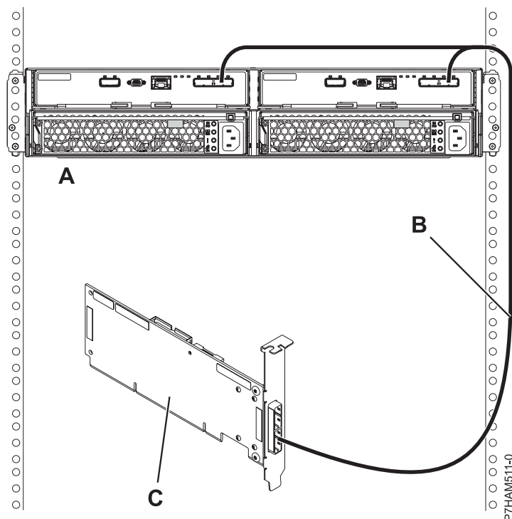
Figura 141. Connexió de mode 1 d'un calaix 5887 utilitzant un cable YO a un adaptador SAS únic
