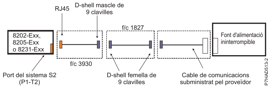
Figura 115. Cables de la font d'alimentació ininterrompible per als models 8246-L1C, 8246-L1S, 8246-L2C i 8246-L2S
