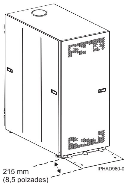
Figura 7. Model 0555 i 7014-S25 amb peu estabilitzador
