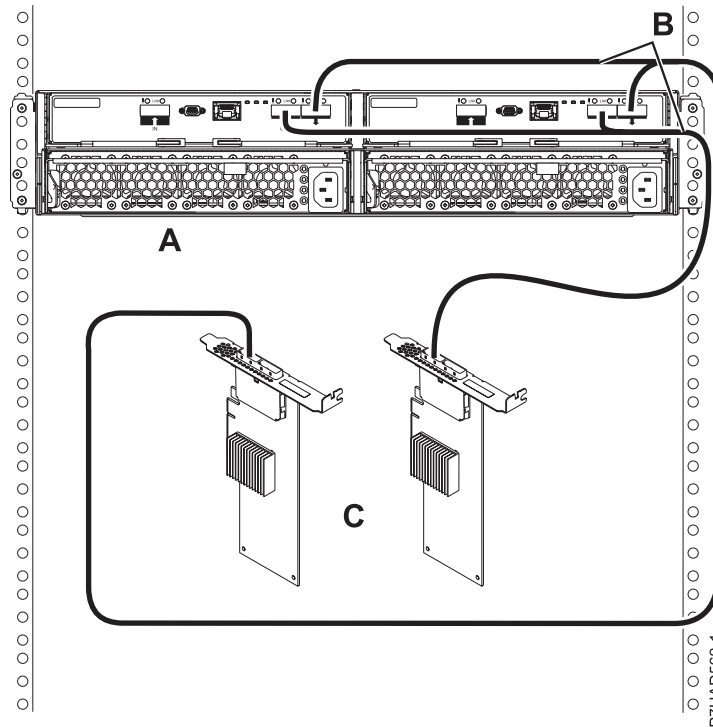
Figura 142. Connexió de mode 1 d'un calaix 5887 utilitzant cables YO a adaptadors SAS duals
