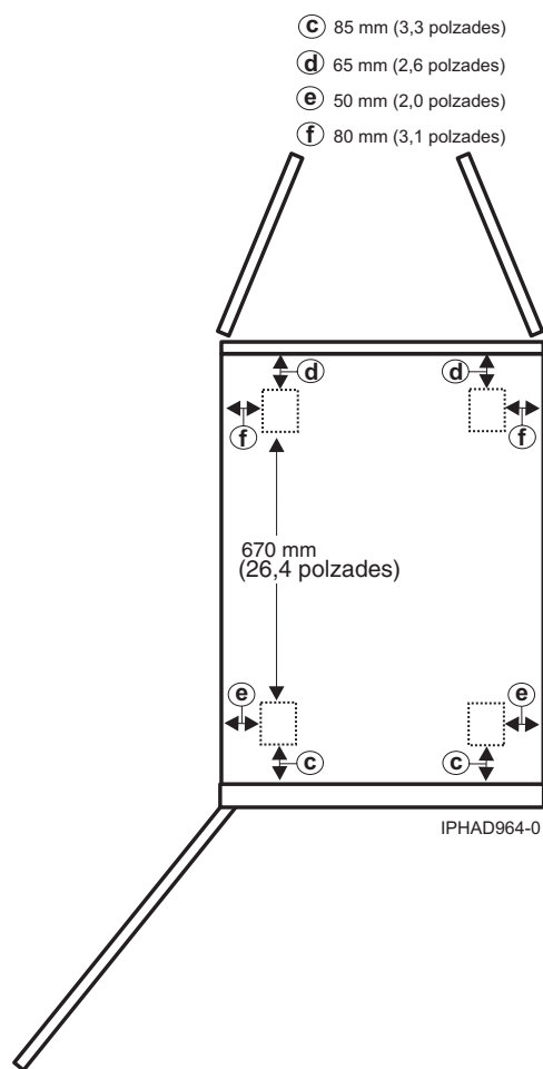
Figura 21. Ubicacions de les rodes giratòries del model 0555 i 7014-S25
