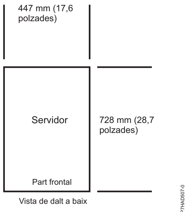
Figura 1. Vista de planta per als models 8231-E2B, 8231-E1C, 8231-E1D, 8231-E2C, 8231-E2D i 8268-E1D (servidor muntat en bastidor)
