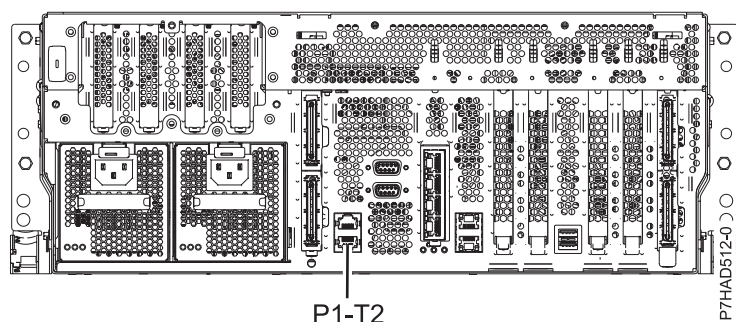
Figura 133. Vista posterior del model 8202-E4B, 8202-E4C, 8202-E4D, 8205-E6B, 8205-E6C i 8205-E6D amb la ubicació d'instal·lació dels cables
