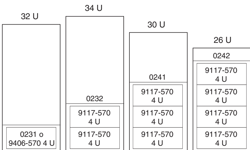
Figura 8. 570 en bastidor
