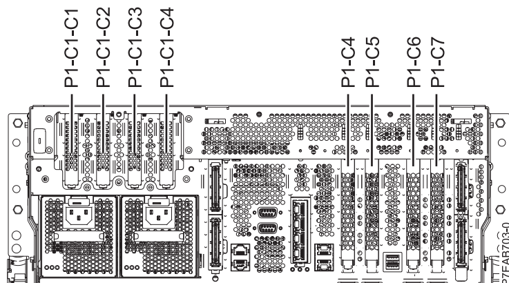
Figura 1. Vista posterior del sistemes 8202-E4B i 8205-E6B amb els codis d'ubicació de les ranures PCI
