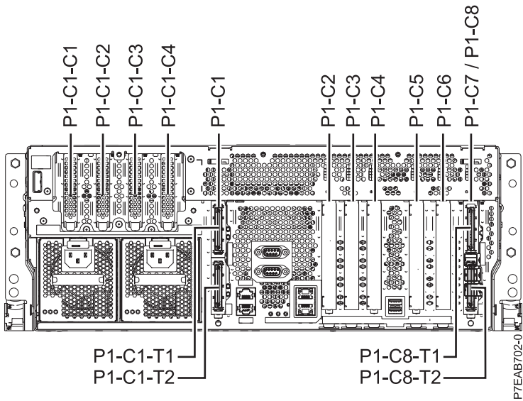
Figura 4. Vista posterior del sistema que mostra les ranures PCI amb els seus codis d'ubicació
