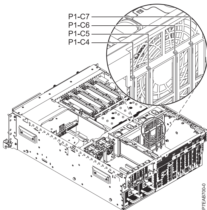
Figura 2. Codis d'ubicació de ranures PCI als sistemes 8202-E4B i 8205-E6B
