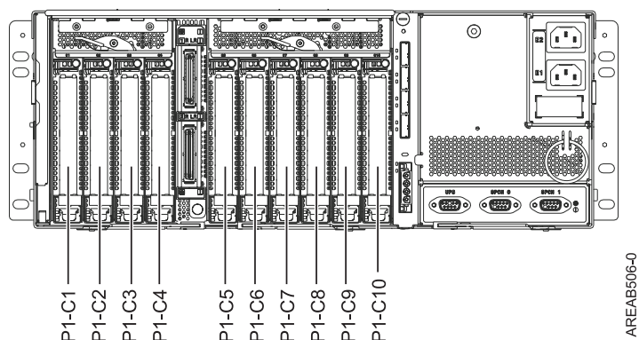
Figura 6. Vista posterior. Aquesta figura mostra la vista posterior de la unitat d'expansió.
