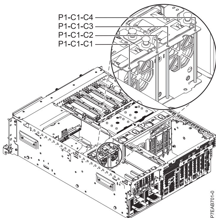
Figura 3. Expansió de l'elevador PCI amb els codis d'ubicació als sistemes 8202-E4B i 8205-E6B
