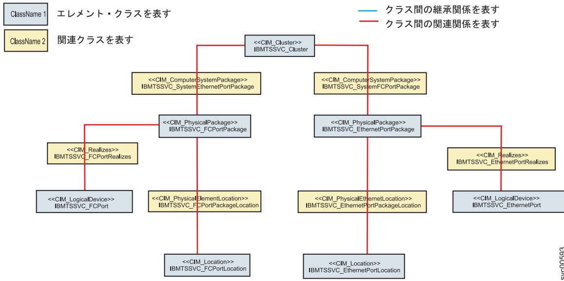
図 19. ロケーションと物理パッケージ間の関係の概要
