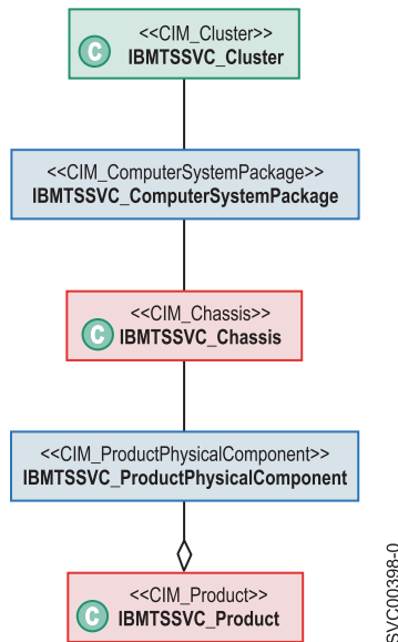
図 23. SAN ボリューム・コントローラー用 CIM エージェントの物理パッケージの概要
