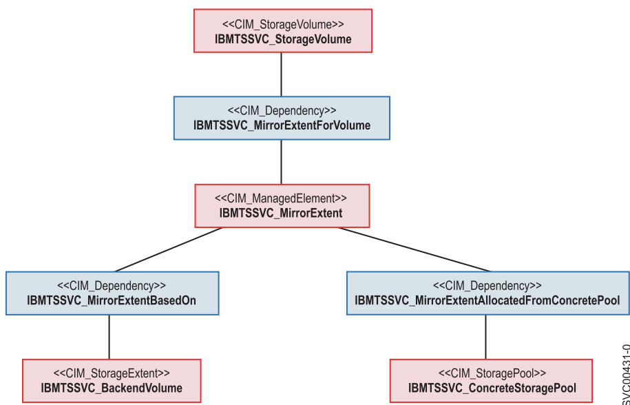
図 26. ミラーリングしたストレージ・ボリュームにおけるクラスと関連付け
