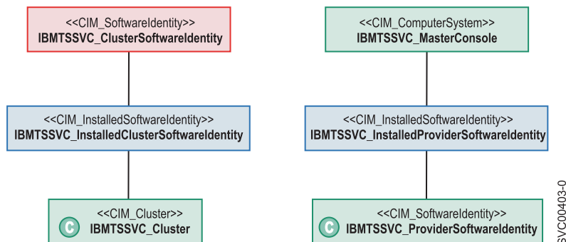
図 25. ソフトウェア・インスタンスのクラス・ダイアグラム
