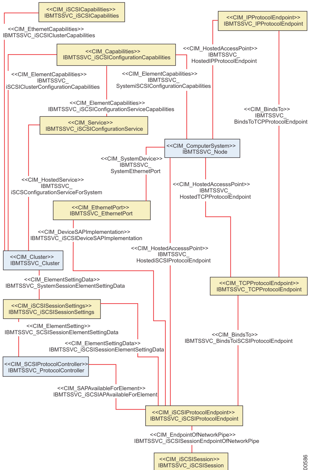
図 17. ターゲット装置の iSCSI 固有の面の概要
