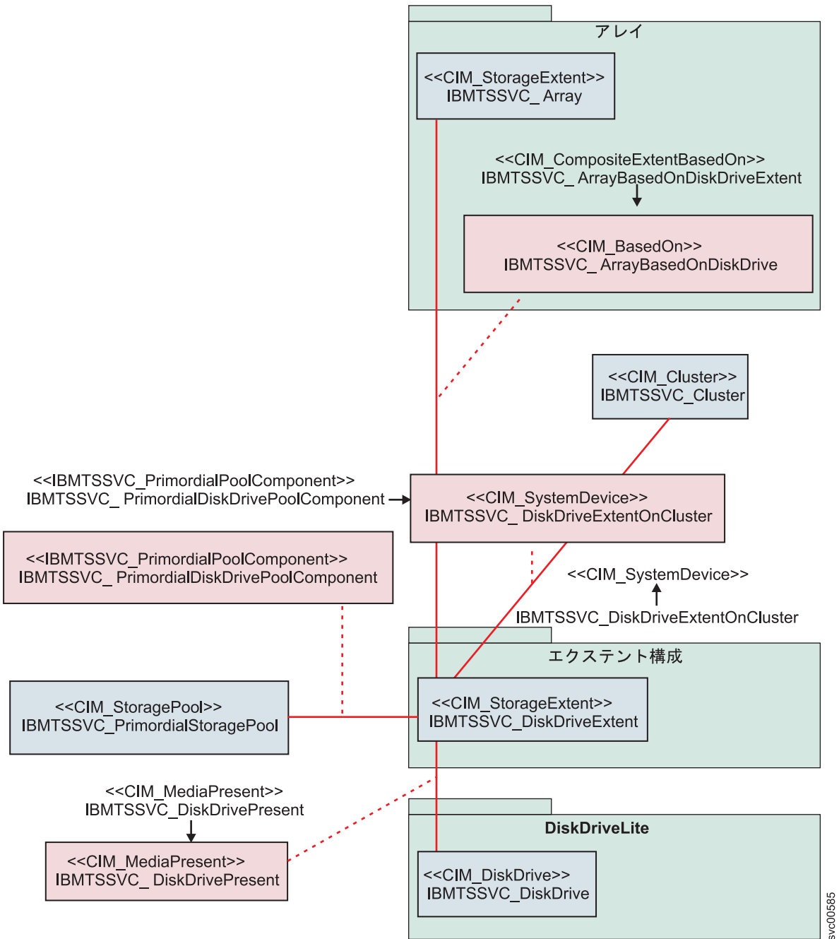
図 14. エクステント構成サブプロファイル
