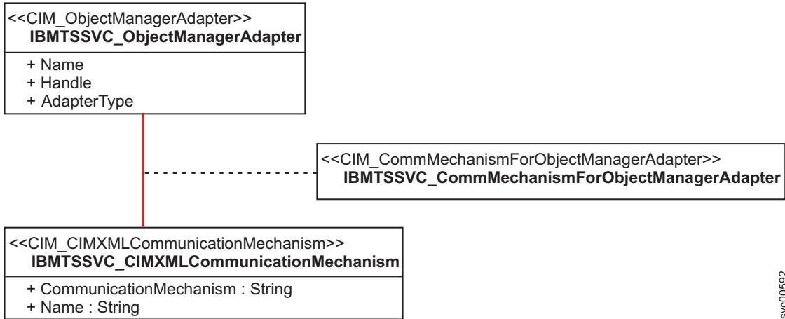
図 22. オブジェクト・マネージャー・アダプター・プロファイルの統一モデリング言語エレメントの概要
