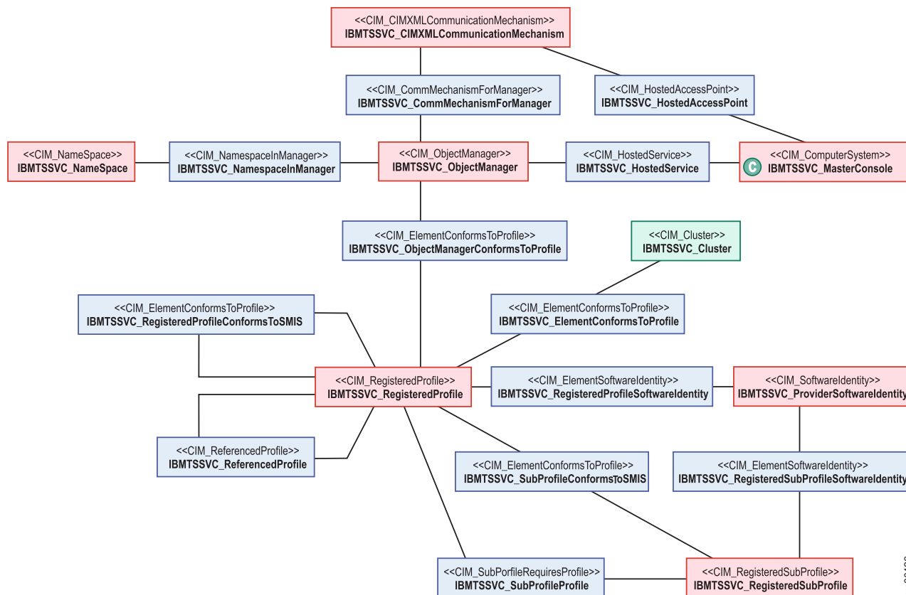
図 24. SAN ボリューム・コントローラー用 CIM エージェントのサーバー・プロファイルの概要
