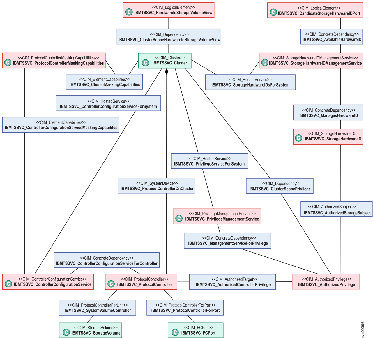
図 20. マスキングおよびマッピング・インスタンスのクラス・ダイアグラム
