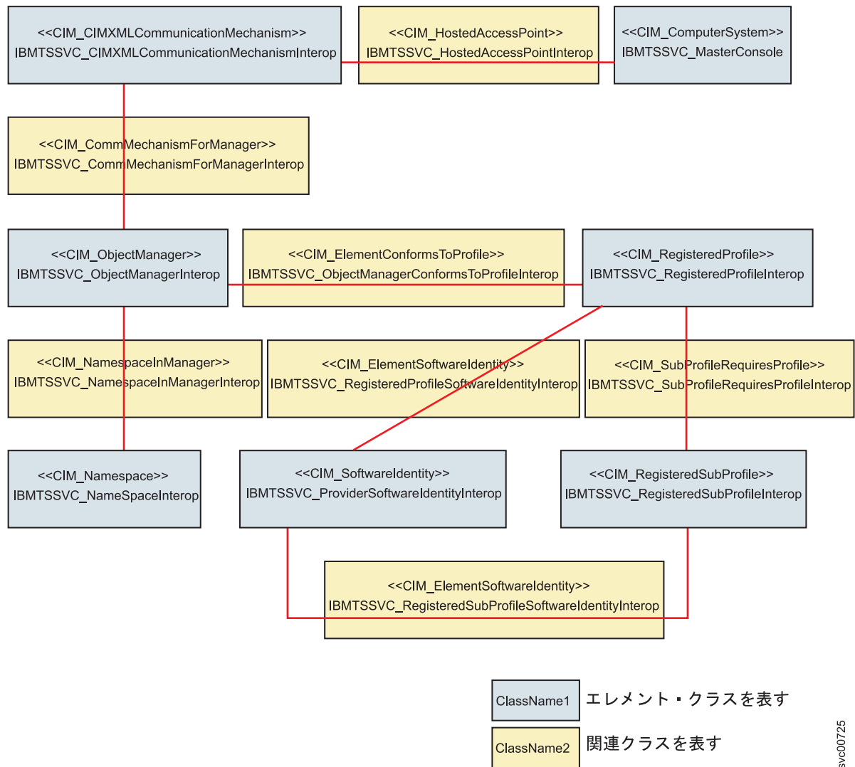
図 16. interop インスタンスのクラス・ダイアグラム
