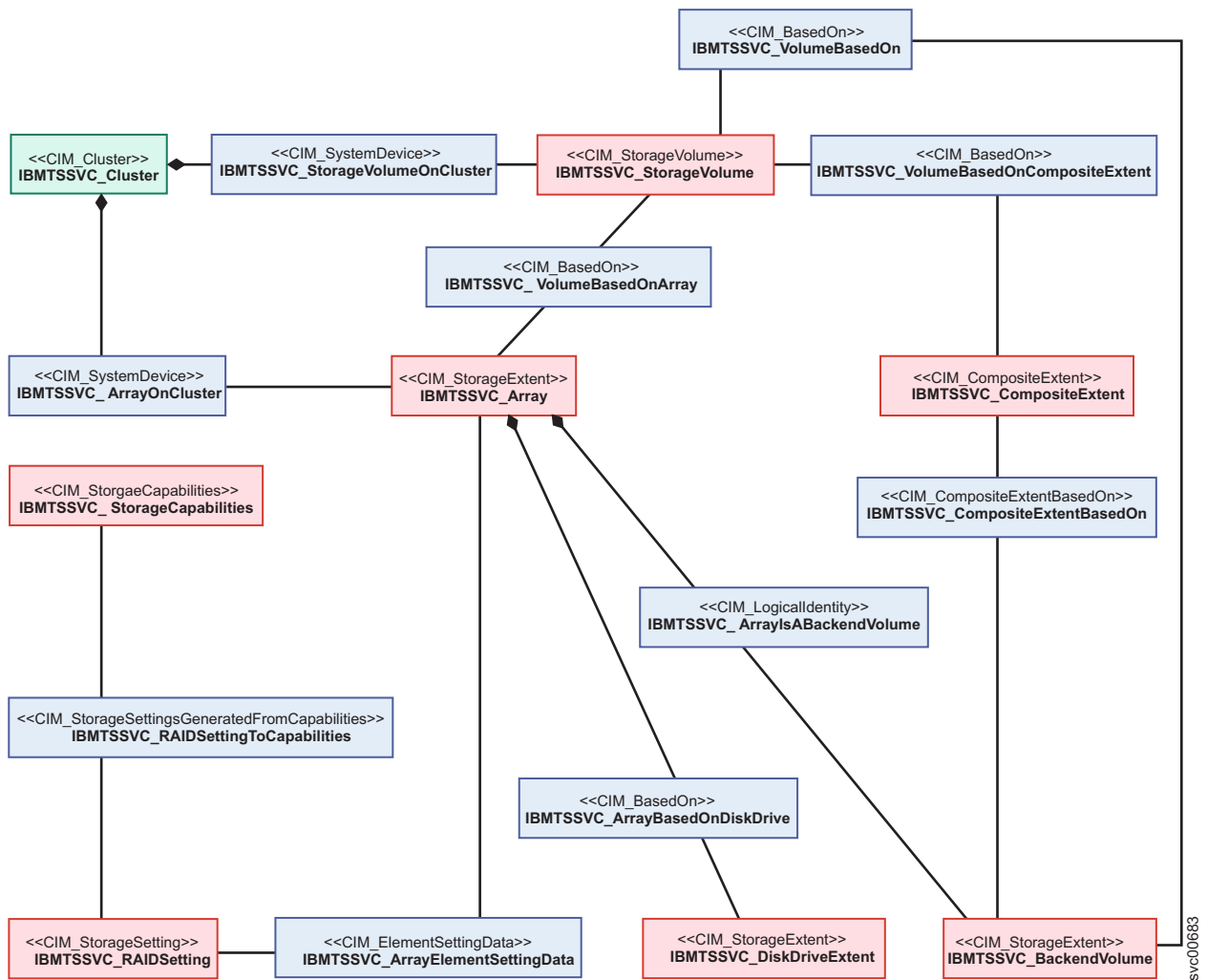
図 7. ブロック・サービスに対する RAID サポート
