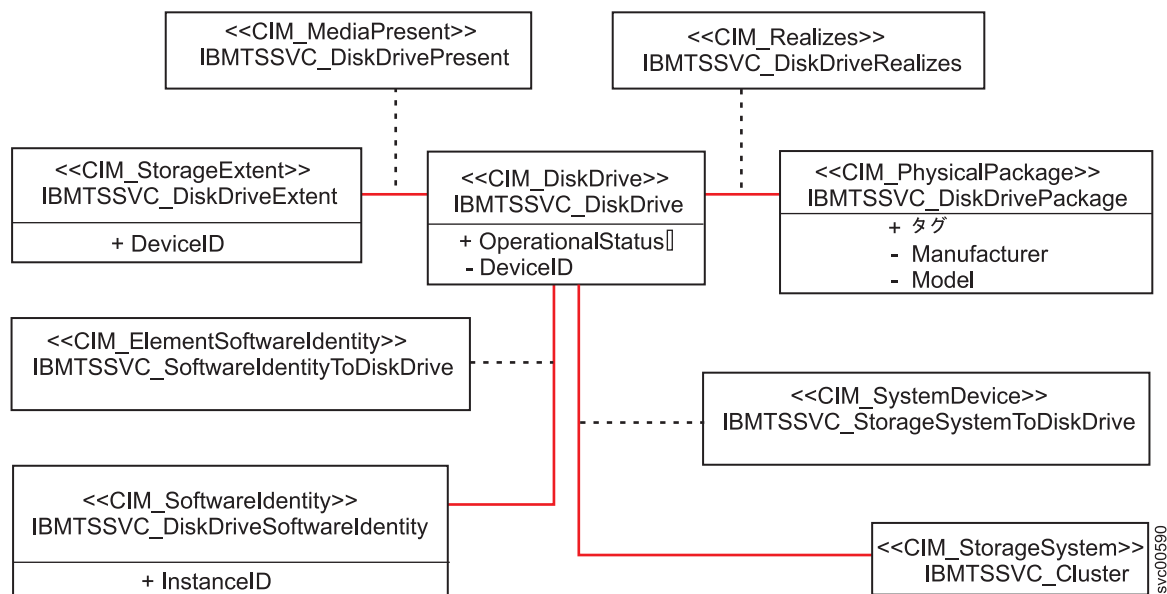
図 10. ディスク・ドライブ・ライト・プロファイルの統一モデリング言語エレメントの概要
