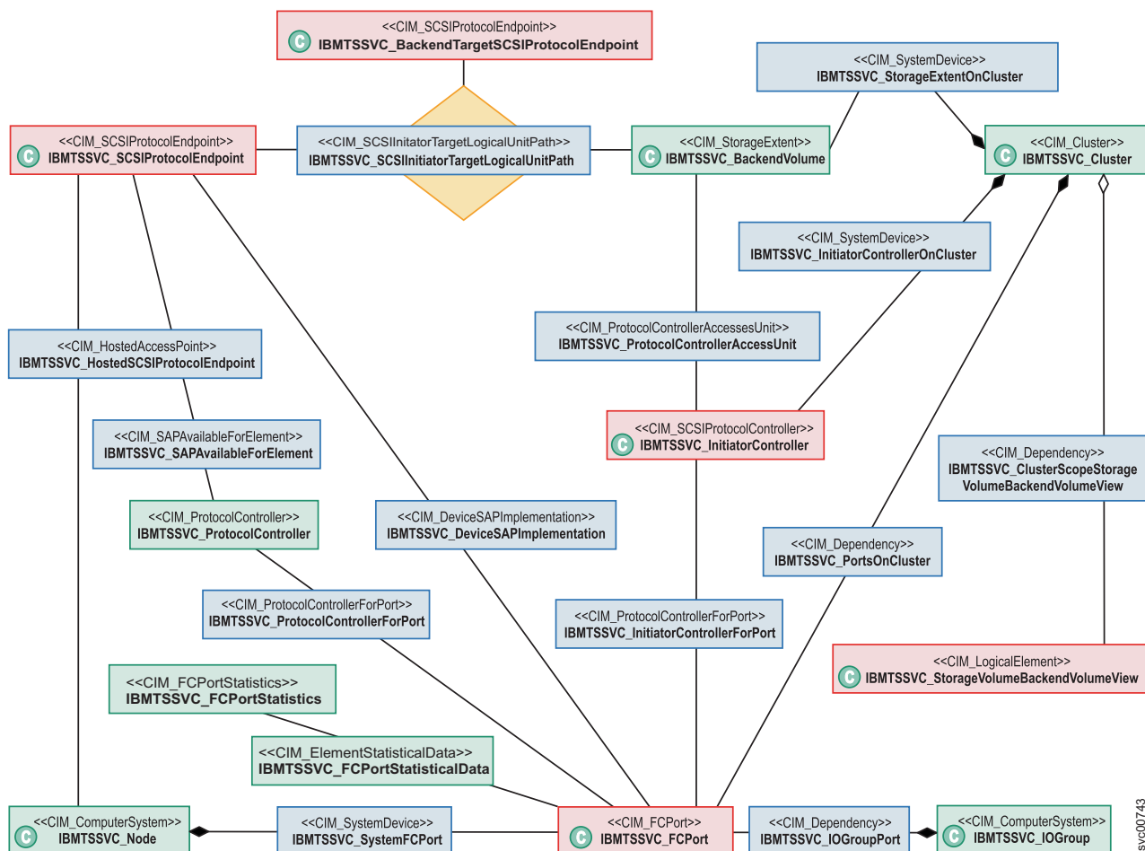
図 15. FC ポート・インスタンスのクラス・ダイアグラム
