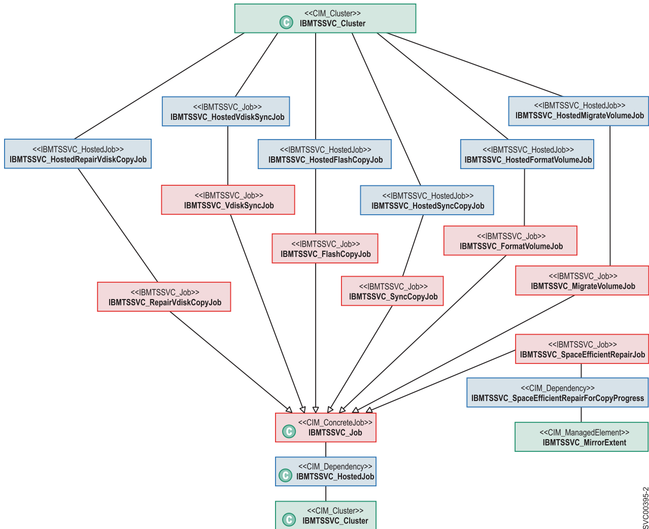
図 18. ジョブ制御インスタンスのクラス・ダイアグラム
