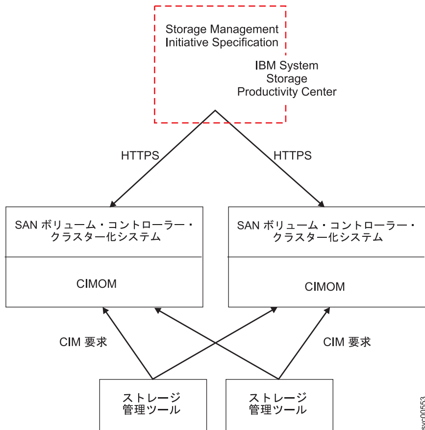
図2. クラスター化システム上の CIMOM
