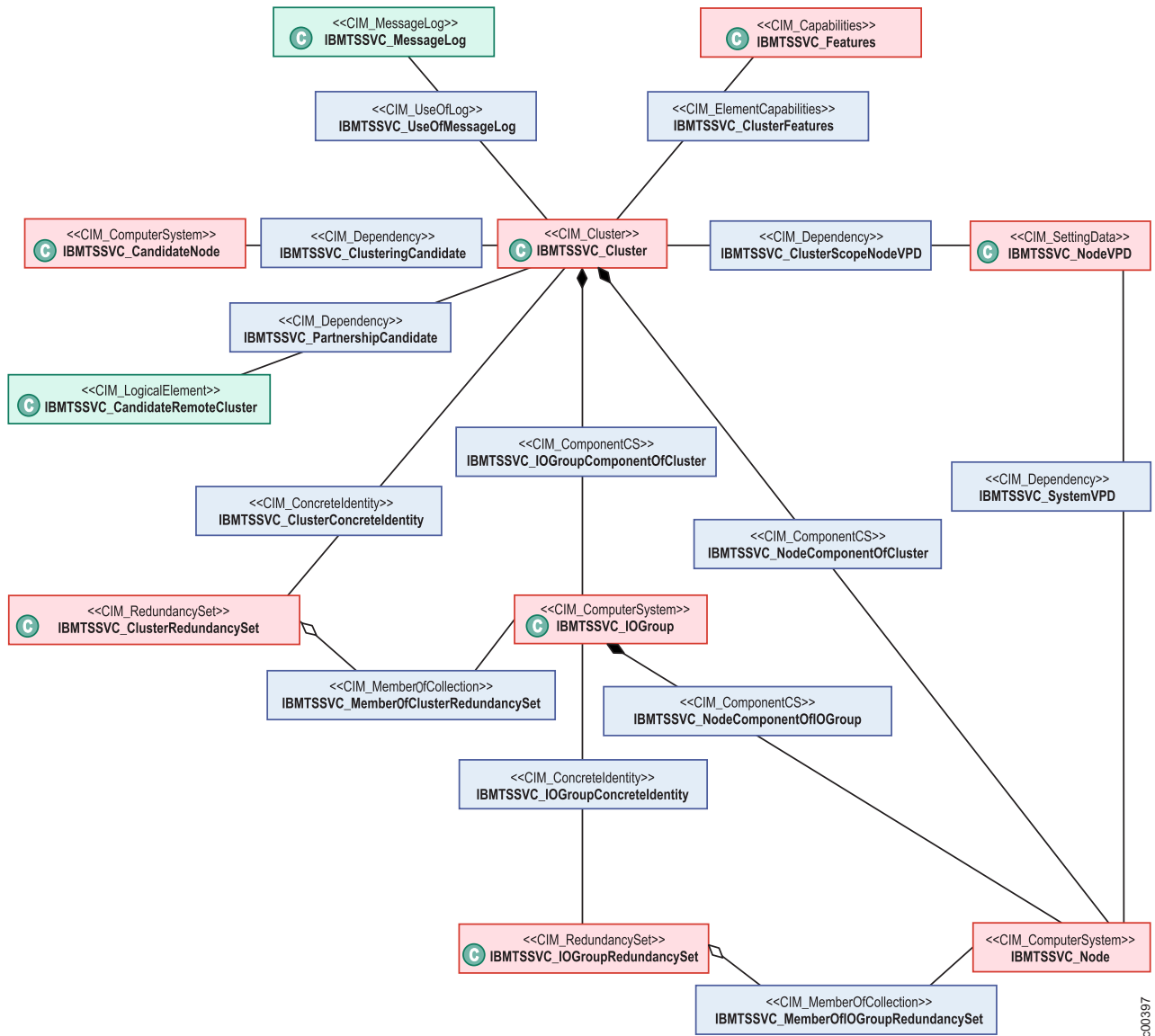
図 21. 複数コンピューター・システム・インスタンスのクラス・ダイアグラム
