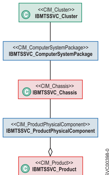
図 24. Storwize V7000用 CIM エージェントの物理パッケージの概要
