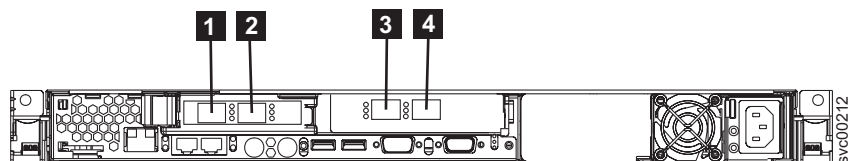
図 15. SAN ボリューム・コントローラー 2145-8F2 の物理ポート番号
