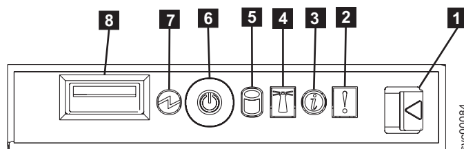
図 2. SAN ボリューム・コントローラー 2145-8F2 および SAN ボリューム・コントローラー 2145-8F4 オペレーター情報パネル
