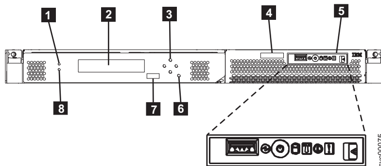
図1. SAN ボリューム・コントローラー 2145-8F2 および SAN ボリューム・コントローラー 2145-8F4 フロント・パネル・アセンブリ
