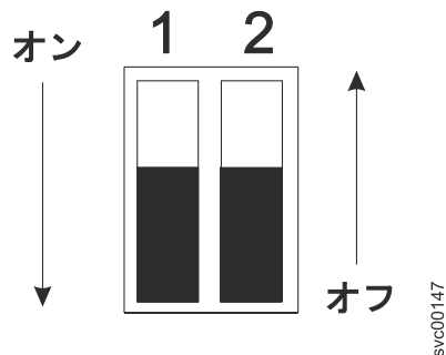
図 19. 2145 UPS-1U ディップ・スイッチ
