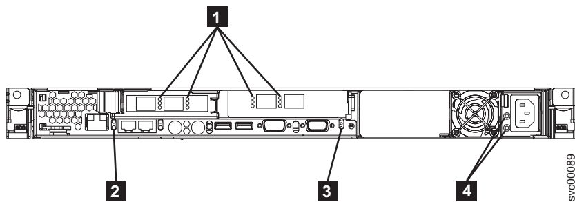
図4. SAN ボリューム・コントローラー 2145-8F2 背面パネルのインディケータ
