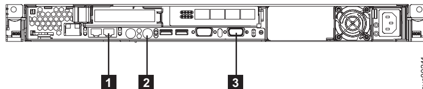
図 9. SAN ボリューム・コントローラー 2145-8F4 のサービス・ポート
