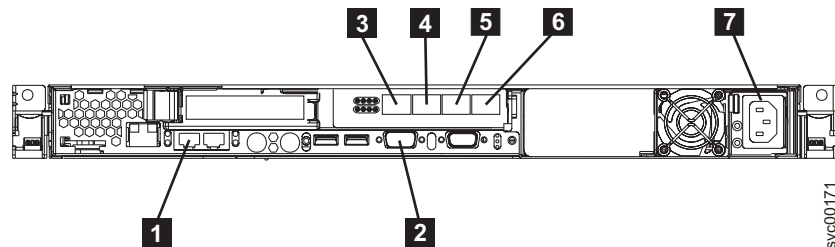
図7. SAN ボリューム・コントローラー 2145-8F4 外部コネクタ
