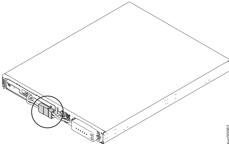
図 33. 2145 UPS-1U 内部バッテリー・コネクタ
