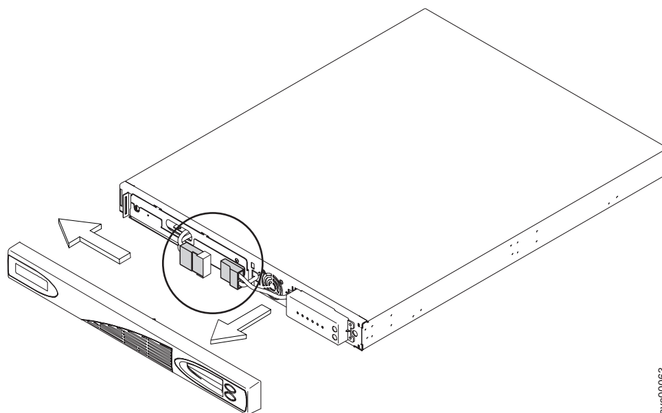
図 31. 2145 UPS-IUのフロント・パネルの取り外し
