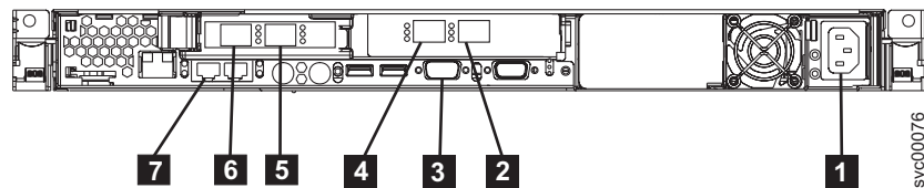
図 12. SAN ボリューム・コントローラー 2145-8F2 外部コネクター
