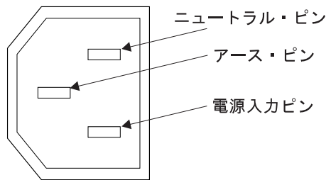
図 8. 電源コネクター
