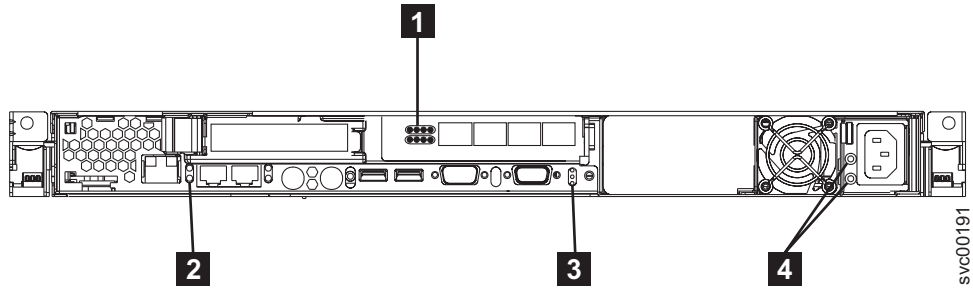
図3. SAN ボリューム・コントローラー 2145-8F4 背面パネルのインディケータ
