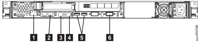
図 10. SAN ボリューム・コントローラー 2145-8F4 の通常の操作では使用されないポート
