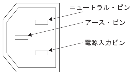
図 13. 電源コネクター
