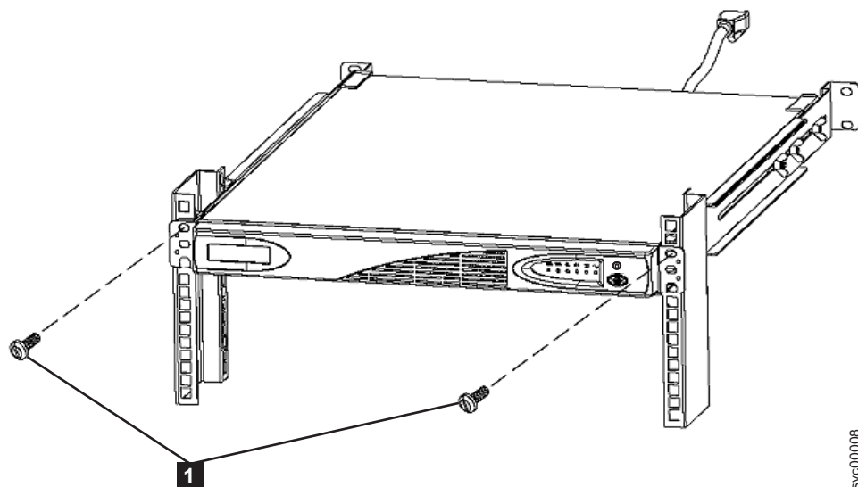
図 30. 2145 UPS-IU用のねじの取り付け
