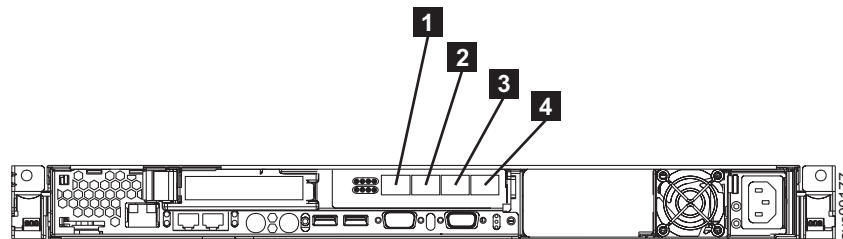
図 14. SAN ボリューム・コントローラー 2145-8F4 の物理ポート番号
