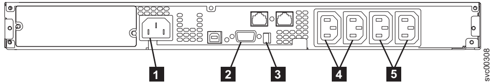
図 18. 2145 UPS-1Uのコネクターおよびスイッチ
