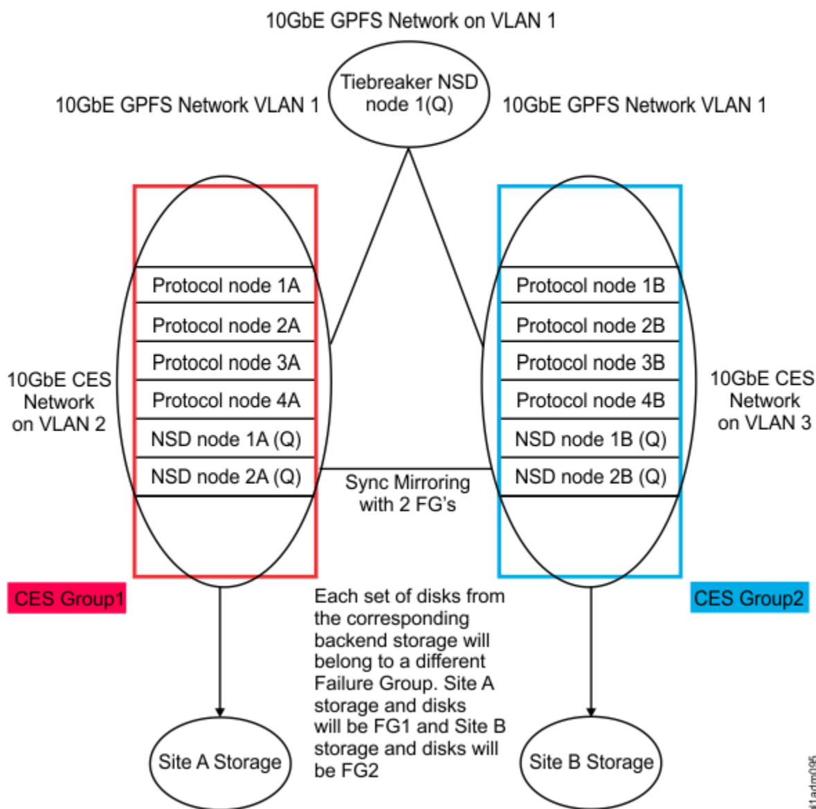
Figure 37. Local Site CES Group
