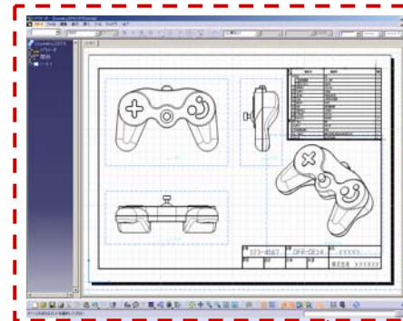
改訂前図面
