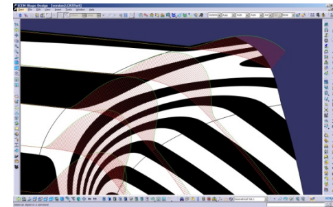
G3: 捩率(曲率変化率)連続
