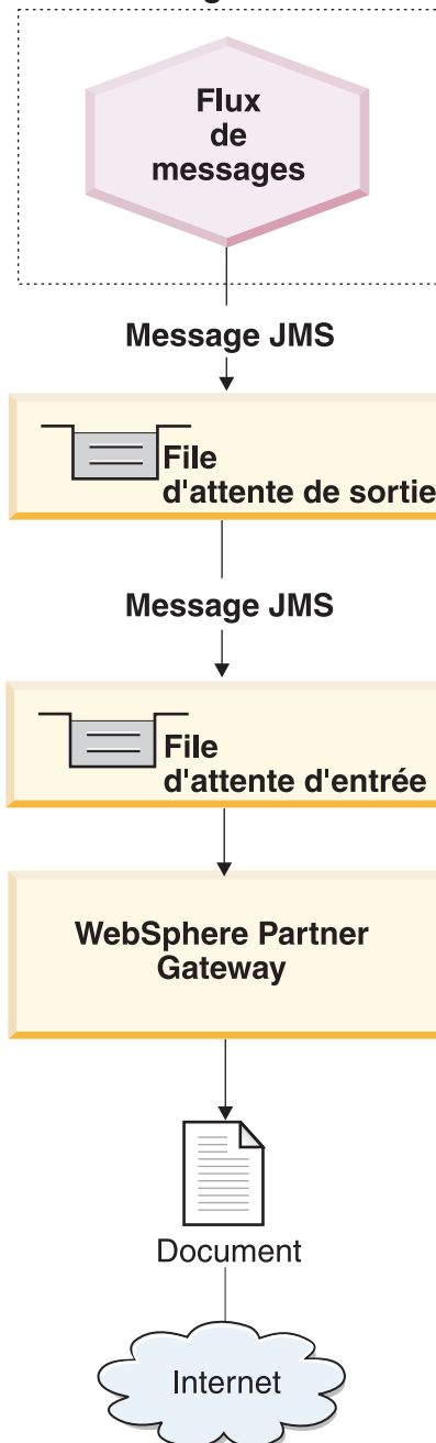
Figure 39. Flux de messages entre un flux de messages et WebSphere Partner Gateway via le protocole de transport JMS
