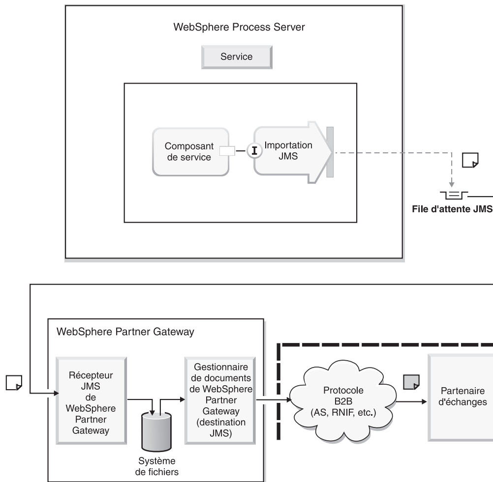
Figure 24. Importation JMS de réception de documents via JMS
