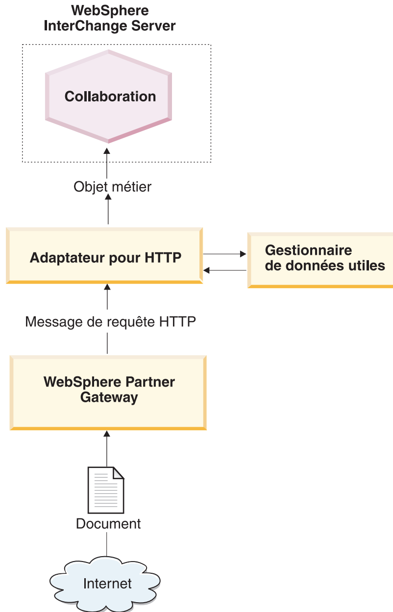
Figure 31. Flux de messages entre WebSphere Partner Gateway et une collaboration via HTTP
