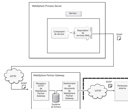
Figure 2. Récepteurs du partenaire interne et des partenaires externes
