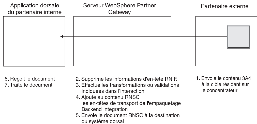
Figure 4. Comment circule un document jusqu'au système dorsal
