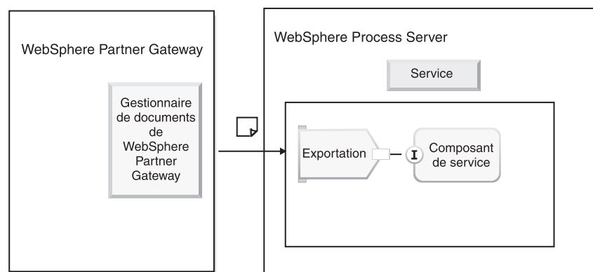
Figure 16. Utilisation de la liaison d'exportation par WebSphere Partner Gateway pour l'envoi de documents à WebSphere Process Server
