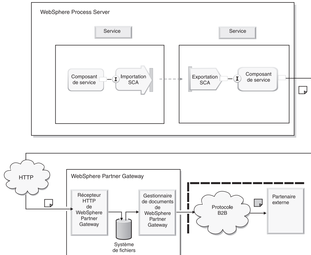
Figure 22. Fonctionnement de l'envoi d'un message de WebSphere Process Server au récepteur HTTP de WebSphere Partner Gateway
