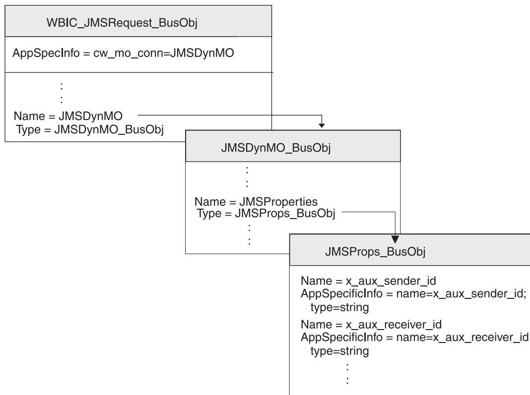
Figure 37. Relation entre l'objet métier de type demande et le méta-objet dynamique JMS
