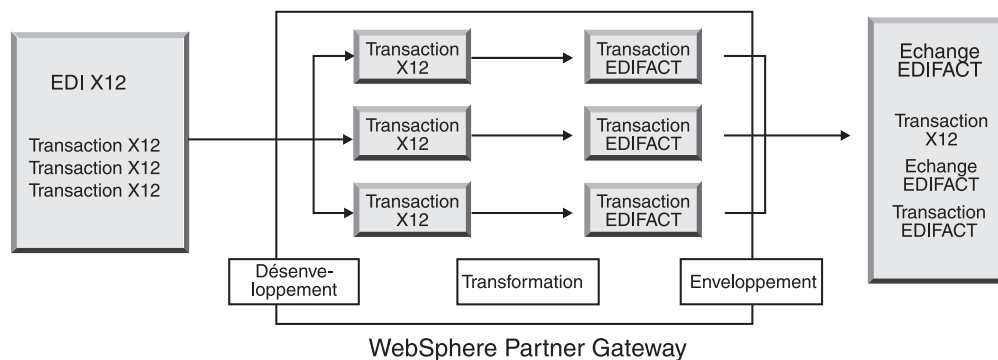
Figure 6. Echange EDI de l'application dorsale au partenaire
