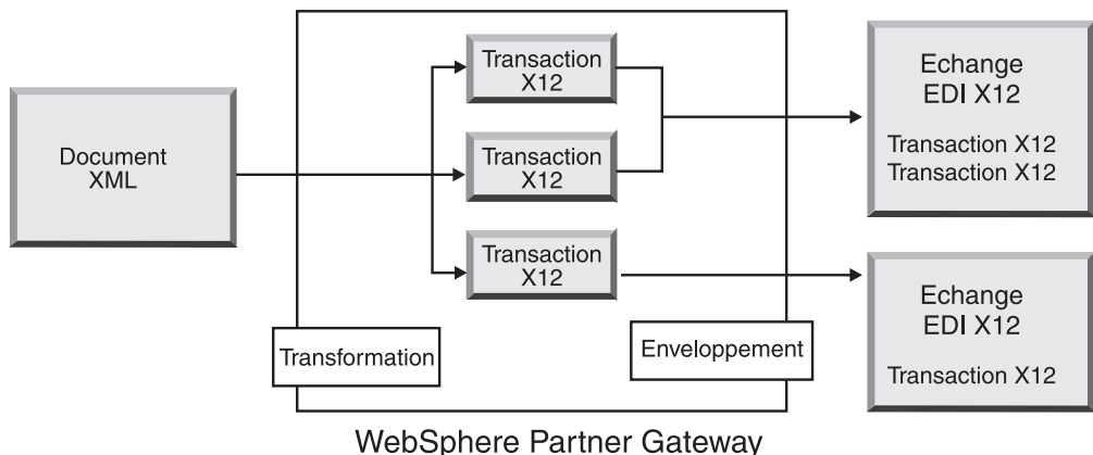
Figure 9. Document XML envoyé de l'application dorsale au partenaire (sous forme d'échange EDI)
