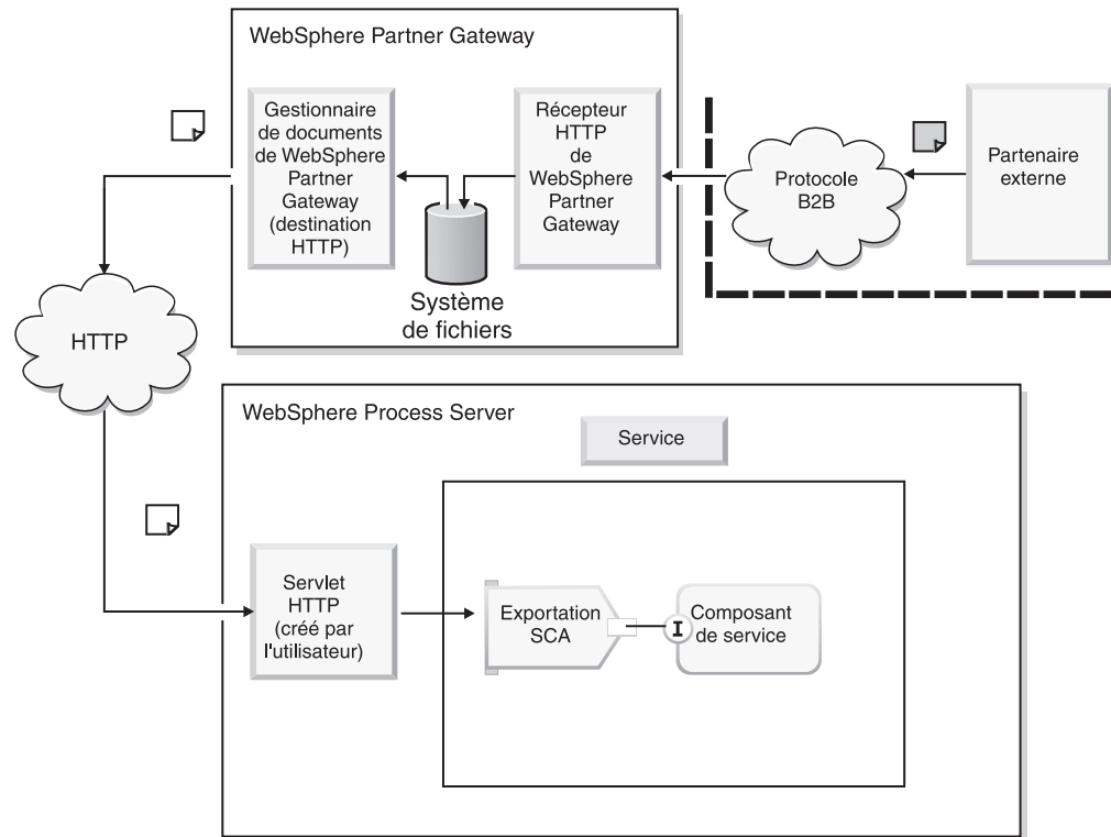
Figure 21. Fonctionnement de l'envoi d'un message de WebSphere Partner Gateway au servlet HTTP
