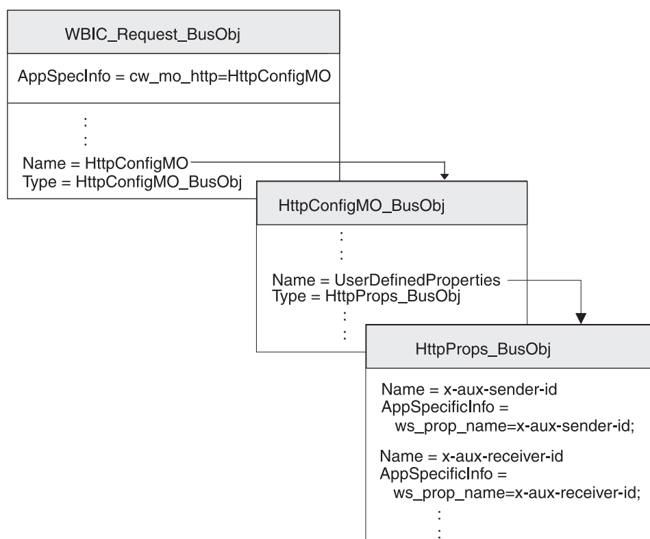
Figure 34. Relation entre l'objet métier de type demande et le méta-objet de configuration de protocole HTTP
