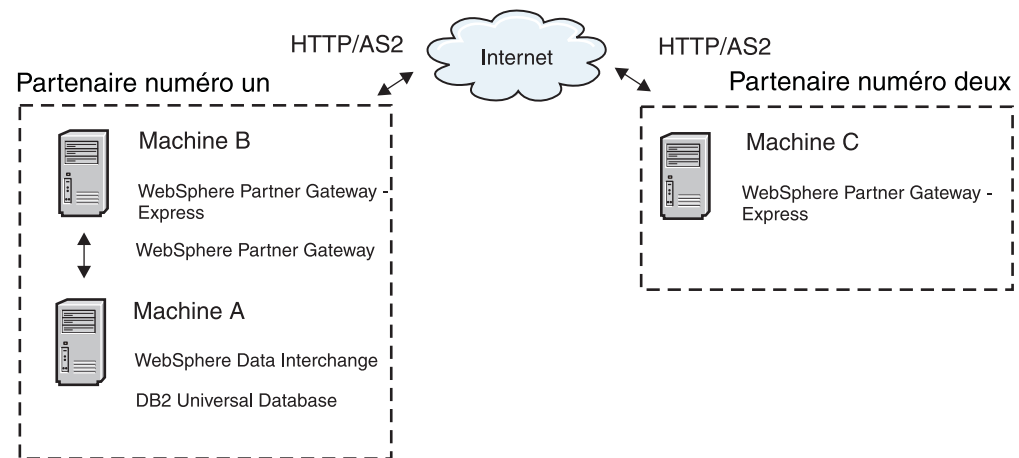
Figure 42. Configuration de deux partenaires dans un exemple de scénario
