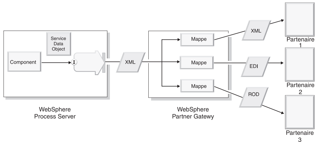
Figure 15. WebSphere Partner Gateway envoie les documents aux partenaires externes dans plusieurs formats
