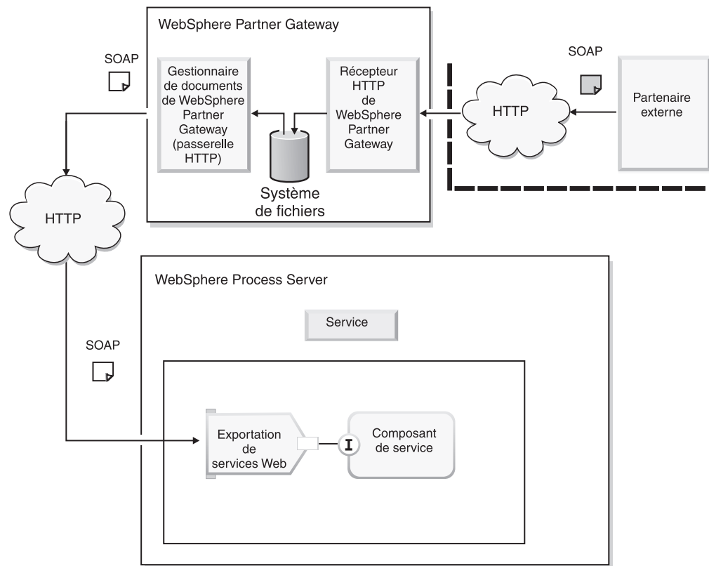
Figure 26. Partenaire externe appelant un service Web
