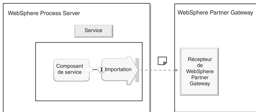
Figure 17. Utilisation de la liaison d'importation par WebSphere Process Server pour appeler WebSphere Partner Gateway
