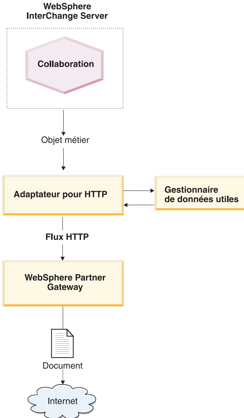
Figure 32. Flux de messages entre une collaboration et WebSphere Partner Gateway via HTTP
