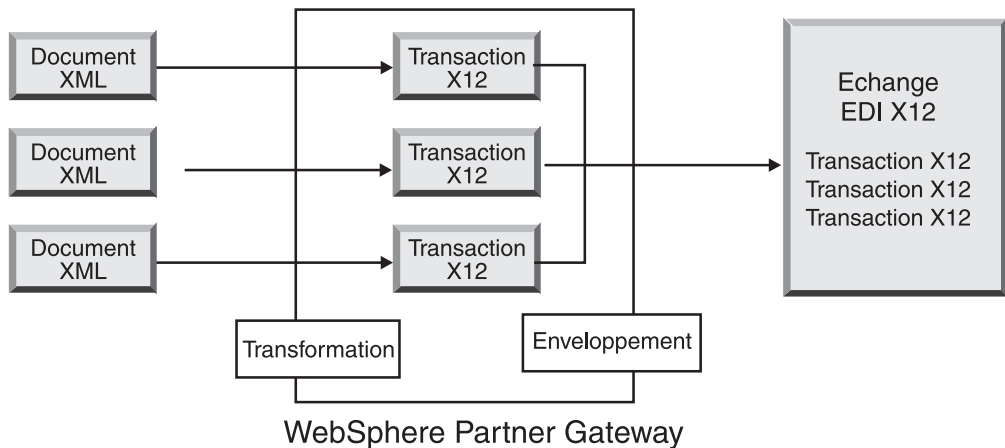
Figure 8. Documents XML envoyés de l'application dorsale au partenaire (sous forme d'échange EDI)
