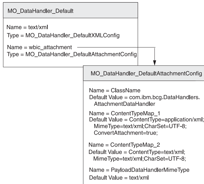
Figure 29. Association du type MIME wbic_attachment MIME au gestionnaire de données de pièces jointes
