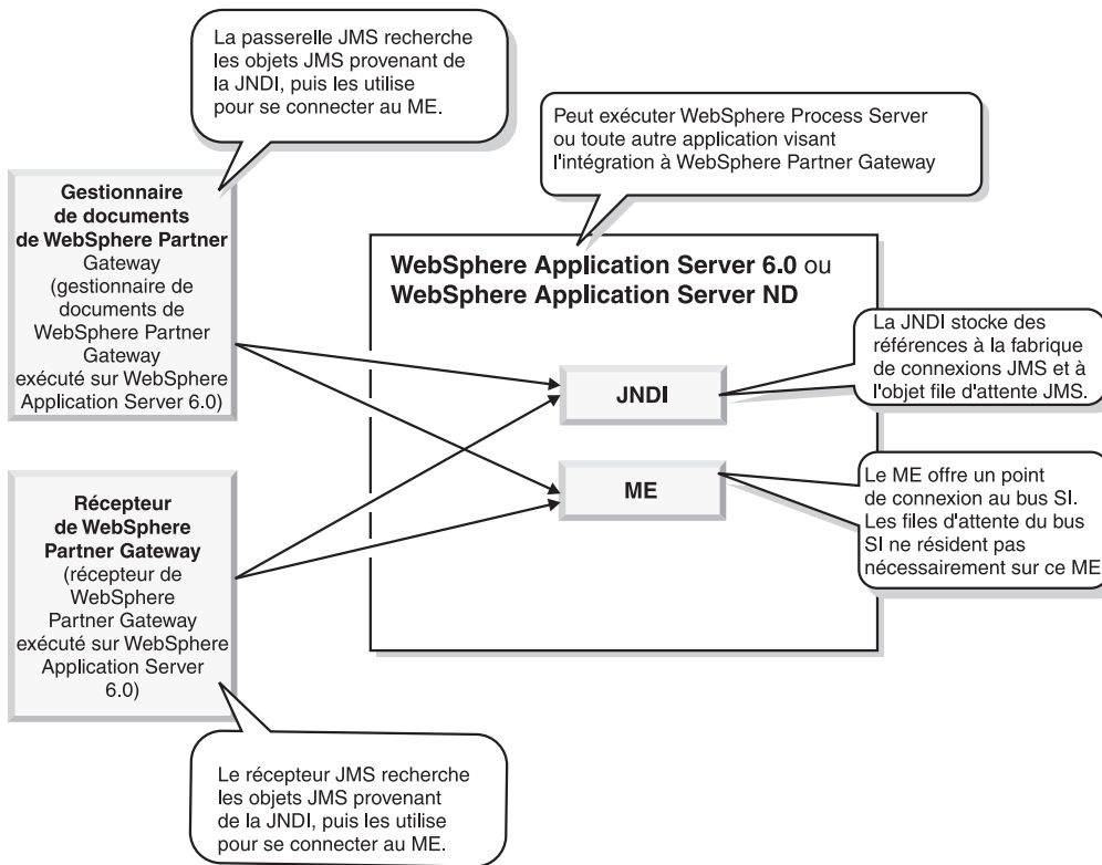
Figure 25. Accès au ME et à la JNDI à partir d'une autre instance de WebSphere Application Server
