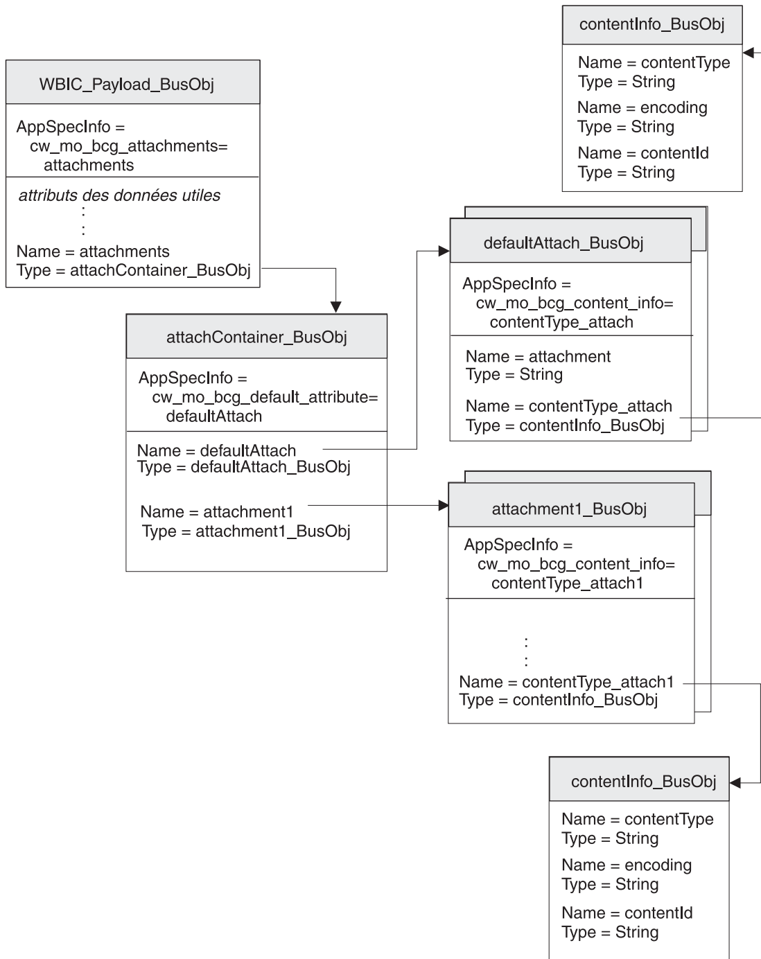
Figure 30. Relation entre l'objet métier données utiles et les objets métier pièce jointe
