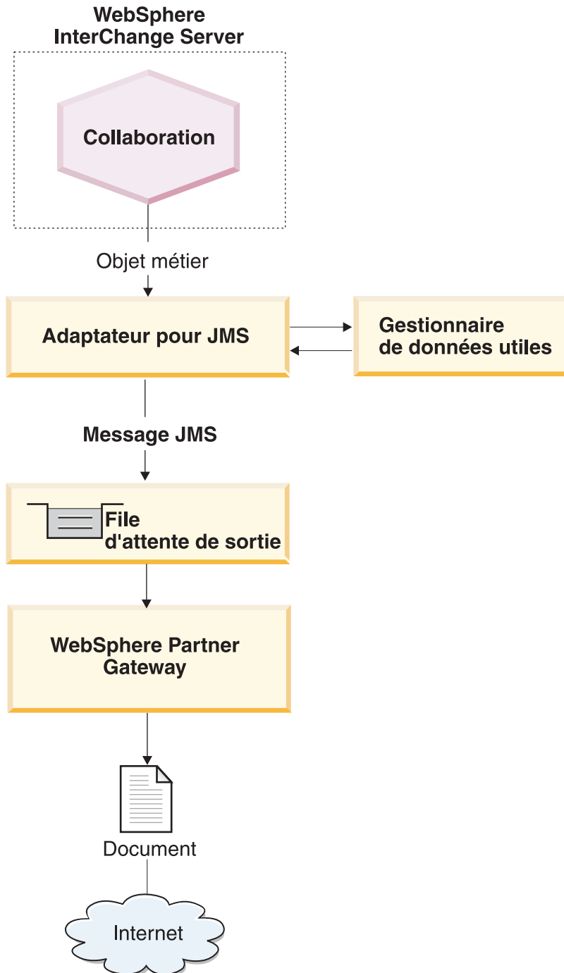
Figure 36. Flux de messages entre une collaboration et WebSphere Partner Gateway via JMS
