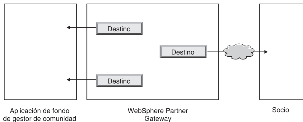
Figura 3. Destinos para el socio interno y los socios externos
