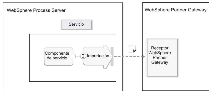
Figura 17. Cómo utiliza WebSphere Process Server el enlace de importación para invocar a WebSphere Partner Gateway
