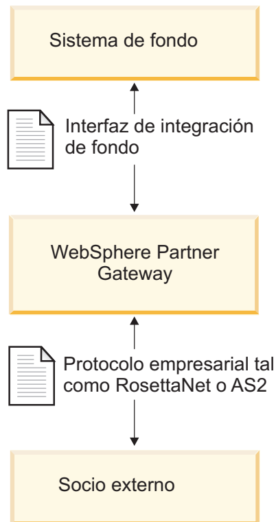
Figura 5. Rol del protocolo empresarial y empaquetado en el flujo de documentos
