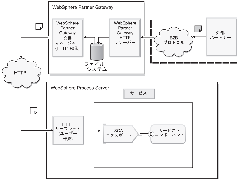
図 21. WebSphere Partner Gateway からメッセージが HTTP サブレットに送信される仕組み
