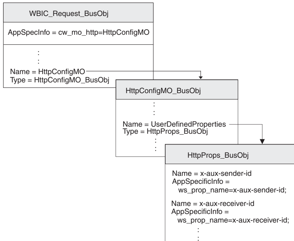
図 34. 要求ビジネス・オブジェクトと HTTP プロトコル構成メタオブジェクトとの関係
