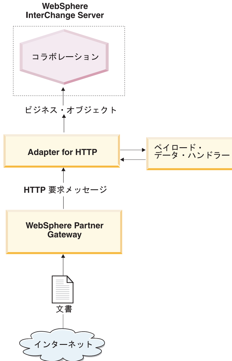
図 31. HTTP トラnsポート・プロトコルによる WebSphere Partner Gateway からコラボレーションへのメッセージ・フロー
