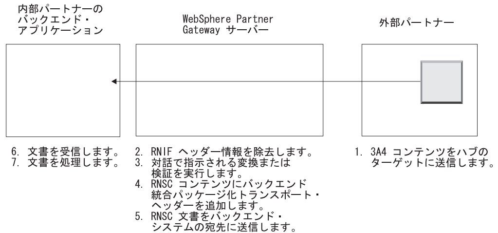
図4. バックエンド・システムへの文書フロー
