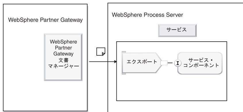
図 16. WebSphere Partner Gateway がエクスポート・バインディングを使用して文書を WebSphere Process Server に送信する仕組み
