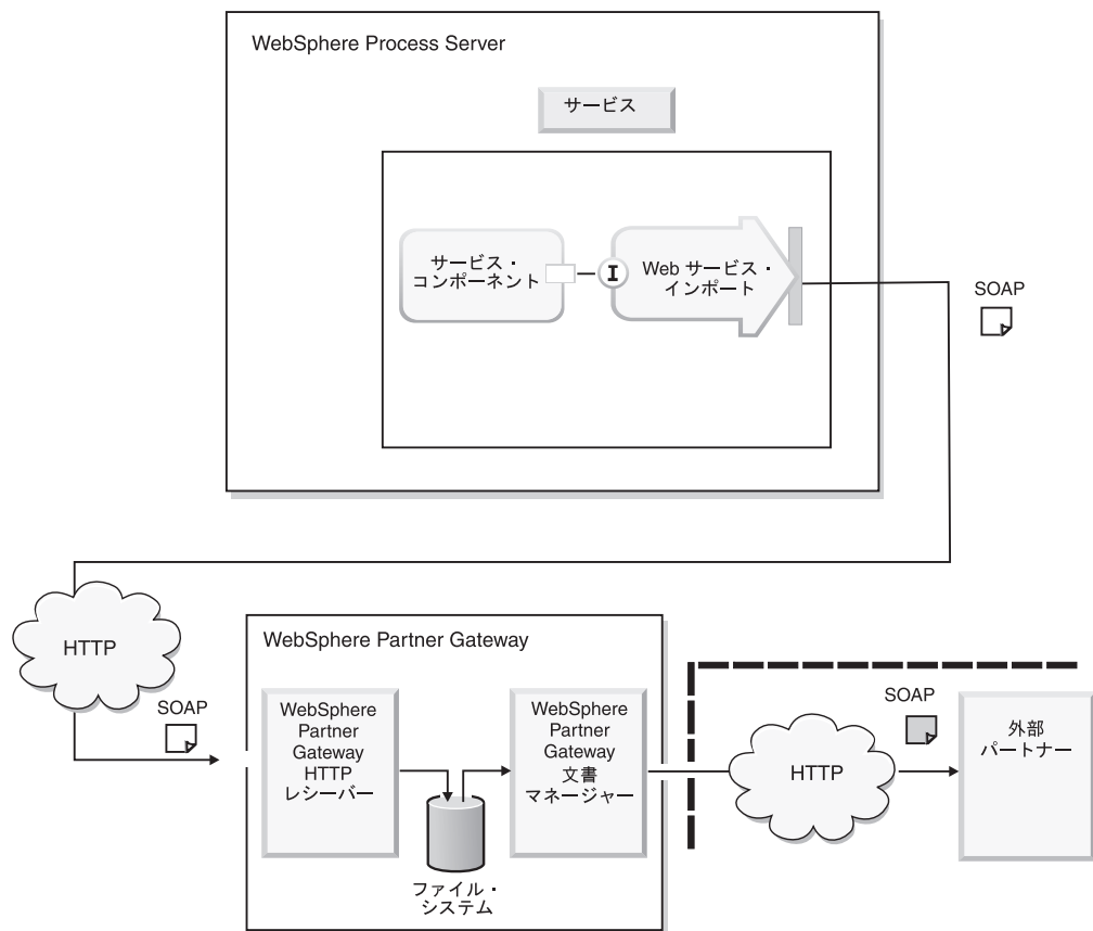
図 27. Web サービスを起動する WebSphere Process Server 上のサービス
