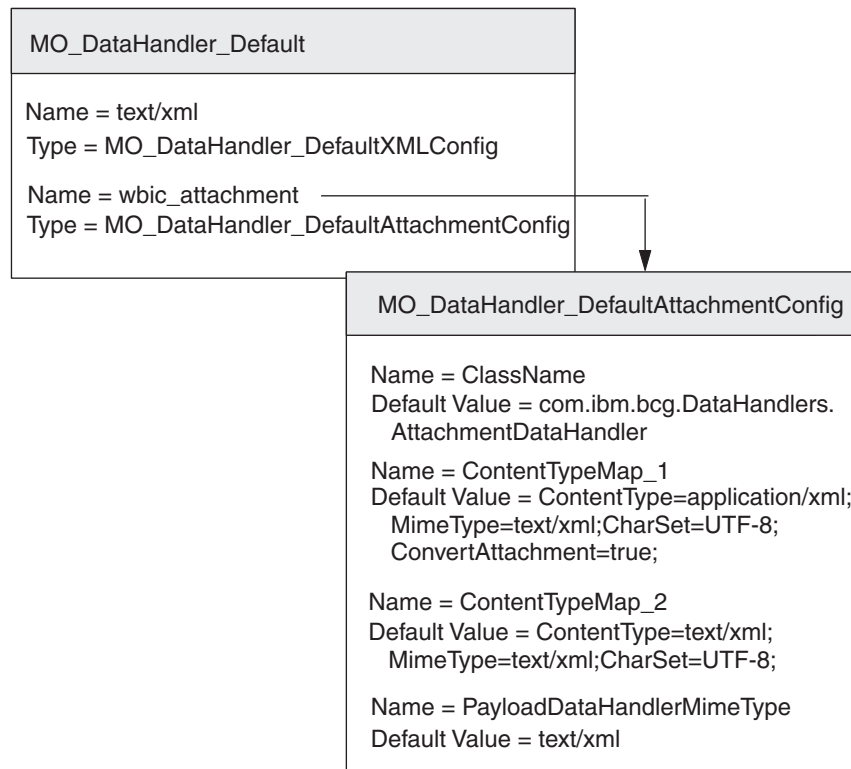
図 29. wbic_attachment MIME タイプと Attachment Data Handler との関連付け
