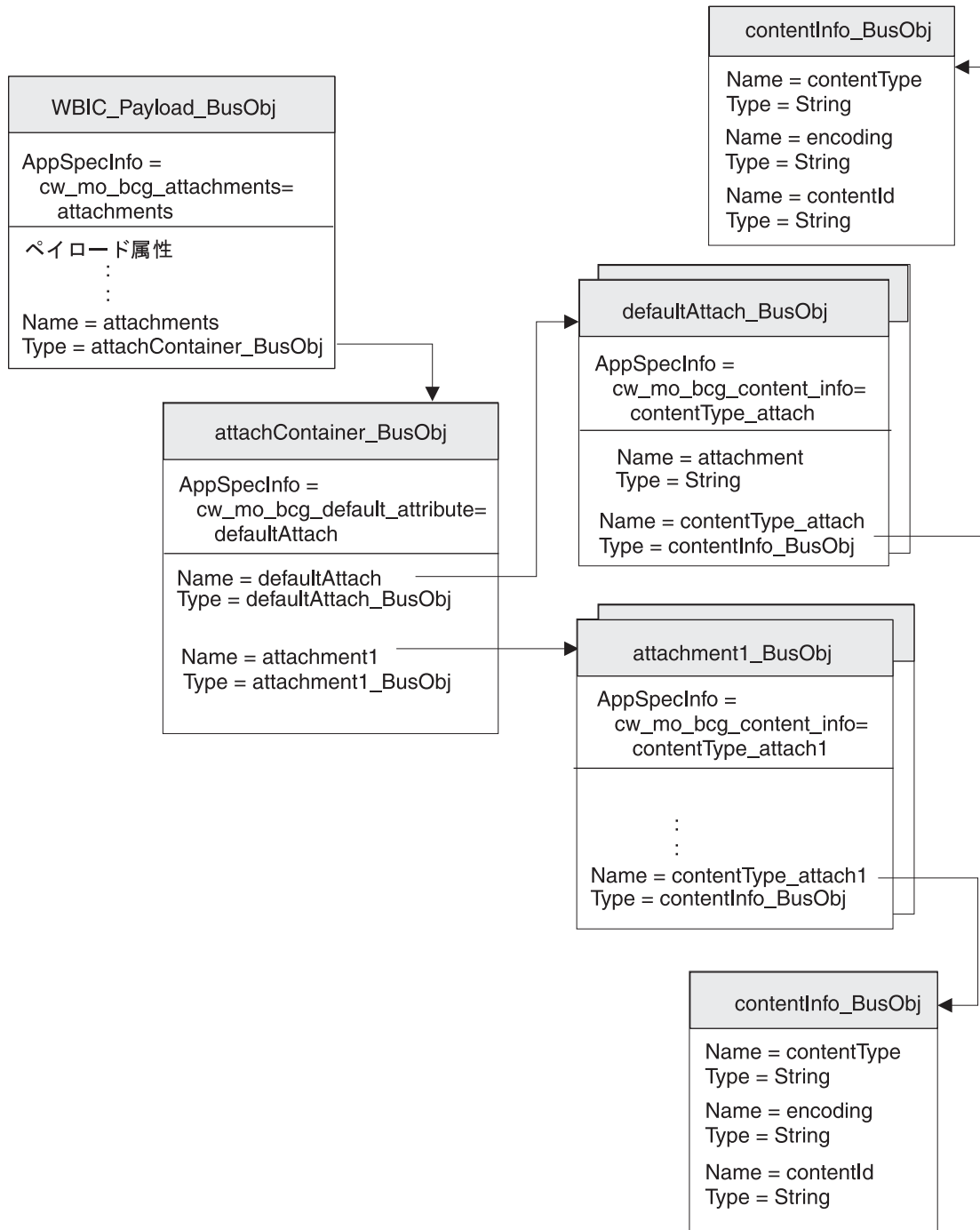
図 30. ペイロード・ビジネス・オブジェクトと添付ファイル・ビジネス・オブジェクトとの関係
