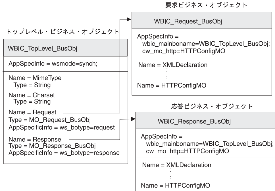
図 33. ICS 用の HTTP ペイロード・ビジネス・オブジェクトのビジネス・オブジェクト構造
