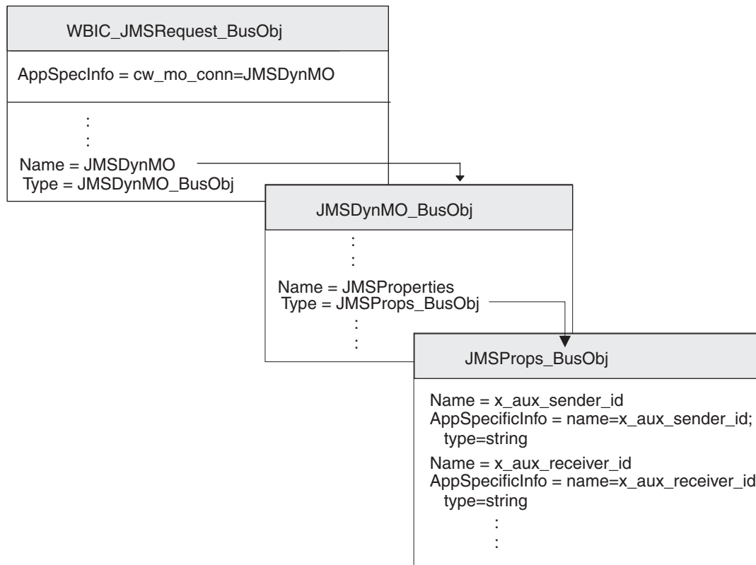
図 37. 要求ビジネス・オブジェクトと JMS 動的メタオブジェクトとの関係
