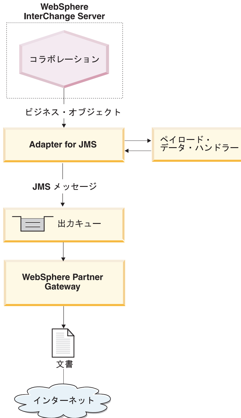
図 36. JMS トランスポート・プロトコルによるコラボレーションから WebSphere Partner Gateway へのメッセージ・フロー
