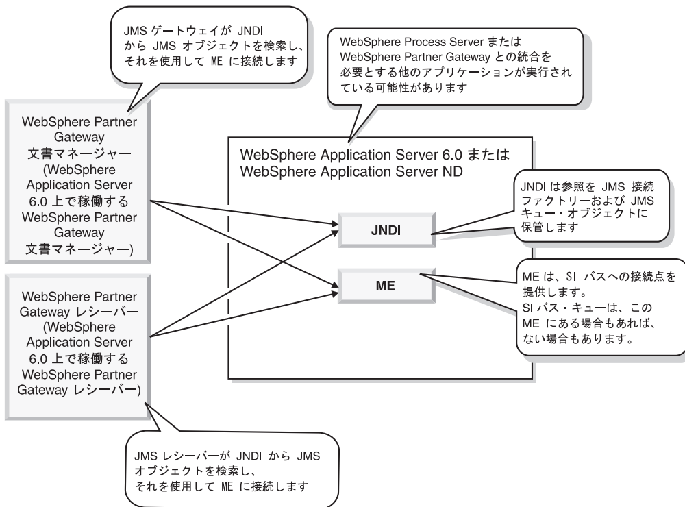
図 25. 別の WebSphere Application Server インスタンスからの ME および JNDI へのアクセス
