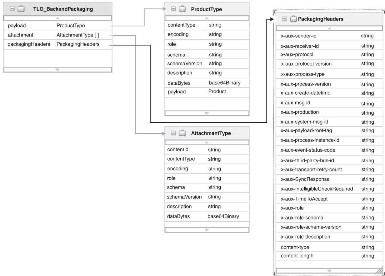
図 18. トップレベル・ビジネス・オブジェクト
