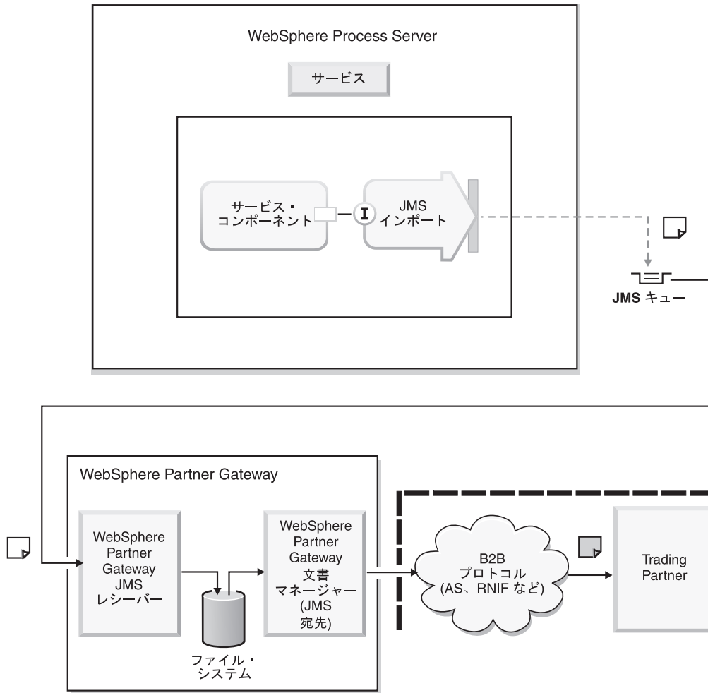
図 24. JMS を介して文書を受信する JMS インポート
