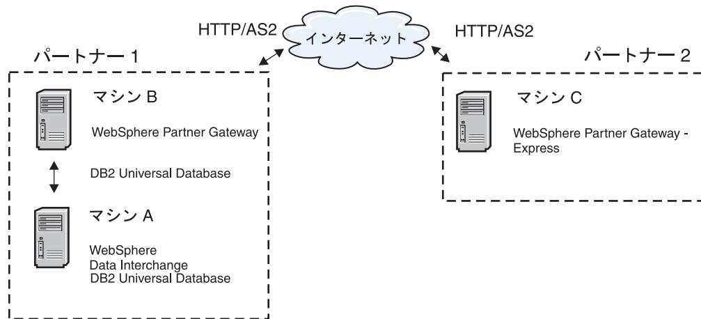
図 42. サンプル・シナリオでの 2 つのパートナーの構成
