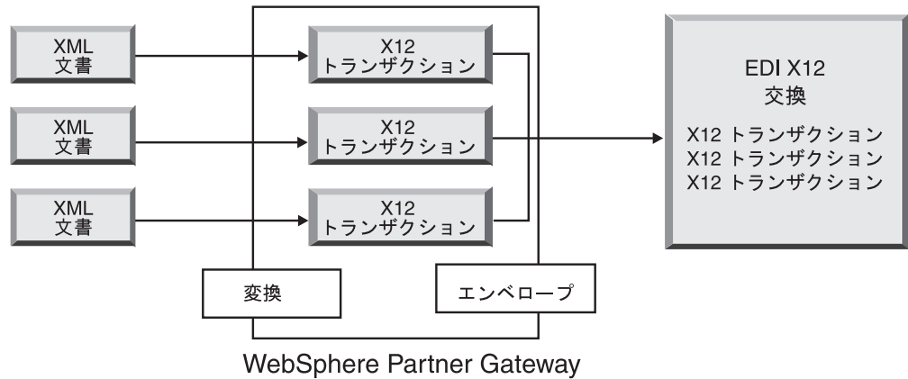
図8. バックエンド・アプリケーションからパートナーへ (1 つの EDI 交換として) 送信される複数の XML 文書
