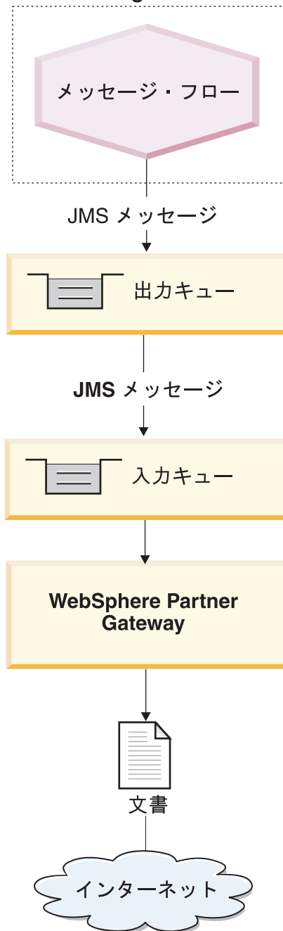
図 39. JMS トラnsポート・プロトコルによるメッセージ・フローから WebSphere Partner Gateway へのメッセージ・フロー
