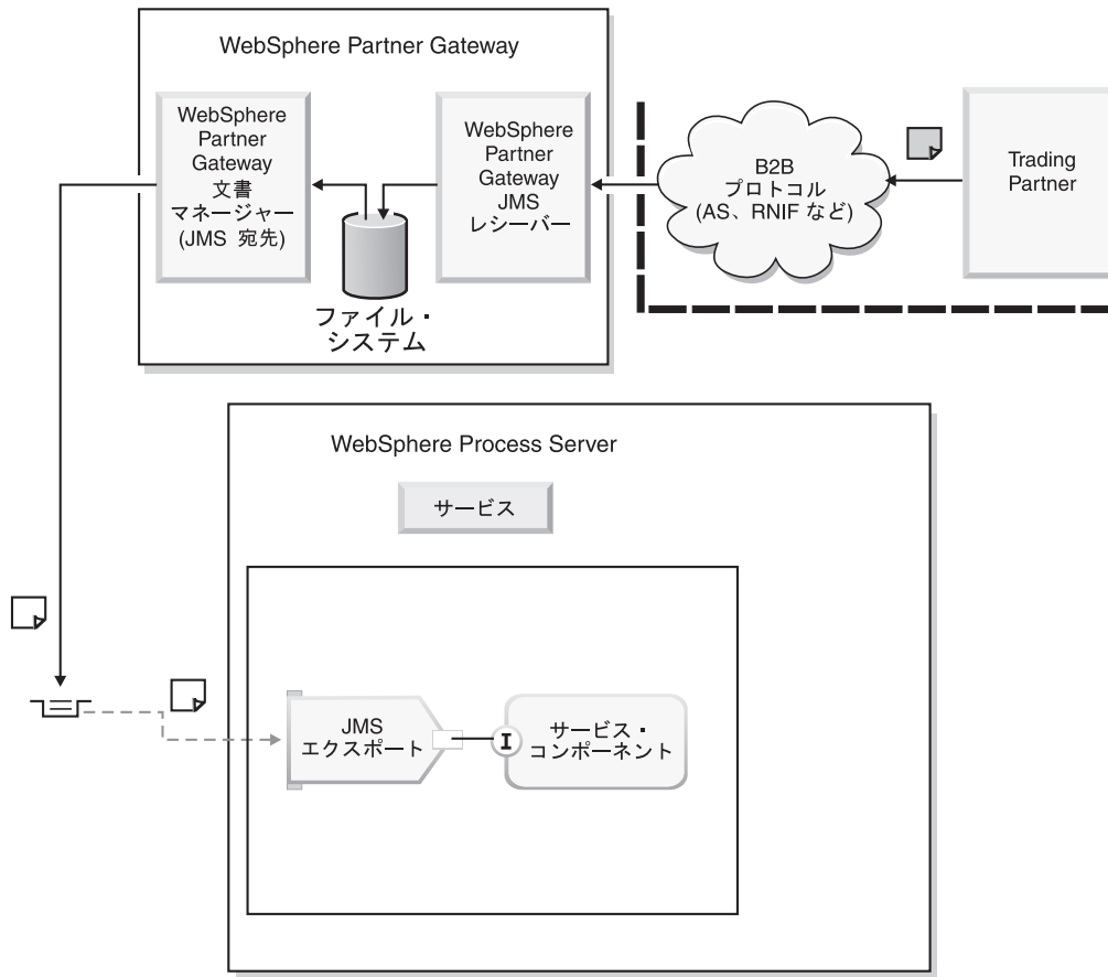
図 23. JMS を介して SCA サービスを呼び出す JMS エクスポート
