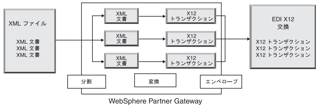
図 10. バックエンド・アプリケーションから送信され、分割され、パートナーへ (1 つの EDI 交換として) 送信される複数の XML 文書
