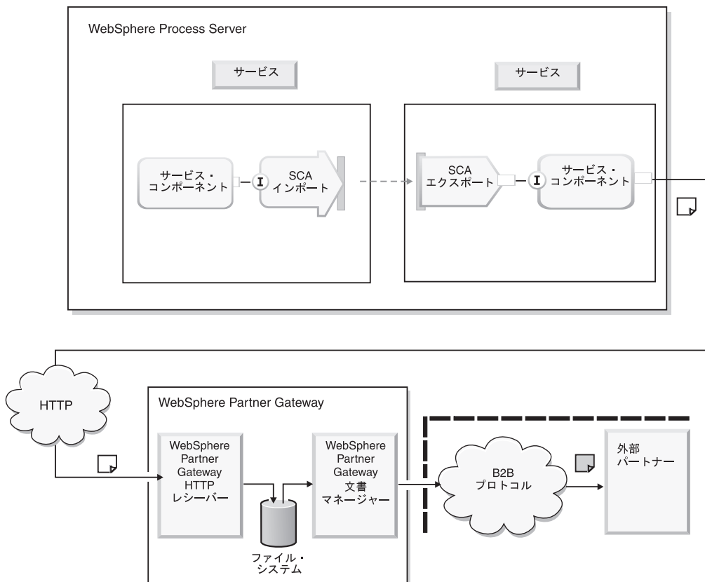
図 22. WebSphere Process Server から WebSphere Partner Gateway 上の HTTP レシーバーにメッセージを送信する仕組み
