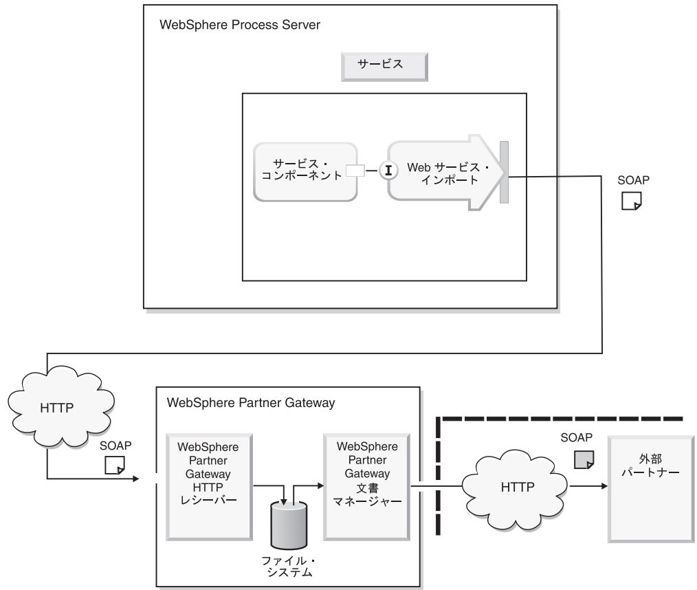
図2. 内部パートナーおよび外部パートナー用のレシーバー
