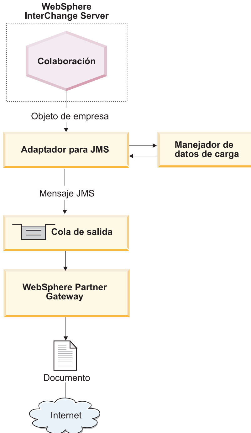
Figura 36. Flujo de mensajes desde una colaboración a WebSphere Partner Gateway mediante el protocolo de transporte JMS
