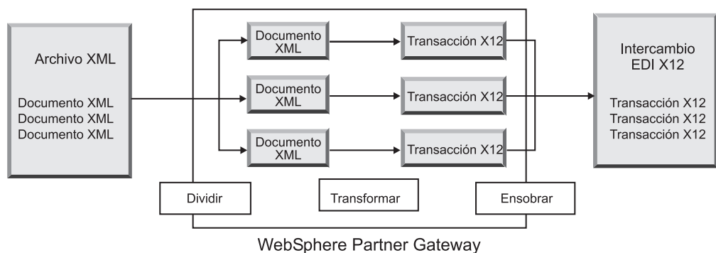
Figura 10. Varios documentos XML enviados desde una aplicación de programa de fondo, divididos y, a continuación, enviados al socio (como un intercambio EDI)
