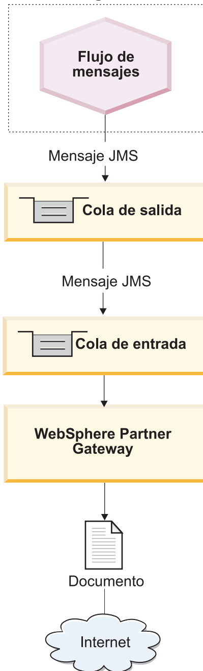
Figura 39. Flujo de mensajes desde un flujo de mensajes a WebSphere Partner Gateway a través el protocolo de transporte JMS
