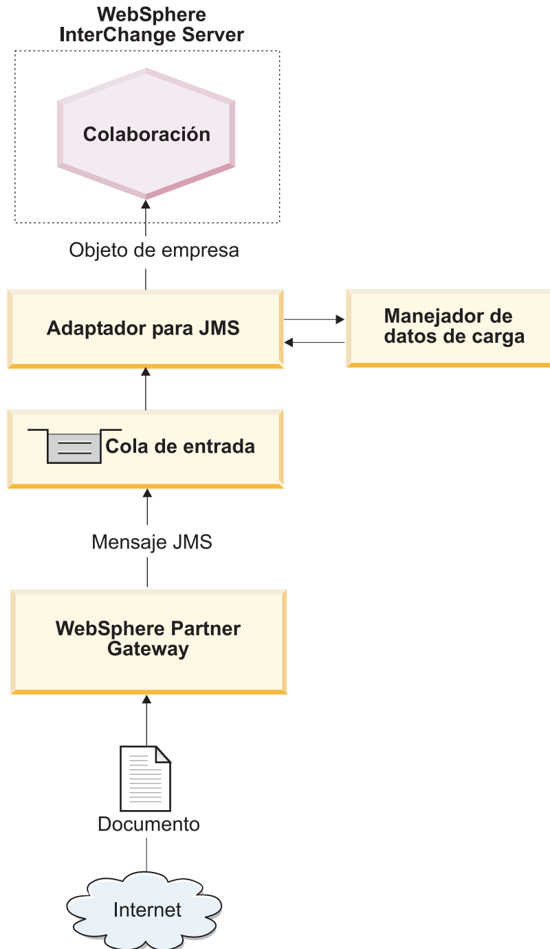
Figura 35. Flujo de mensajes desde WebSphere Partner Gateway a una colaboración a través del protocolo de transporte JMS
