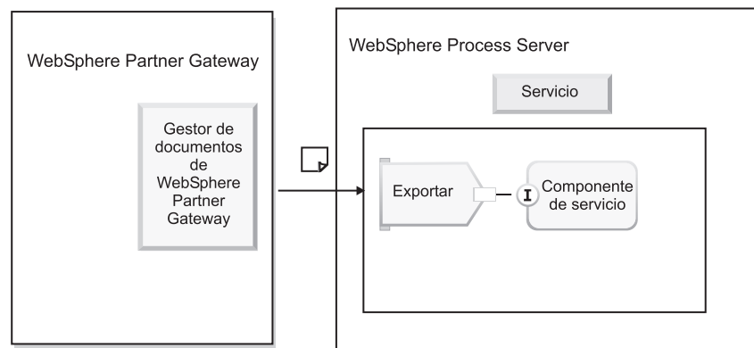
Figura 16. Cómo utiliza WebSphere Partner Gateway el enlace de exportación para enviar documentos a WebSphere Process Server
