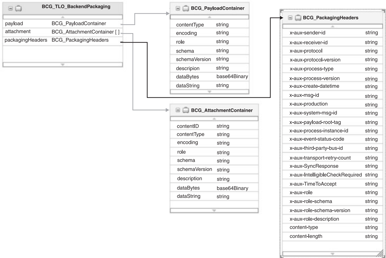
Figura 19. Objeto de empresa de nivel superior predeterminado
