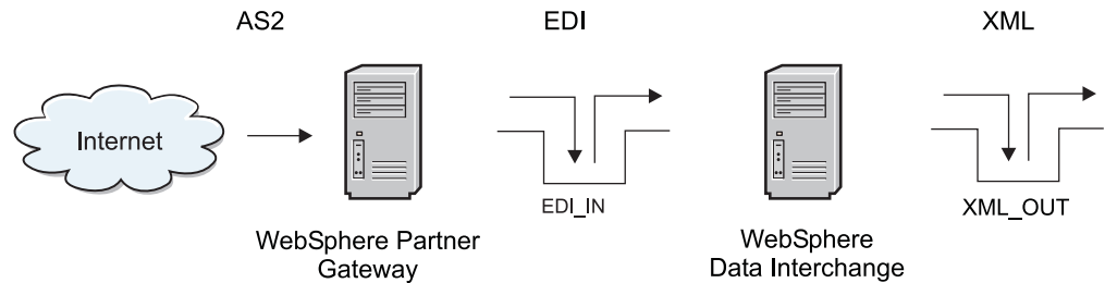
Figura 40. Documento EDI de WebSphere Partner Gateway
