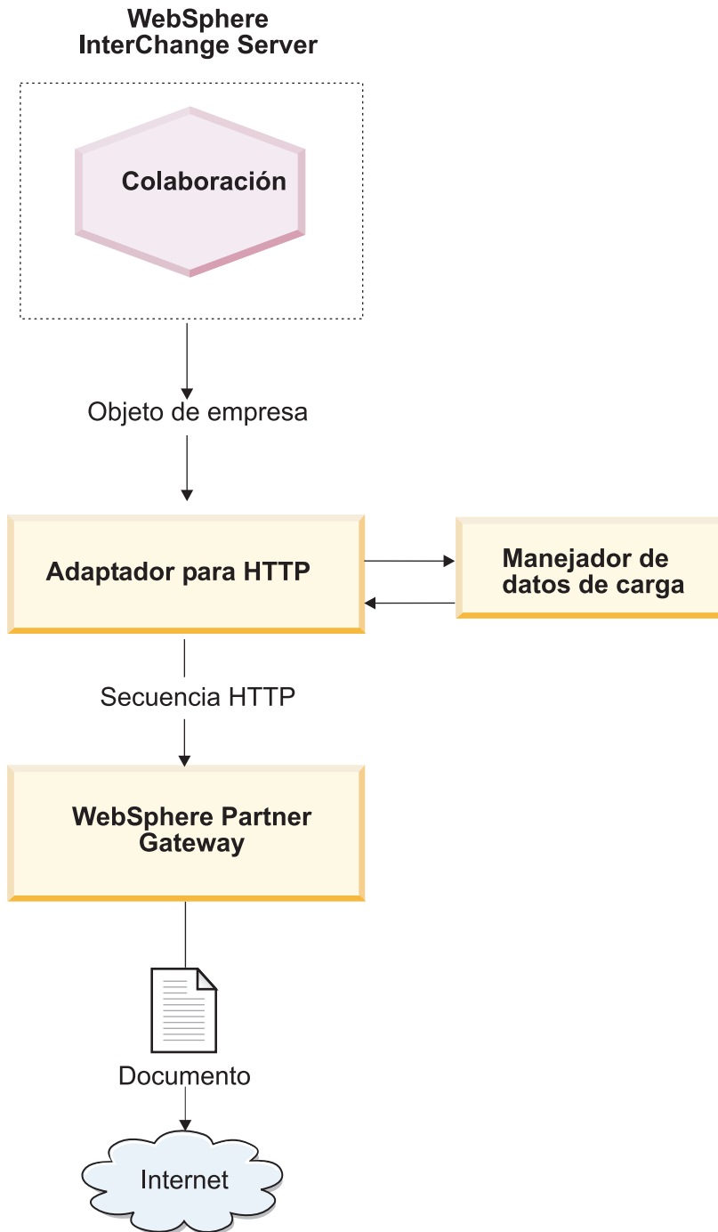
Figura 32. Flujo de mensajes desde una colaboración a WebSphere Partner Gateway a través del protocolo de transporte HTTP
