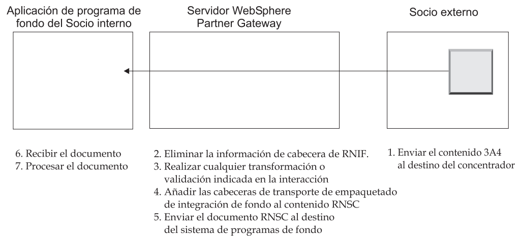
Figura 4. Cómo fluye un documento al sistema de fondo
