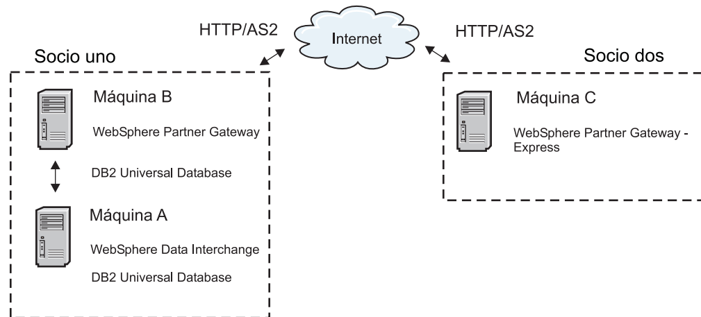
Figura 42. Configuración de dos socios en el caso de ejemplo
