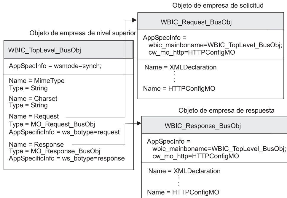
Figura 33. Estructura del objeto de empresa para el objeto de empresa de carga HTTP para ICS
