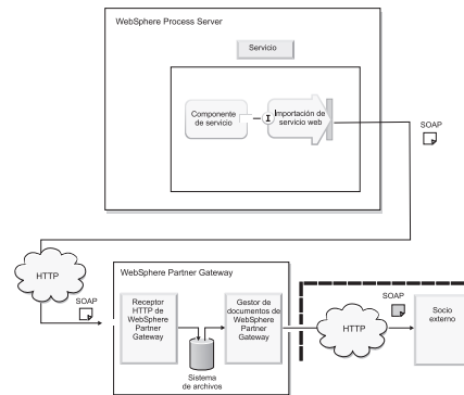
Figura 2. Receptores para el socio interno y los socios externos.
