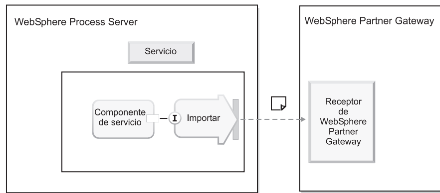
Figura 17. Cómo utiliza WebSphere Process Server el enlace de importación para invocar a WebSphere Partner Gateway
