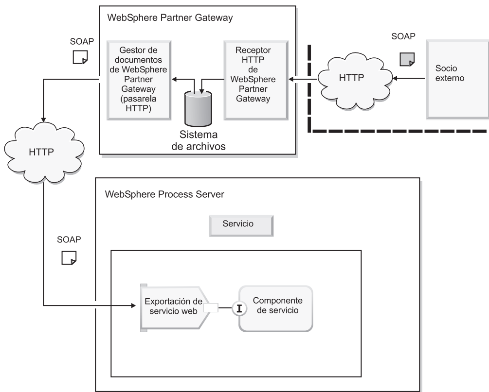
Figura 26. Socio externo que invoca un servicio web
