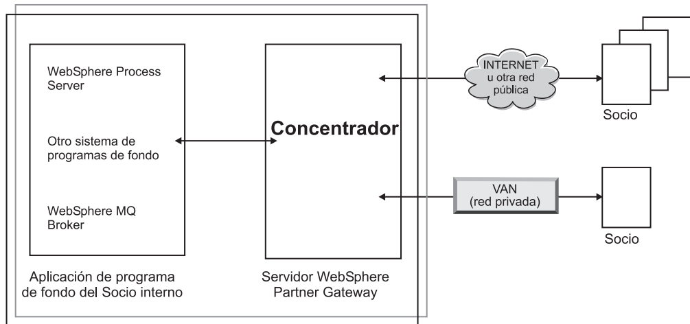
Figura 1. Flujo de documentos de extremo a extremo
