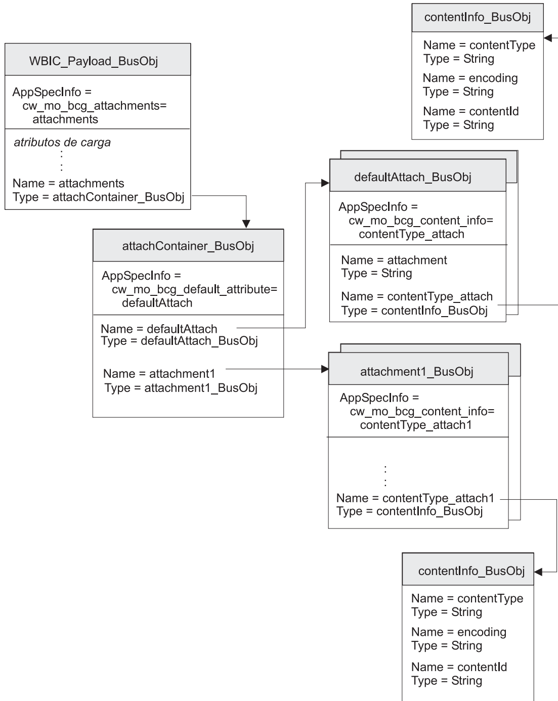
Figura 30. Relación del objeto de empresa de carga con los objetos de empresa de archivo adjunto
