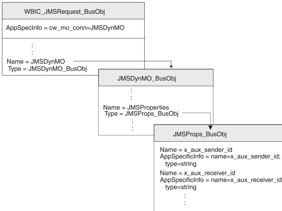
Figura 37. Relación del objeto de empresa de solicitud con el metaobjeto dinámico JMS
