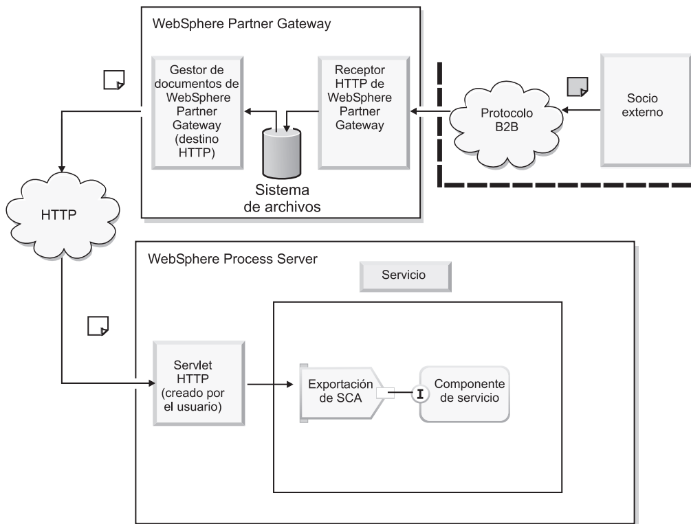
Figura 21. Cómo se envía un mensaje de WebSphere Partner Gateway al servlet HTTP
