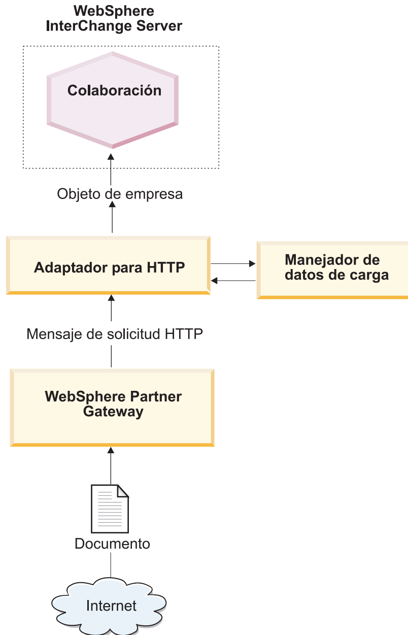
Figura 31. Flujo de mensajes desde WebSphere Partner Gateway a una colaboración a través del protocolo de transporte HTTP
