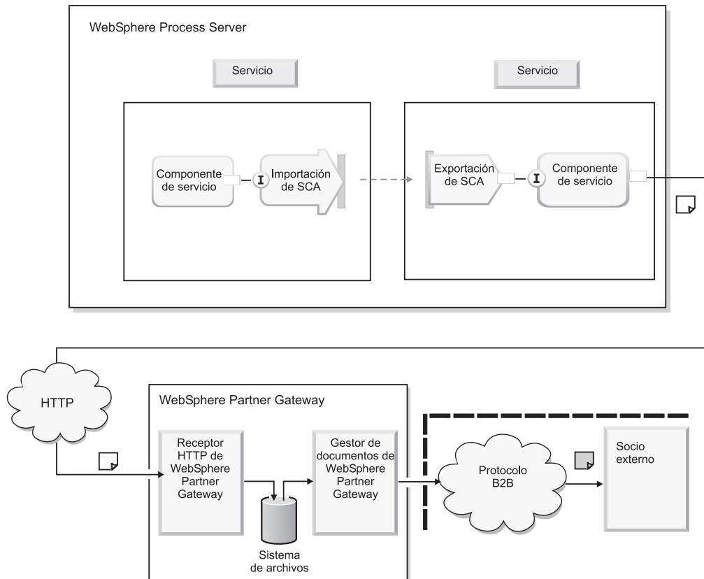
Figura 22. Cómo se envía un mensaje de WebSphere Process Server al receptor HTTP en WebSphere Partner Gateway
