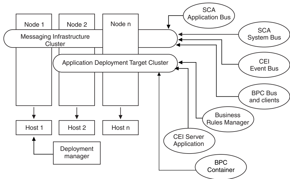
Rysunek 6. Remote messaging pattern
