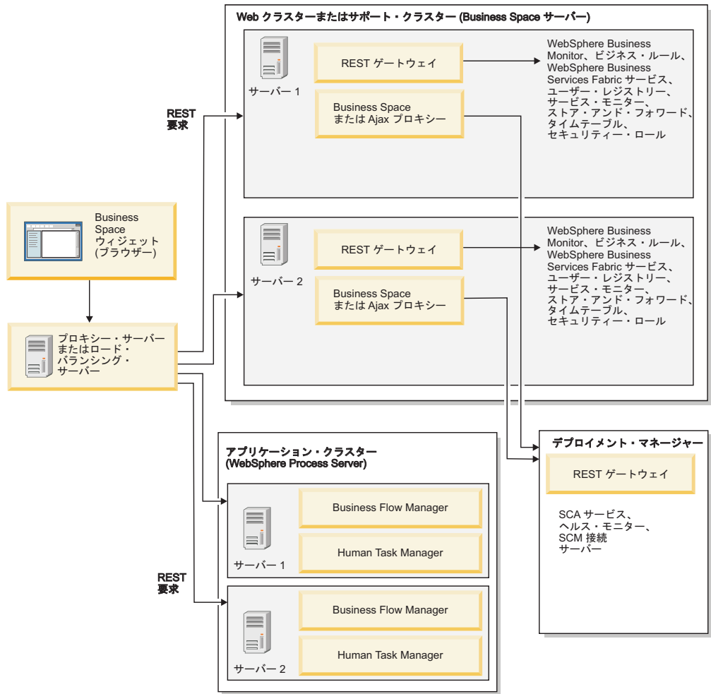
図 1. 標準的トポロジー
