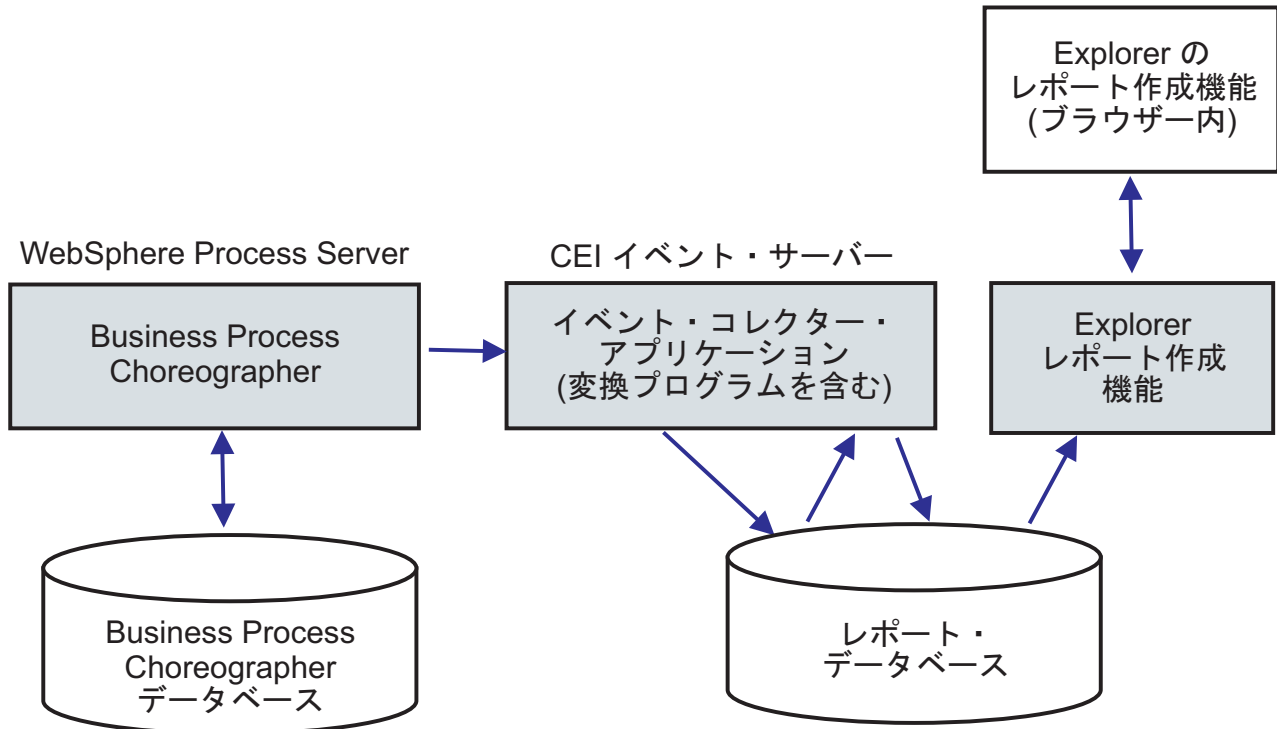
図 16. 実動パフォーマンスを考慮した Business Process Choreographer Explorer レポート作成のセットアップ
