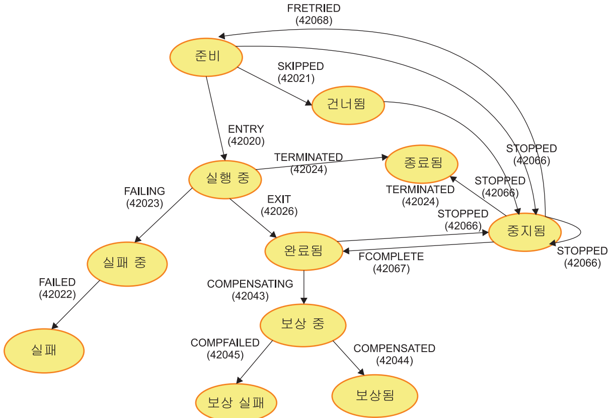
그림 6. 범위 활동에 대한 상태 전이 및 이벤트
