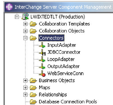
Figure 28. Dossier Connecteurs dans la vue Gestion de composant InterChange Server
