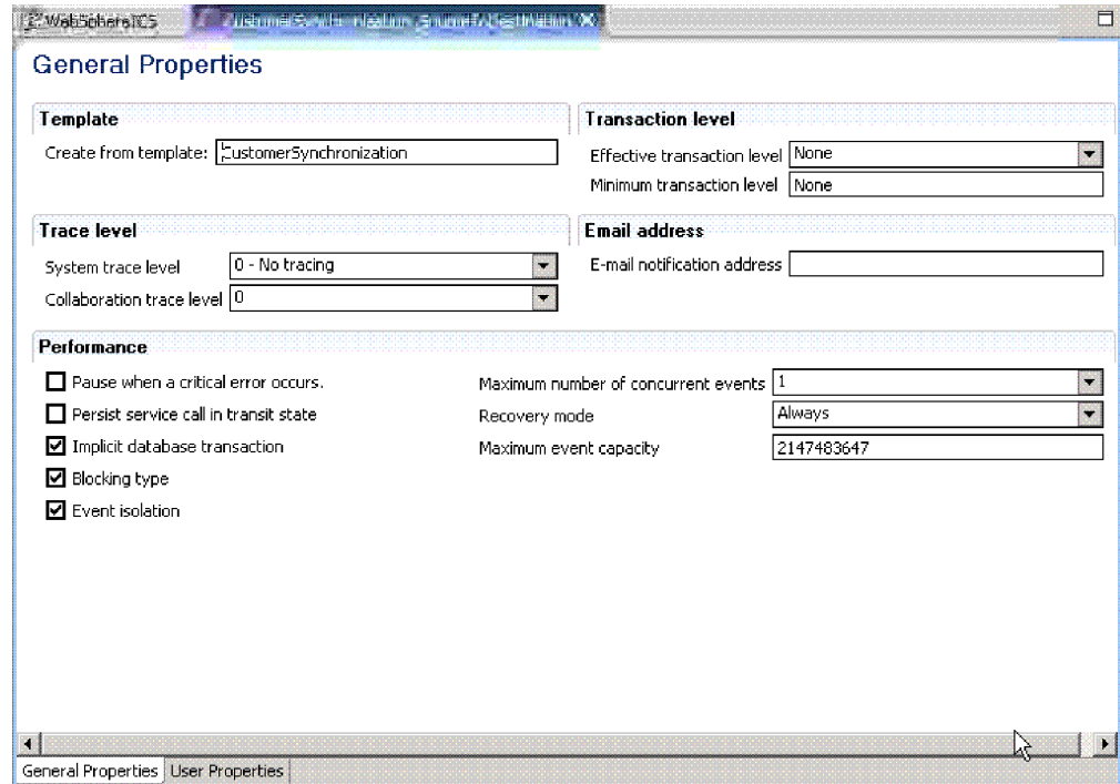
Figure 33. Boîte de dialogue Propriétés, onglet Propriétés générales de collaboration
