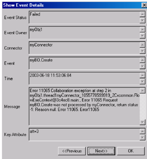
Figure 73. Boîte de dialogue Afficher le détail des événements de Flow Manager
