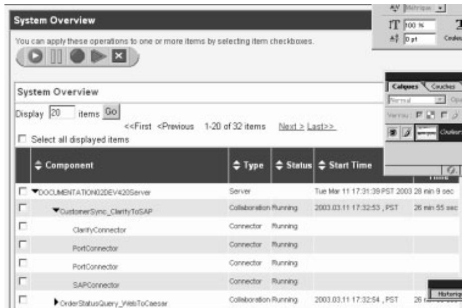
Figure 27. System Monitor, Aperçu général du système affichant l'état des connecteurs
