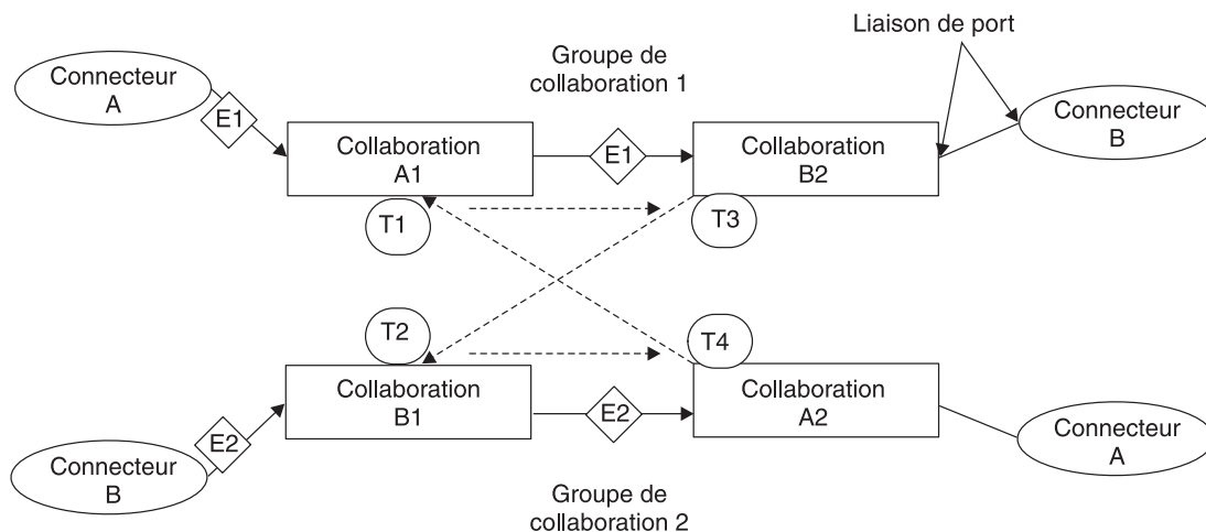
Figure 75. Blocage entre groupes de collaborations
