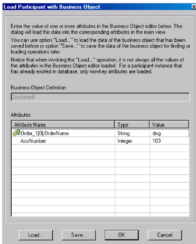
Figure 43. Boîte de dialogue Charger le participant avec l'objet métier
