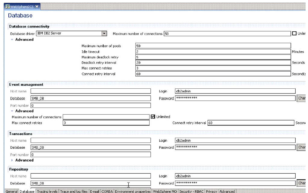
Figure 21. Onglet Base de données de la fenêtre Modifier la configuration
