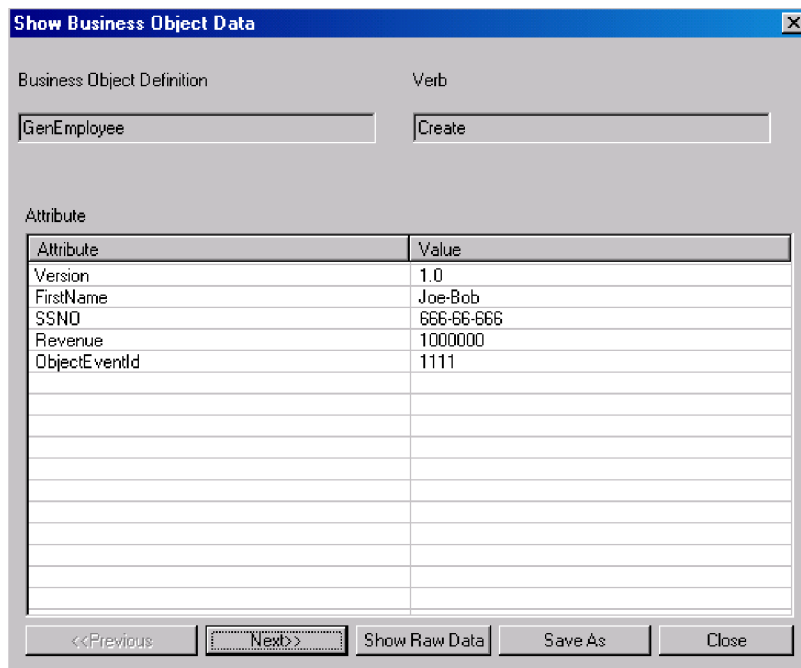
Figure 74. Boîte de dialogue Affichage des données d'objet métier
