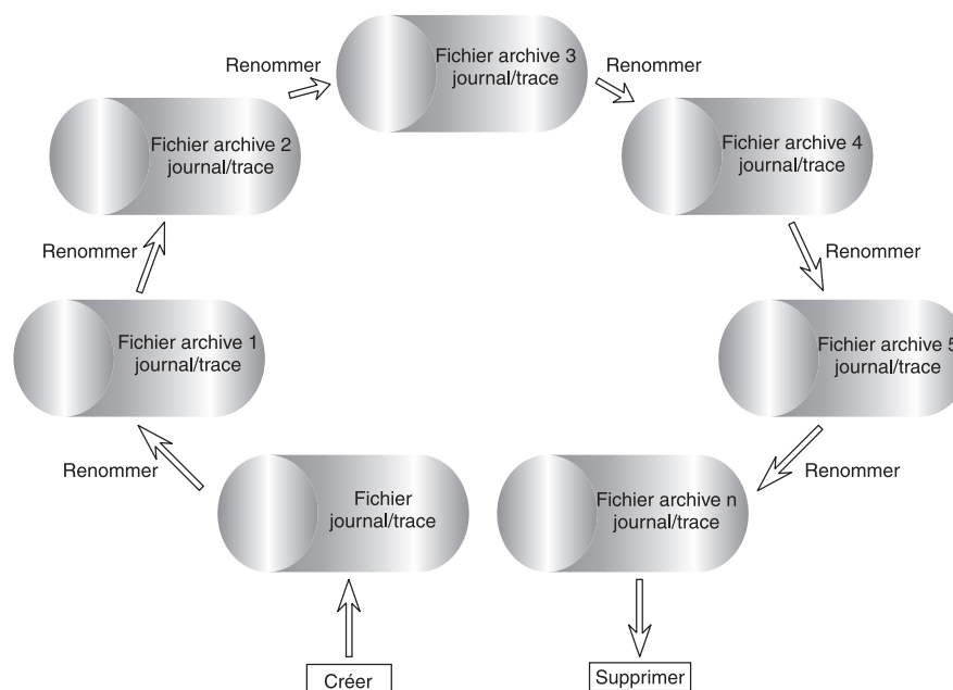
Figure 51. Journalisation d'archivage circulaire
