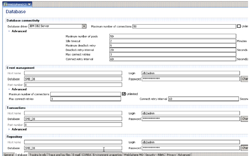
Figure 76. Ecran Modifier la configuration, onglet Base de données
