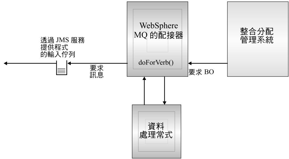
圖 2. 應用程式與連接器的通訊方法：訊息要求
