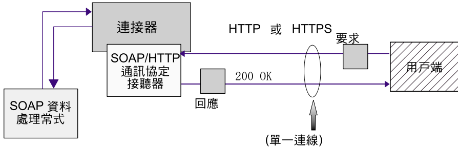
圖 24. SOAP/HTTP 通訊協定接聽器：同步的事件處理程序
