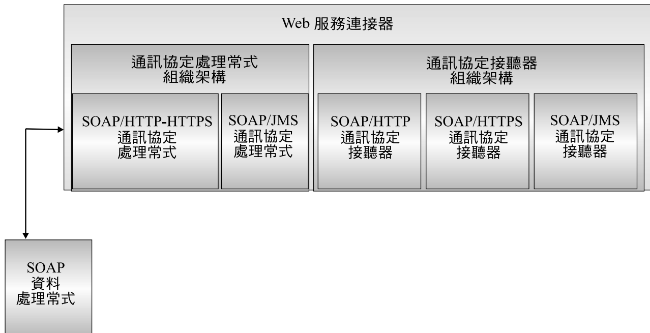
圖 1. Web 服務的連接器
