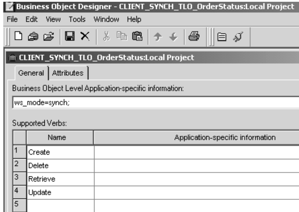
図 11. 同期要求処理のためのトップレベル・ビジネス・オブジェクト
