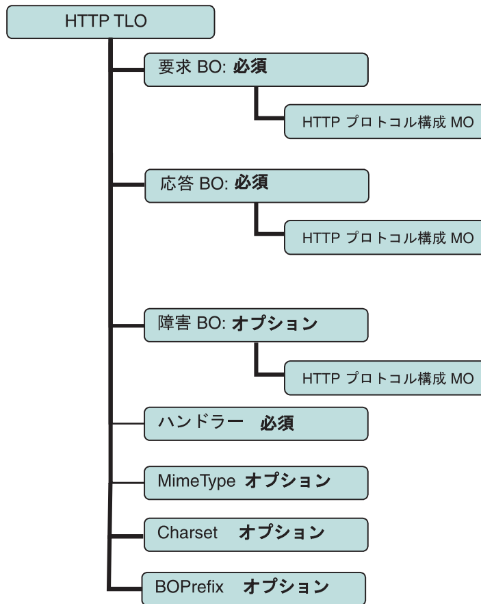
図 10. 同期要求処理のためのビジネス・オブジェクト階層
