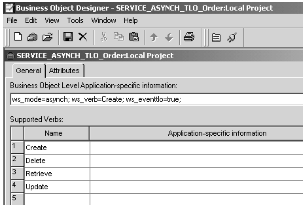
図 8. 非同期イベント処理のためのトップレベル・ビジネス・オブジェクト
