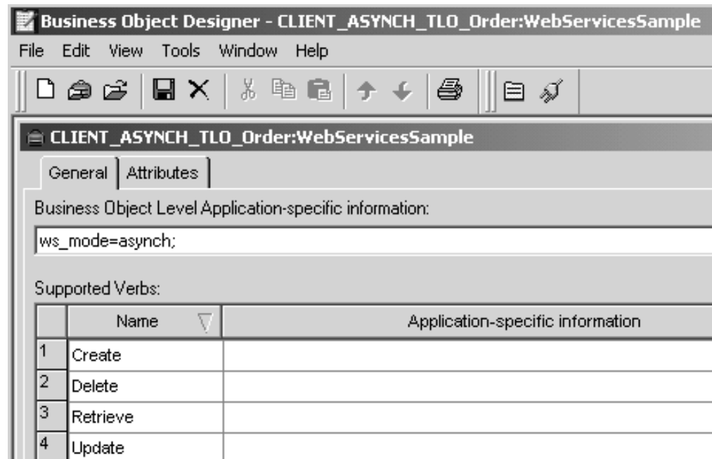
図 13. 非同期要求処理のためのトップレベル・ビジネス・オブジェクト
