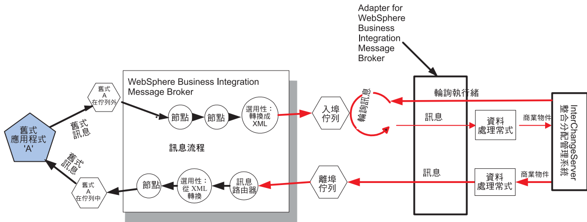
圖 1. WebSphere Business Integration 環境中的配接器
