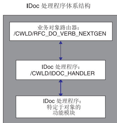
图 75. IDoc 处理程序体系结构
