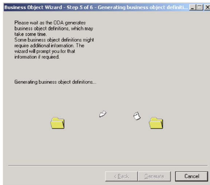
图 11. 生成定义
