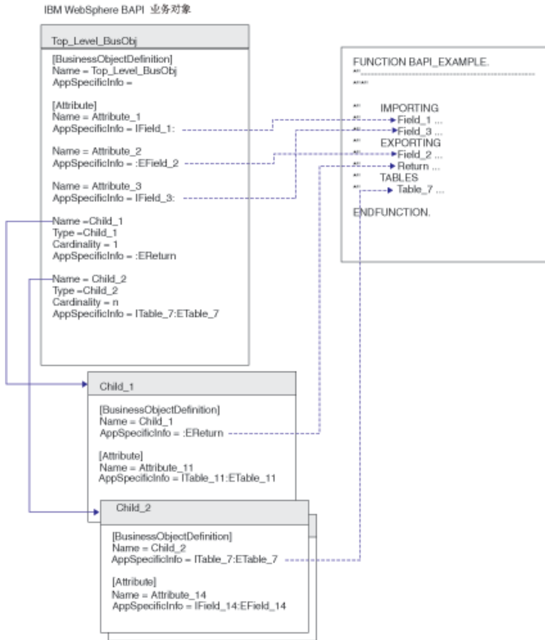
图 58. 业务对象和示例 BAPI 之间的映射
