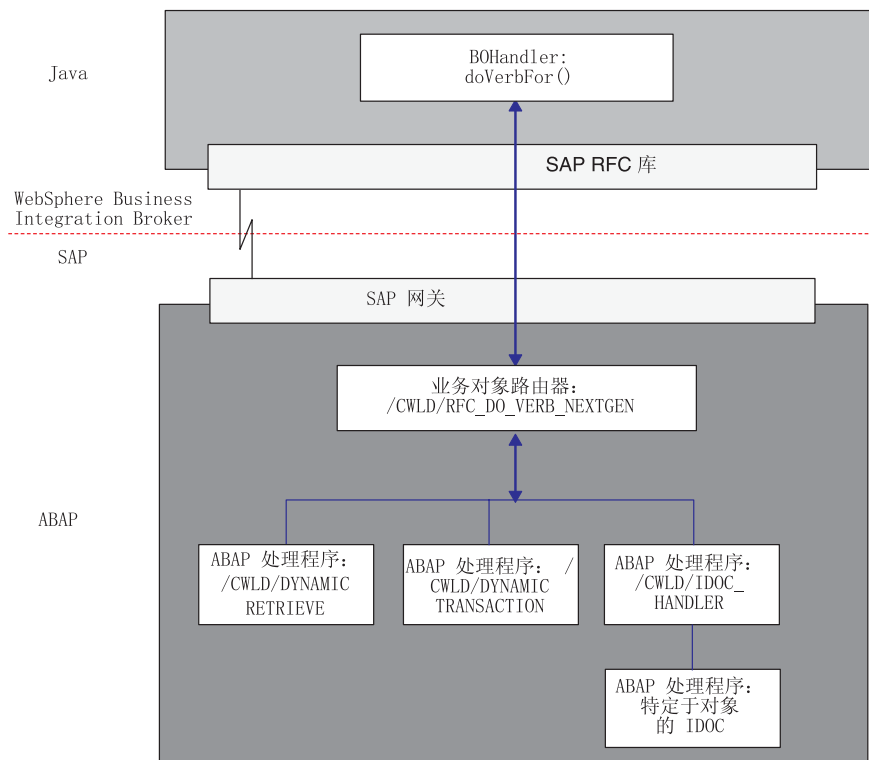
图 66. 适配器提供的业务对象处理组件
