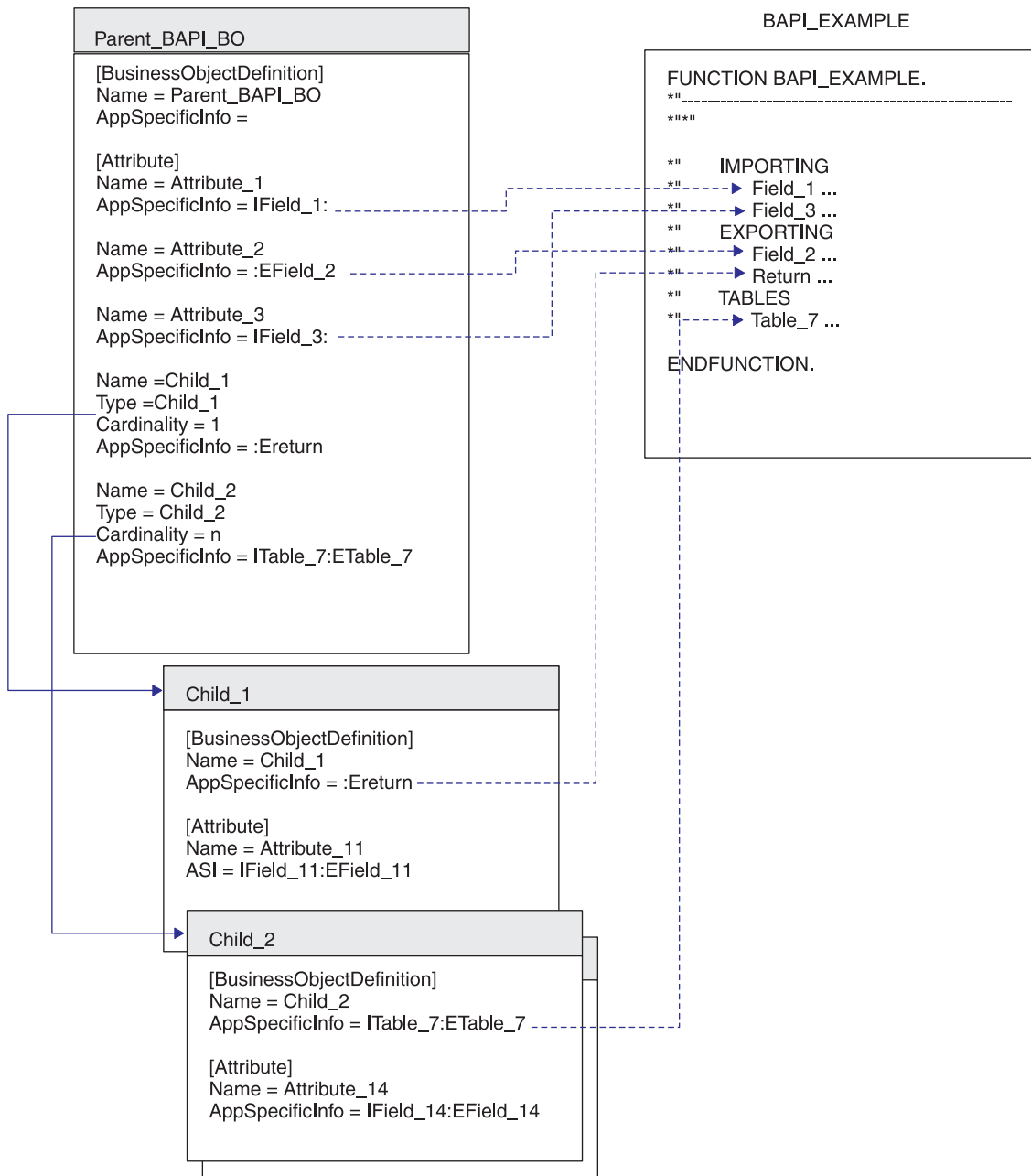
图 49. 业务对象和示例 BAPI 之间的对应项
