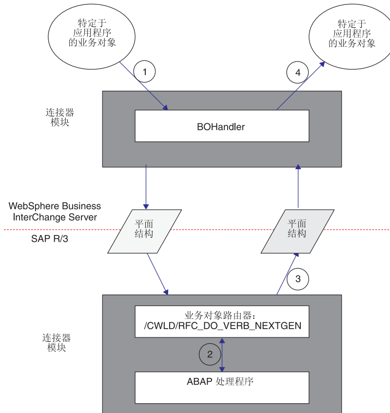
图 71. 业务对象处理
