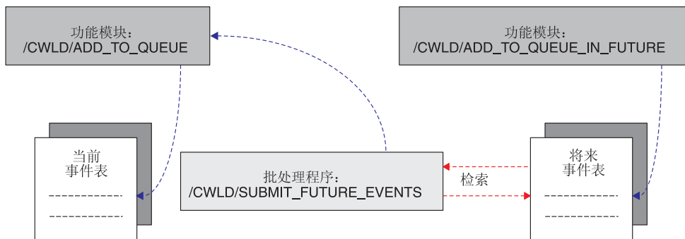
图 69. /CWLD/ADD_TO_QUEUE_IN_FUTURE
