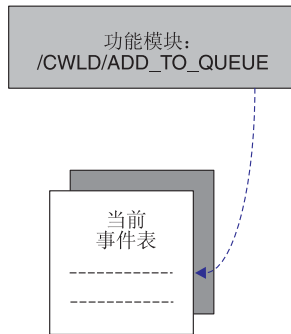
图 68. /CWLD/ADD_TO_QUEUE
