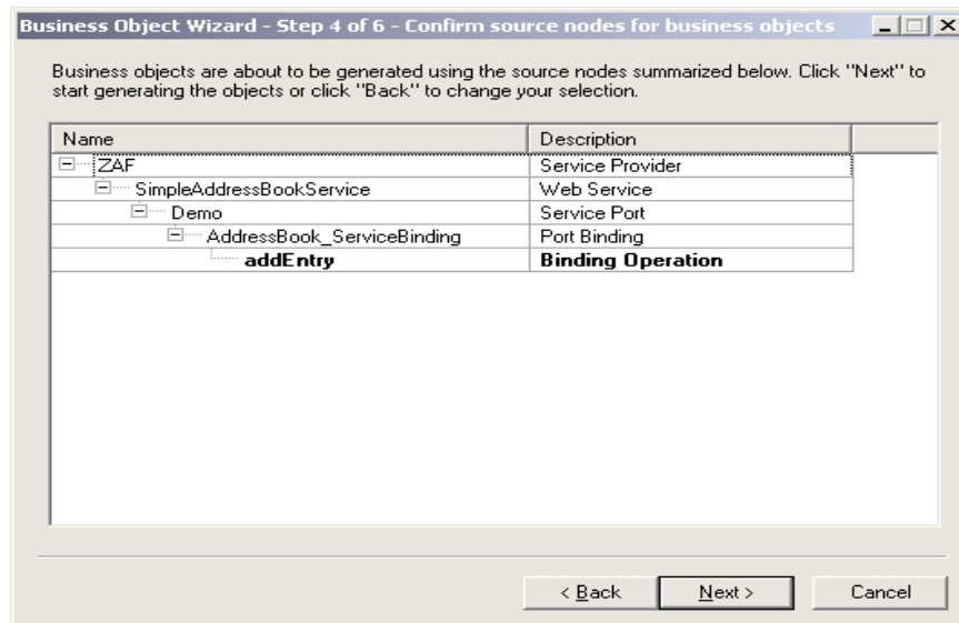
圖 67. 「確認」視窗
