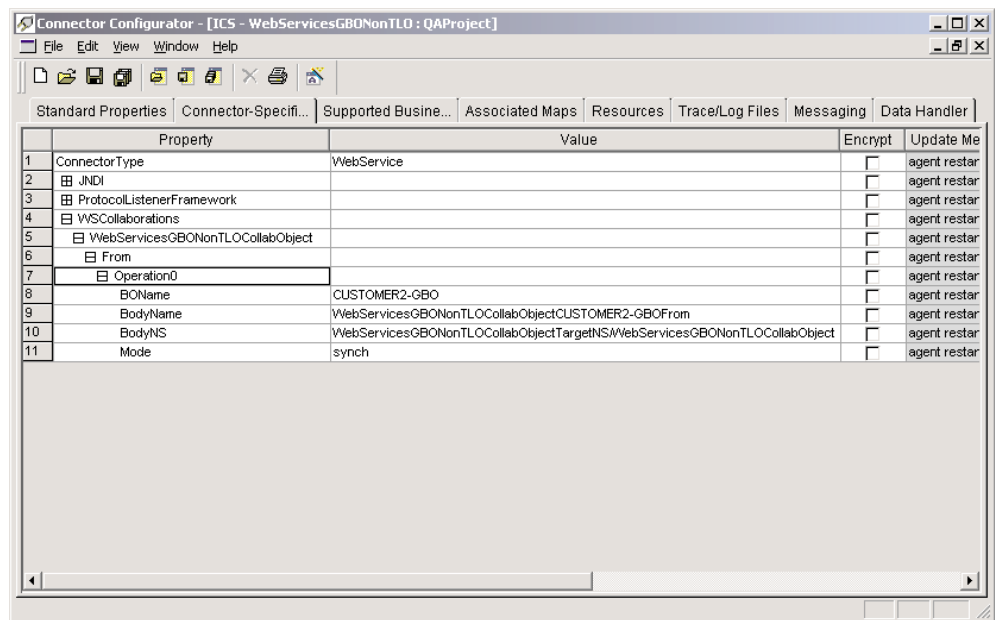
圖 61. WSCollaborations
