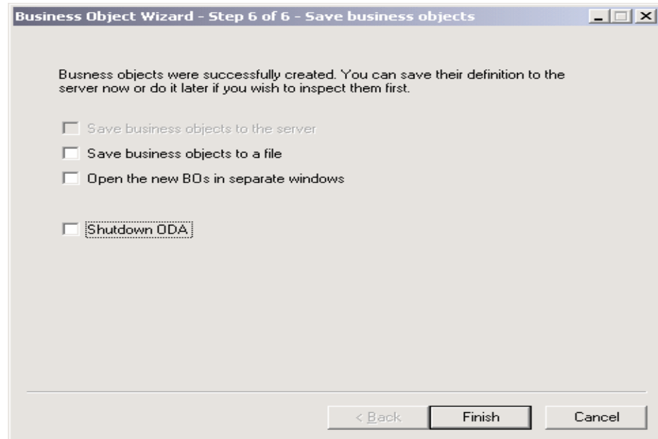
圖 68. 「儲存」視窗
