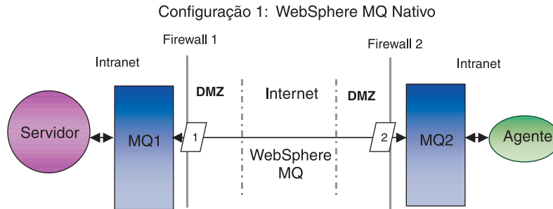
Figura 2. Configuração do WebSphere MQ Nativo
