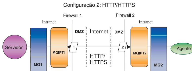
Figura 3. Configuração do HTTP/HTTPS
