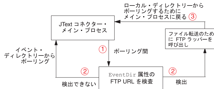
図 6. ローカルおよびリモートのイベント通知操作
