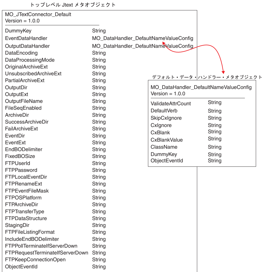
図 5. JText メタオブジェクトの階層構造
