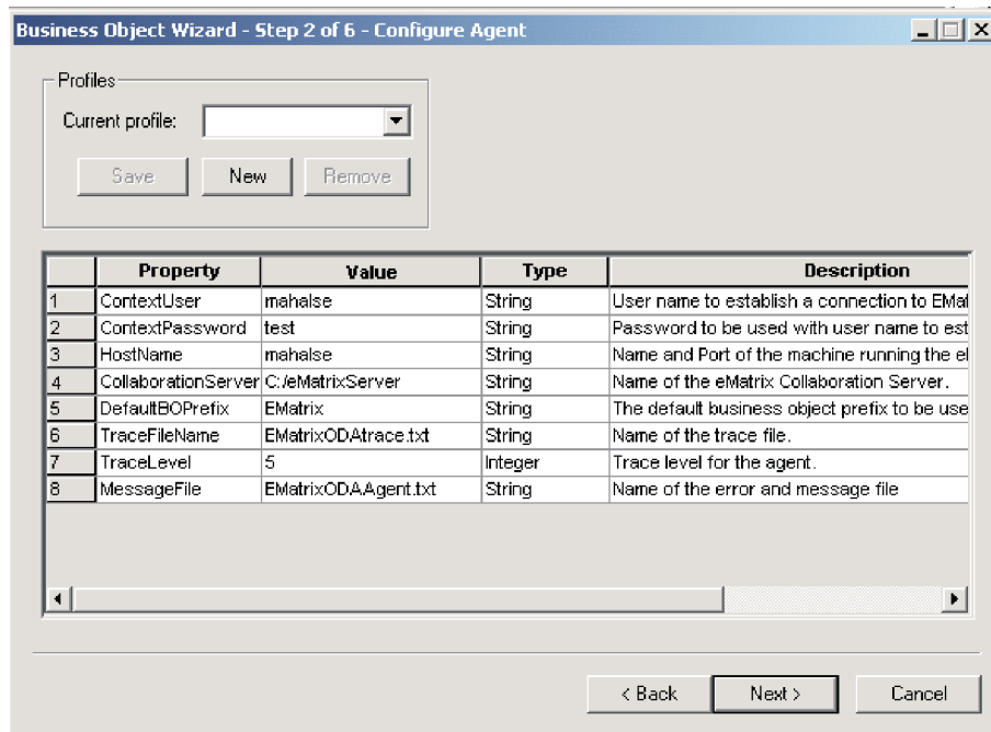
図9. 「エージェントの構成」画面
