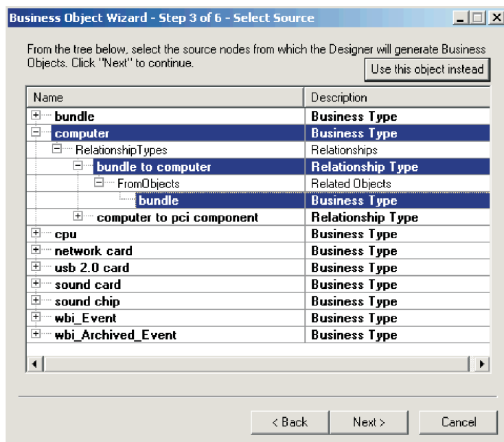
図 14. ビジネス・オブジェクト関係の選択
