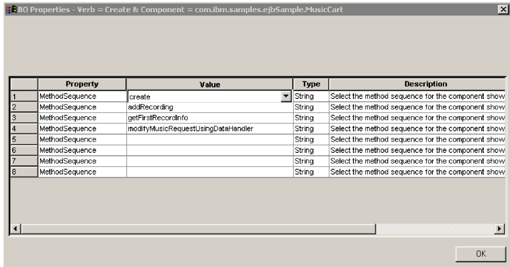
図 10. 動詞のメソッド・シーケンスの設定
