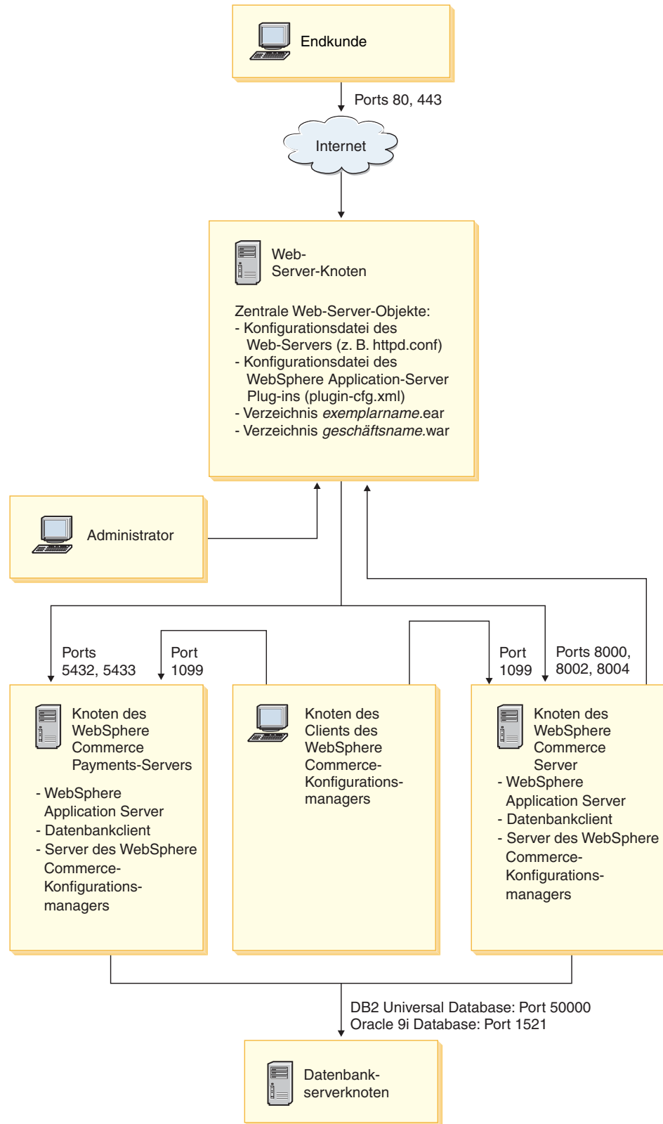
Abbildung 2. Angepasste Fünfknoteninstallation
