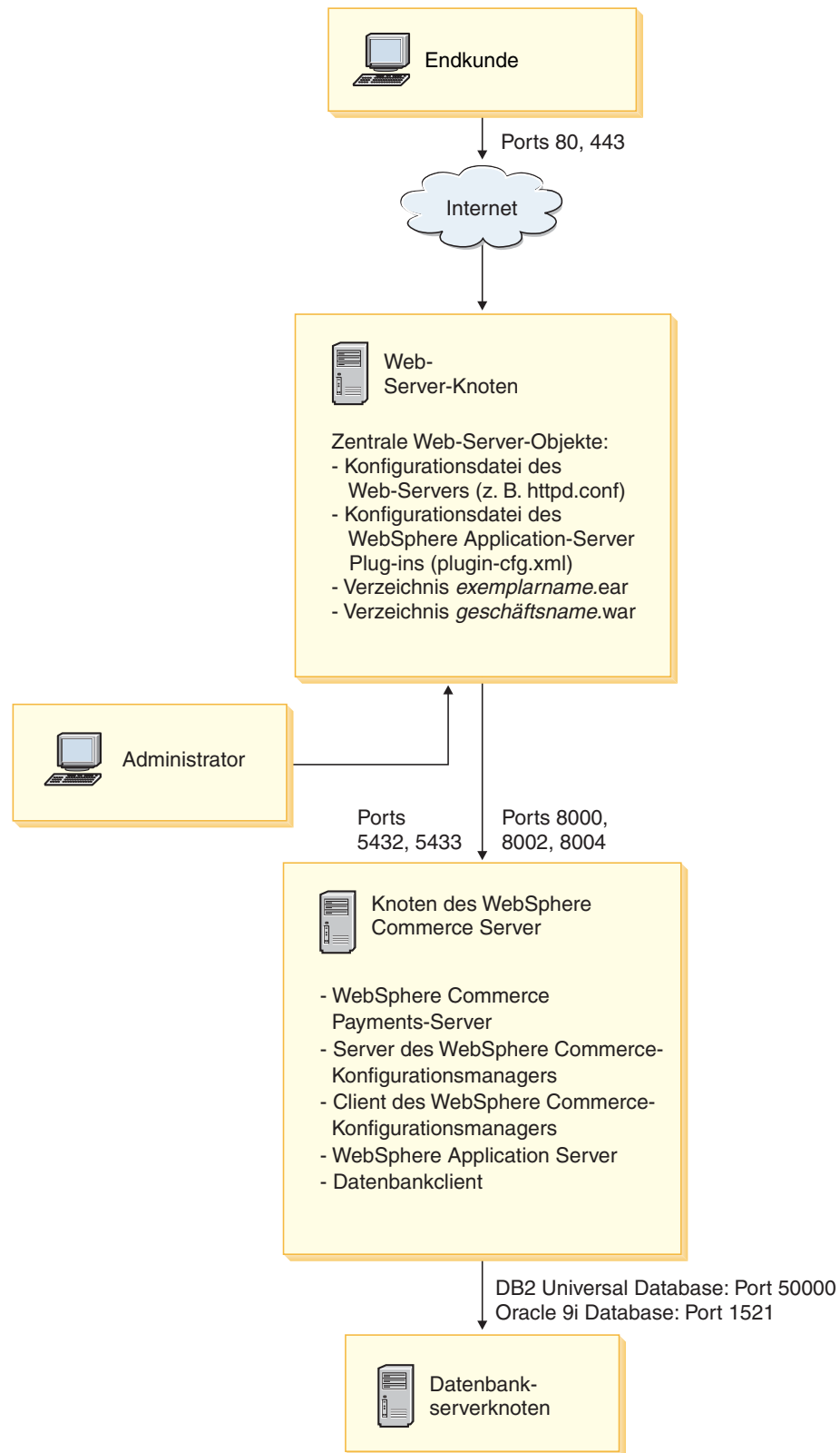
Abbildung 1. Dreiknoten-Standardinstallation
