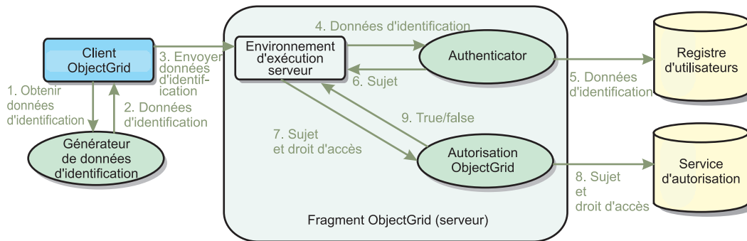
Figure 32. Flux d'authentification et d'autorisation du client
