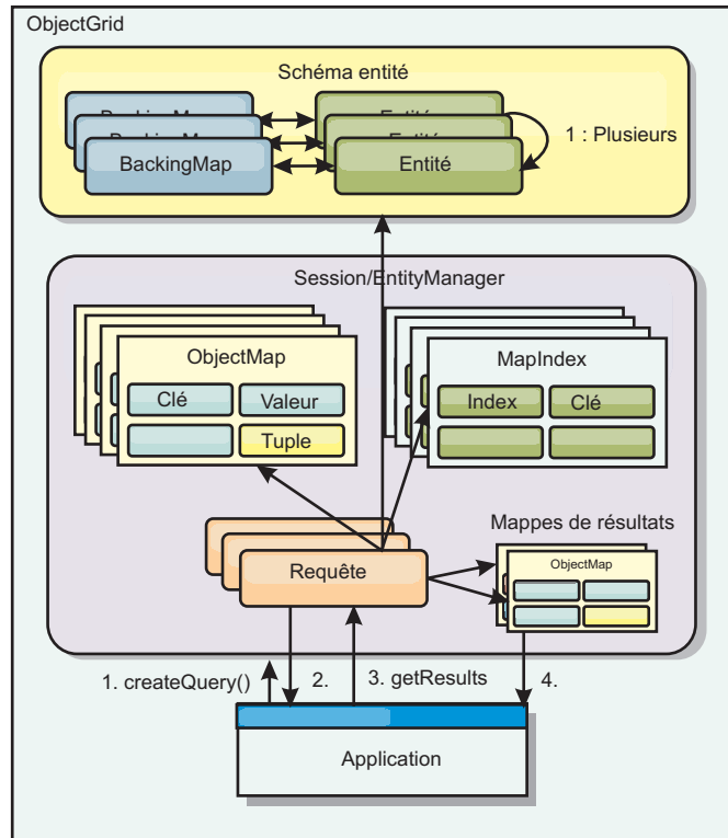
Figure 26. Interaction de la requête avec les mappes de l'objet ObjectGrid, définition du schéma d'entité et association de celui-ci à une mappe ObjectGrid.
