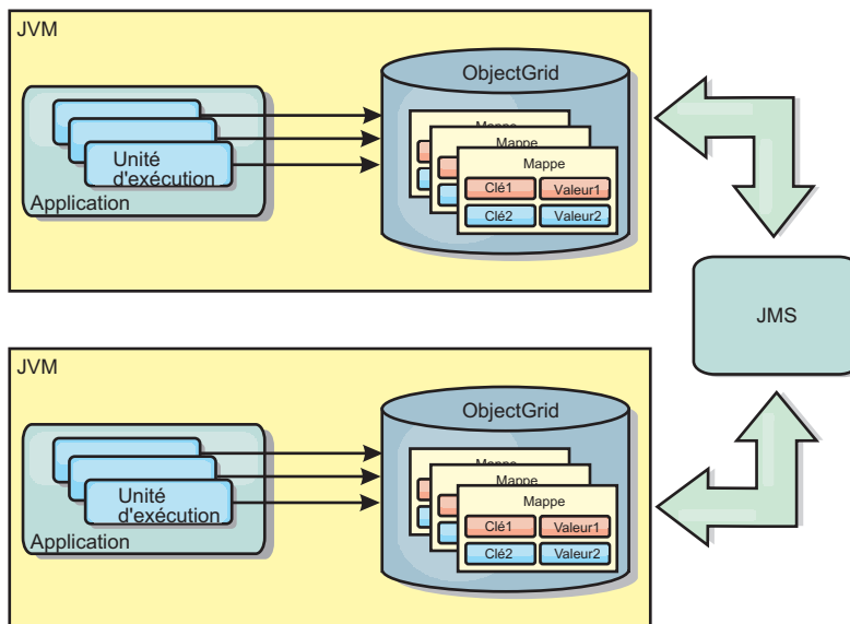
Figure 6. Cache répliqué sur des homologues avec des modifications qui sont propagées à l'aide de JMS
