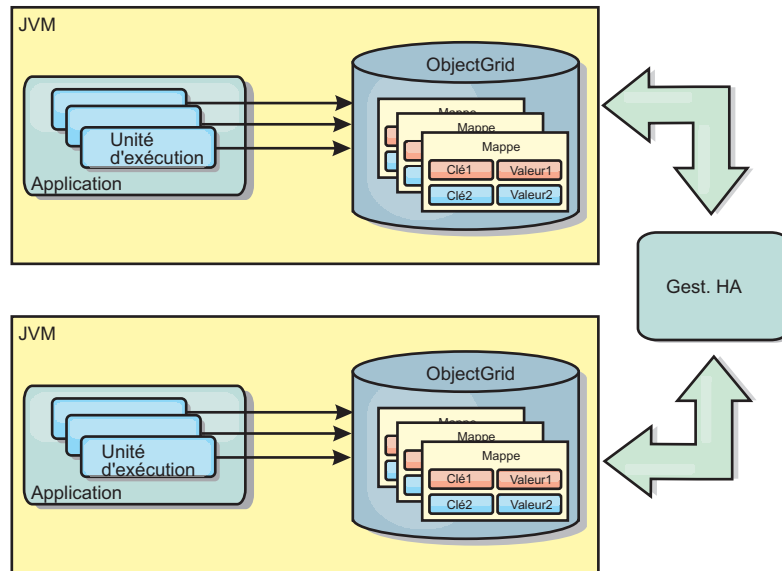
Figure 7. Cache répliqué sur des homologues avec des modifications qui sont propagées à l'aide du gestionnaire de haute disponibilité
