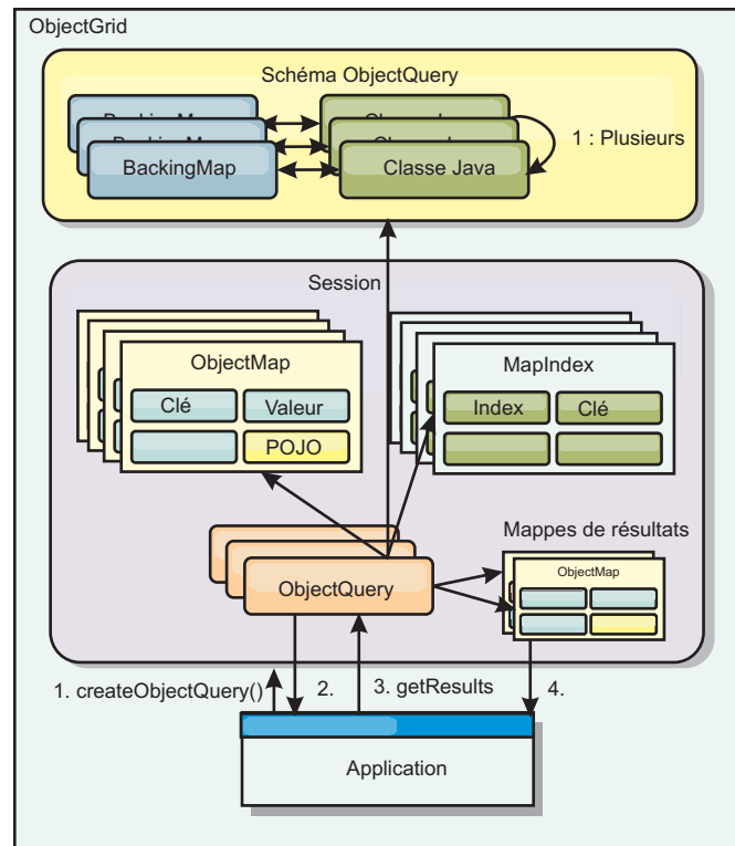
Figure 25. Interaction de la requête avec les mappes de l'objet ObjectGrid, définition d'un schéma pour les classes et association de celui-ci à une mappe ObjectGrid.
