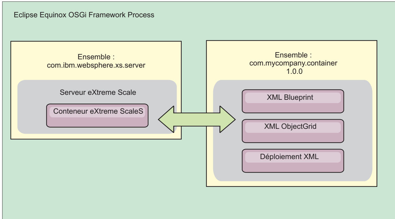
Figure 3. Processus Eclipse Equinox pour inclure toute la configuration et toutes les métadonnées dans un ensemble OSGi
