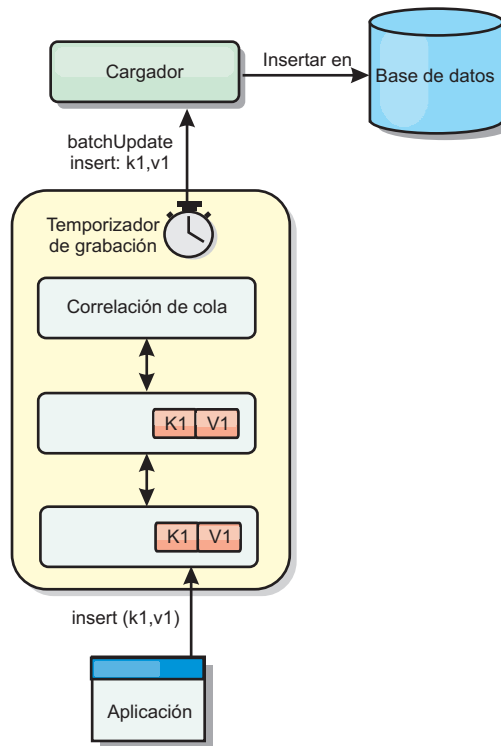
Figura 18. Almacenamiento en memoria caché de grabación diferida
