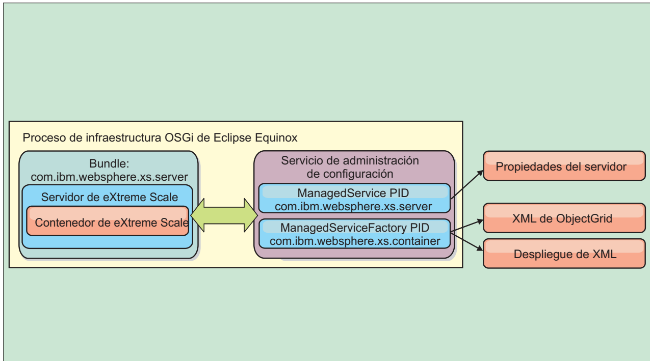
Figura 4. Proceso de Eclipse Equinox para especificar la configuración y los metadatos fuera de un paquete OSGi
