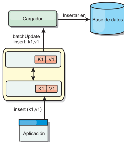
Figura 16. Almacenamiento en memoria caché de grabación directa
