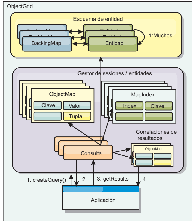
Figura 26. La interacción de la consulta con las correlaciones de objeto ObjectGrid y cómo se define y asocia el esquema de entidad con una correlación de ObjectGrid.
