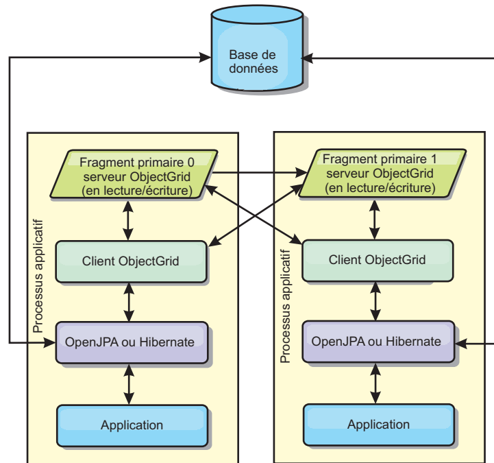
Figure 13. Topologie imbriquée et partitionnée JPA
