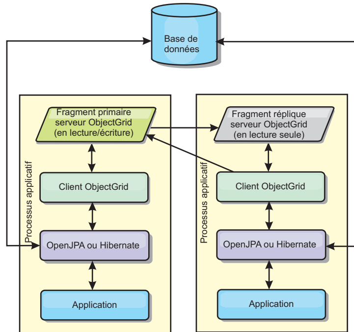
Figure 12. Topologie imbriquée JPA
