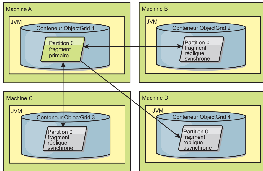
Figure 32. Exemple de positionnement d'une mappe ObjectGrid définie pour la partition partition0. La règle de déploiement comprend une valeur minSyncReplicas de 1, une valeur maxSyncReplicas de 2 et une valeur maxAsyncReplicas de 1.
