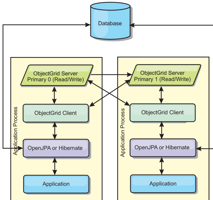
Figura 45. Topologia Particionada Integrada do JPA
