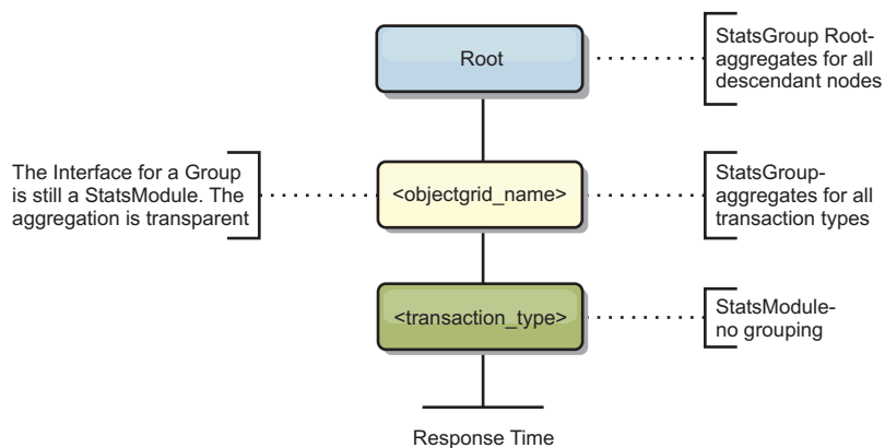
Figura 61. Estrutura do Módulo ObjectGridModule
