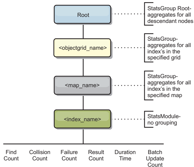
Figura 65. Estrutura do Módulo hashIndexModule
