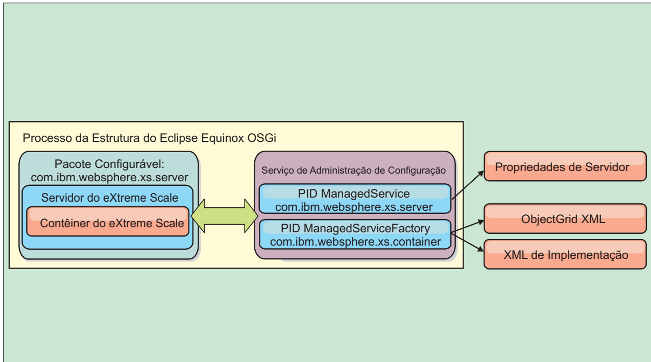
Figura 55. Processo do Eclipse Equinox para Especificar a Configuração e os Metadados Fora de um Pacote Configurável OSGi
