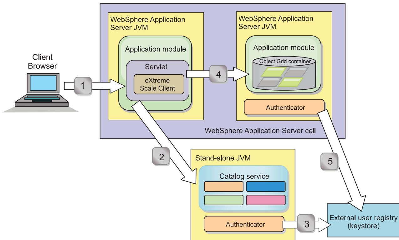
Figura 25. Fluxo de Autenticação
