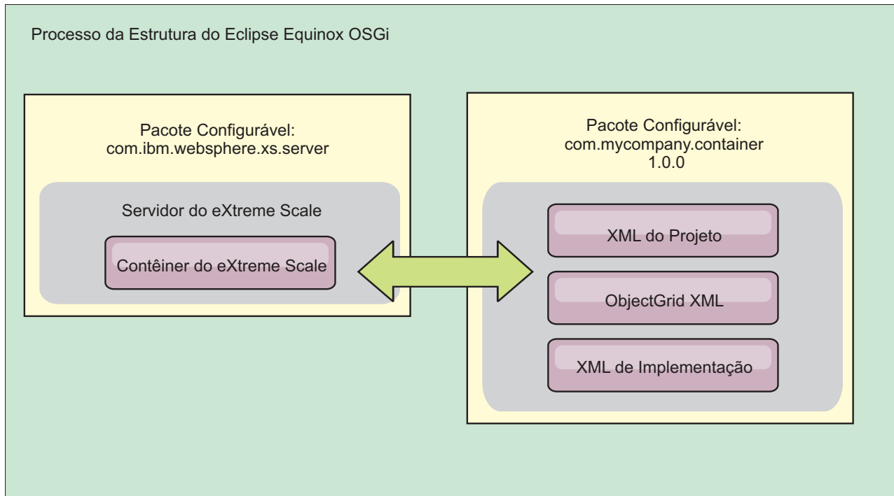
Figura 54. Processo do Eclipse Equinox para Incluir Toda a Configuração e Todos os Metadados em um Pacote Configurável OSGi
