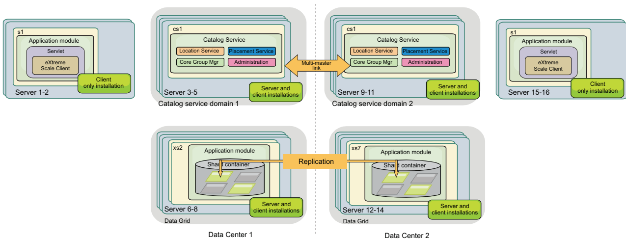
Figura 27. Topologia Independente com Dois Datacenters
