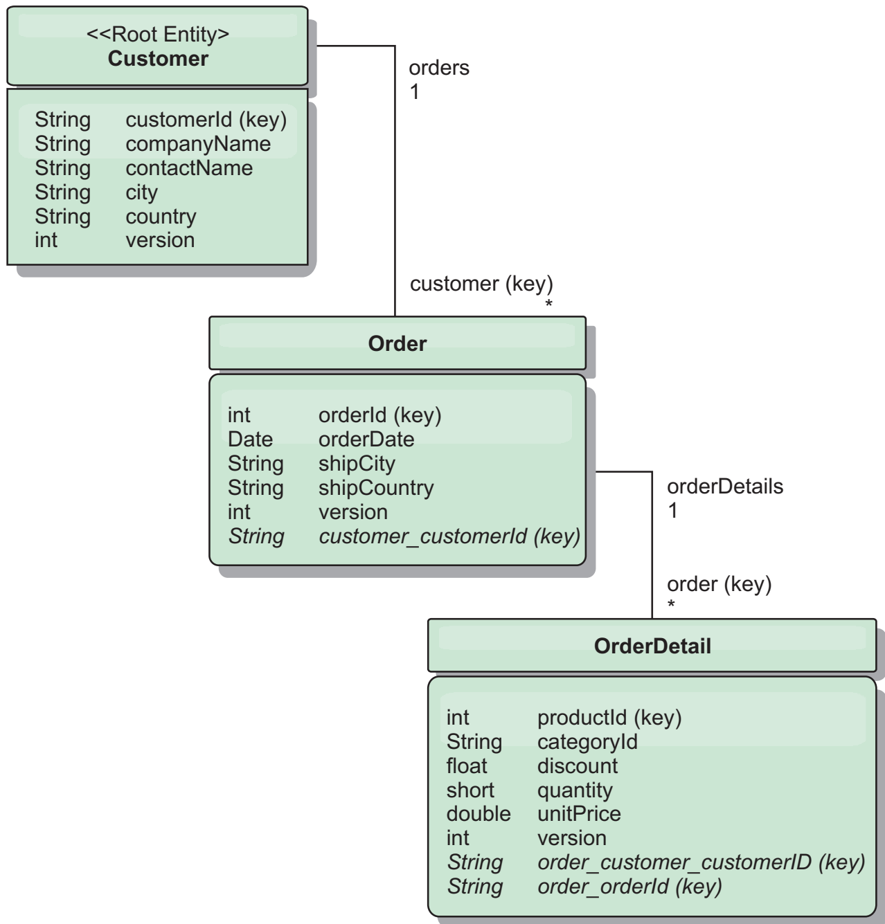
Figura 49. Diagrama do Esquema de Entidade Cliente e Ordem
