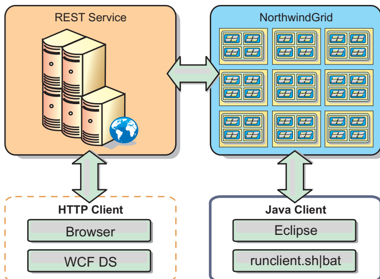
Figura 47. Topologia de Amostra de Introdução. Os clientes HTTP que usam o serviço de dados REST e os clientes Java podem acessar a mesma grade de dados.
