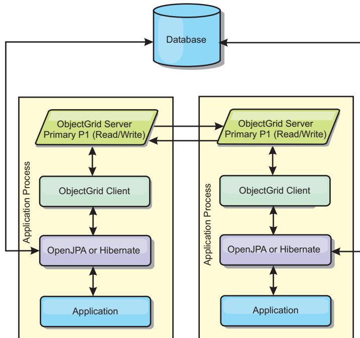
Figura 43. Topologia de Intradomínio do JPA
