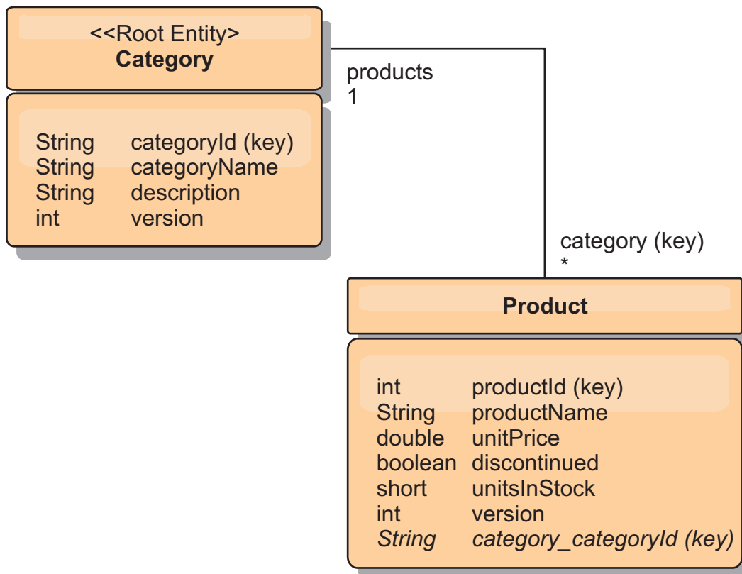
Figura 50. Diagrama do Esquema de Entidade Categoria e Produto
