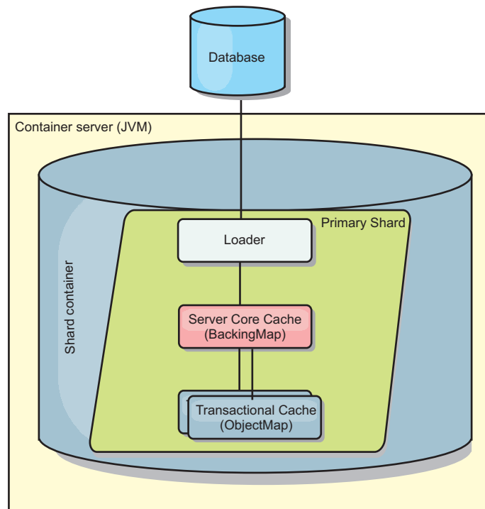
Figura 18. Plug-in do Utilitário de Carga
