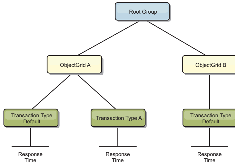
Figura 62. Exemplo da Estrutura do Módulo ObjectGridModule
