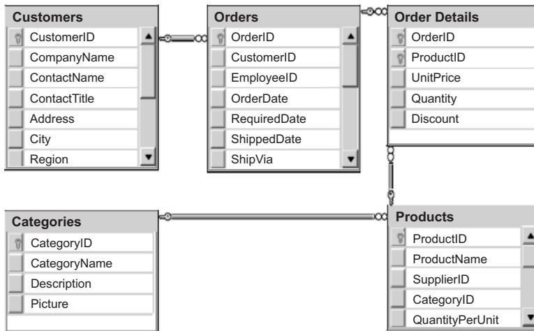
Figura 48. Diagrama do Esquema da Amostra Northwind do Microsoft SQL Server
