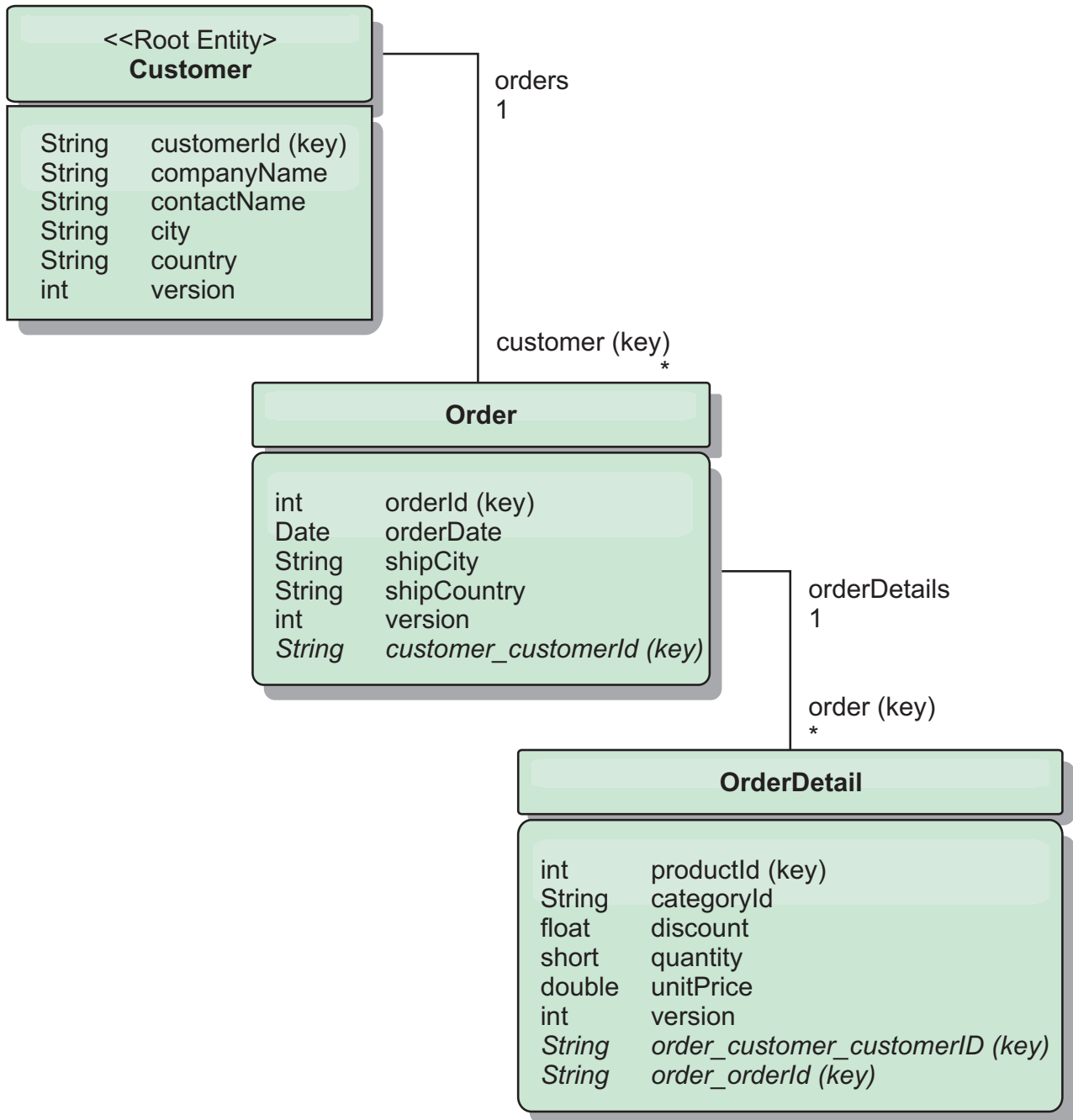
Figura 51. Diagrama do Esquema de Entidade Cliente e Ordem
