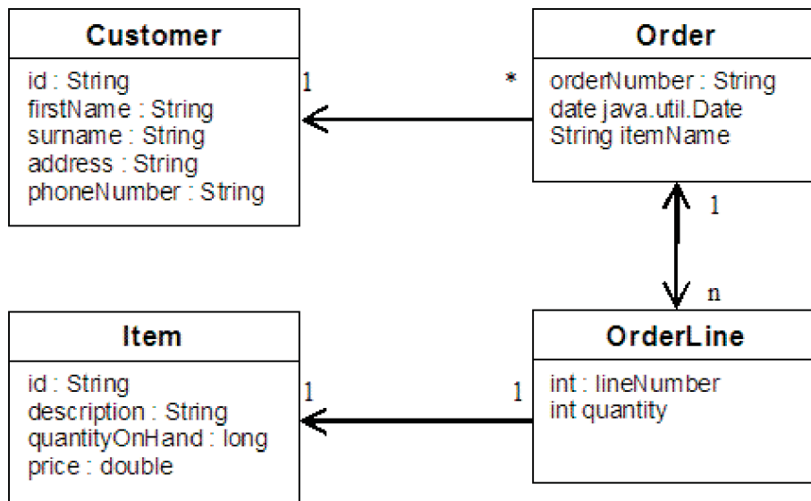
Figura 21. Esquema de Ordem . Um Esquema de Ordem tem um relacionamento um-para-um com o Cliente e um relacionamento um-para-muitos com o OrderLine. O mapa OrderLine tem um relacionamento um-para-um com o Item e inclui a quantidade pedida.
