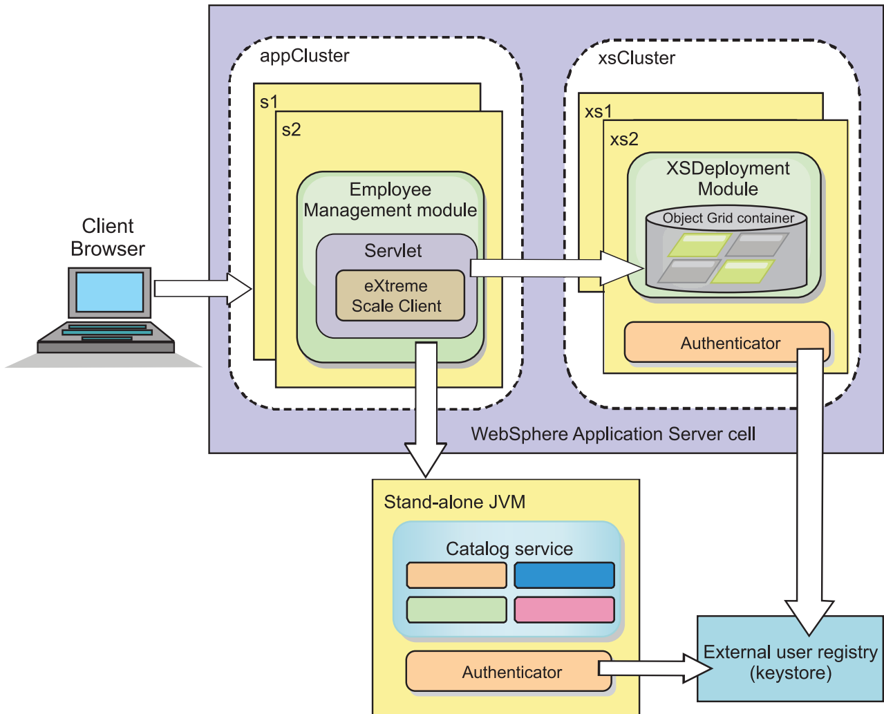
Figura 24. Topologia do Tutorial
