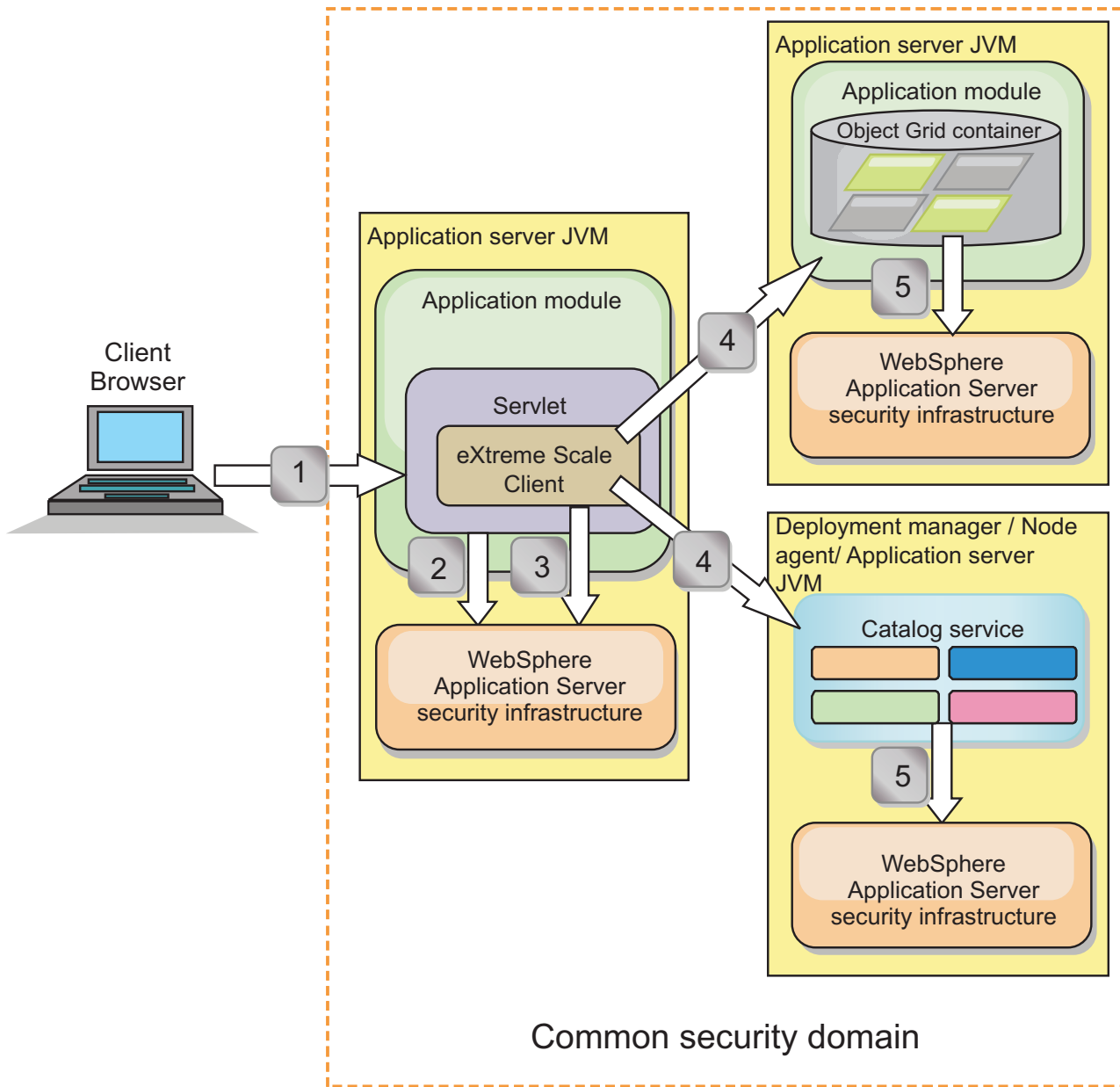
Figura 71. Fluxo de Autenticação para Servidores Dentro do Mesmo Domínio de Segurança
