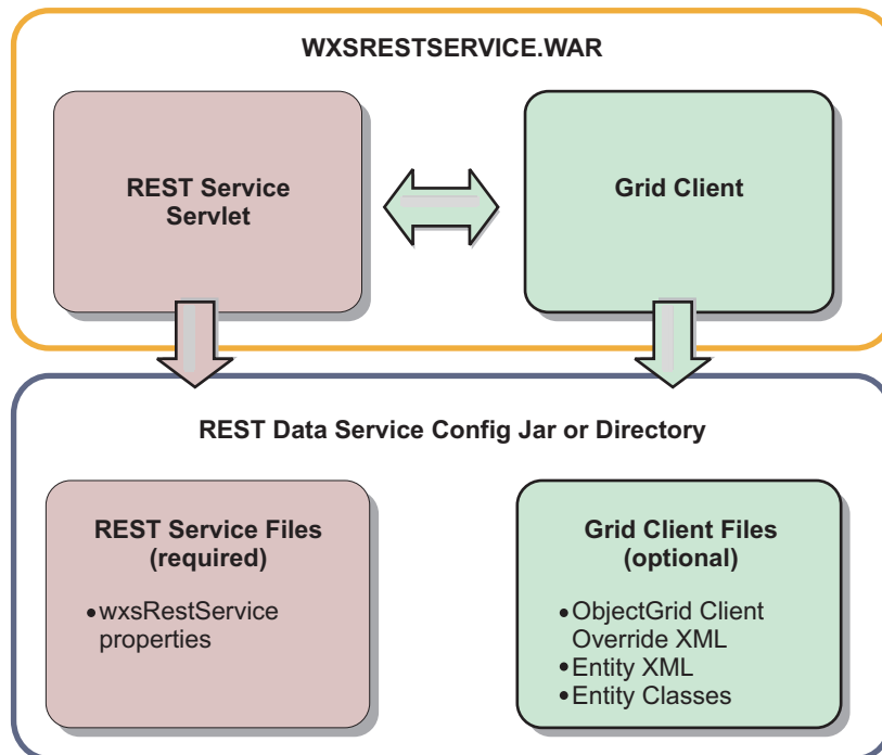
Figura 30. Arquivos do Serviço de Dados REST do WebSphere eXtreme Scale
