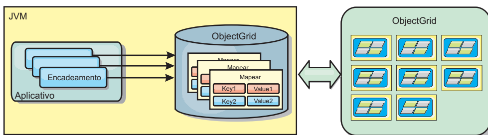
Figura 8. Cache Local
