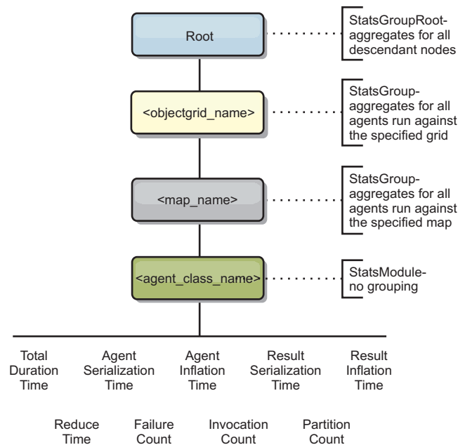
Figura 67. Estrutura agentManagerModule
