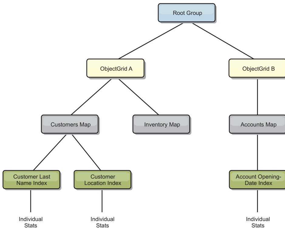
Figura 66. Exemplo da Estrutura do Módulo hashIndexModule
