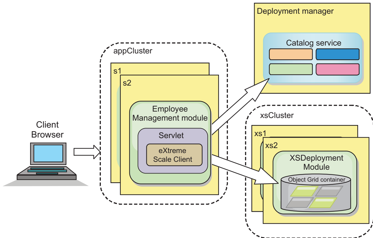
Figura 23. Topologia do Tutorial
