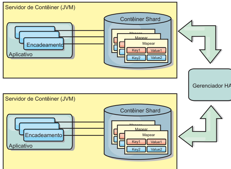
Figura 5. Cache Replicado pelo Peer com Alterações que são Propagadas com o Gerenciador de Alta Disponibilidade
