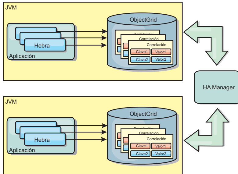
Figura 5. La memoria caché duplicada por un igual con los cambios propagados con el High Availability Manager.
