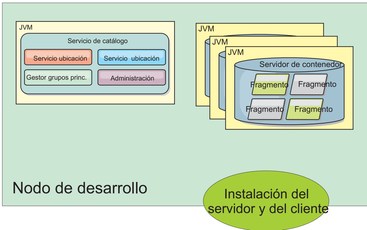
Figura 26. Nodo de desarrollo
