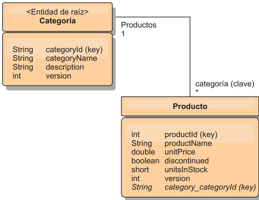
Figura 50. Diagrama del esquema de entidades Category y Product
