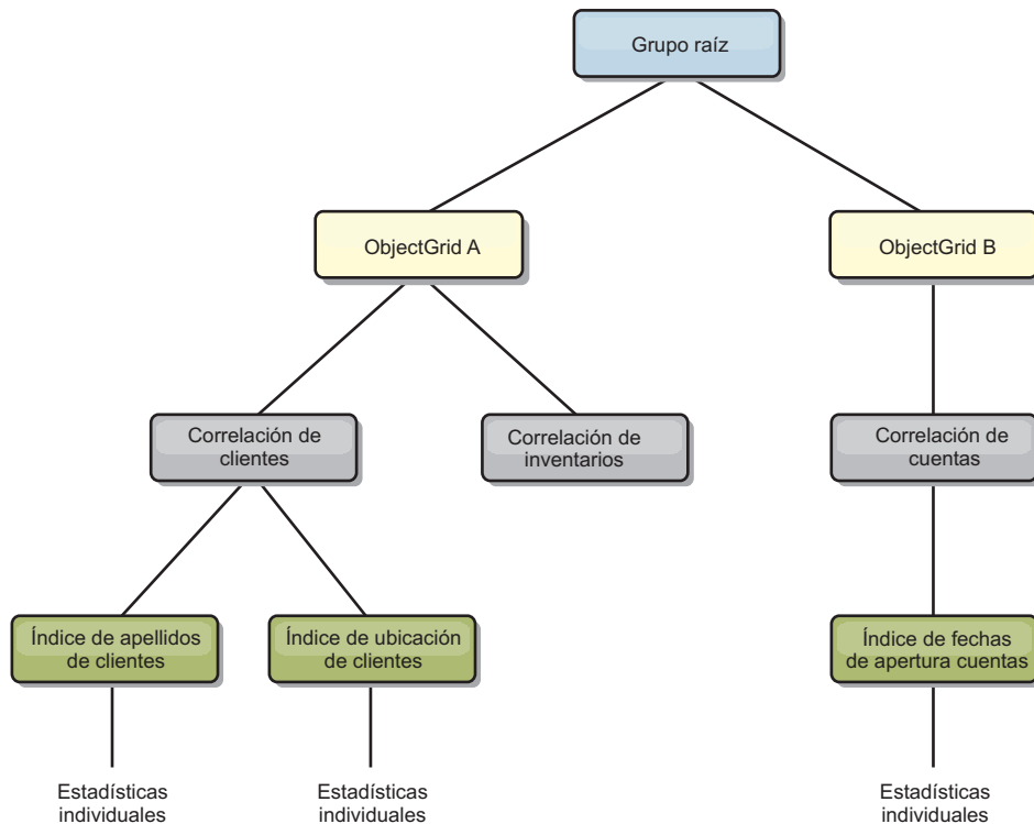
Figura 66. Ejemplo de estructura del módulo hashIndexModule
