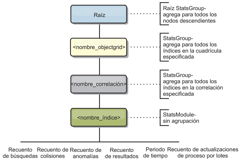
Figura 65. Estructura del módulo hashIndexModule
