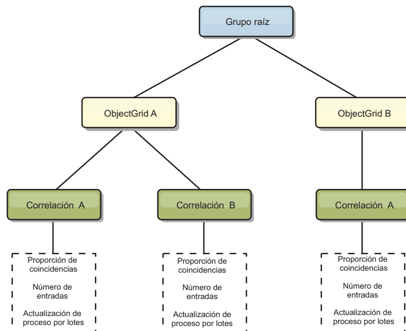
Figura 64. Ejemplo de la estructura del módulo mapModule
