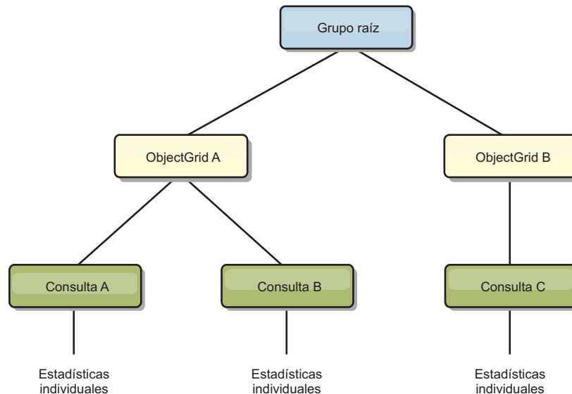
Figura 70. Ejemplo de la estructura de queryModule de QueryStats.jpg
