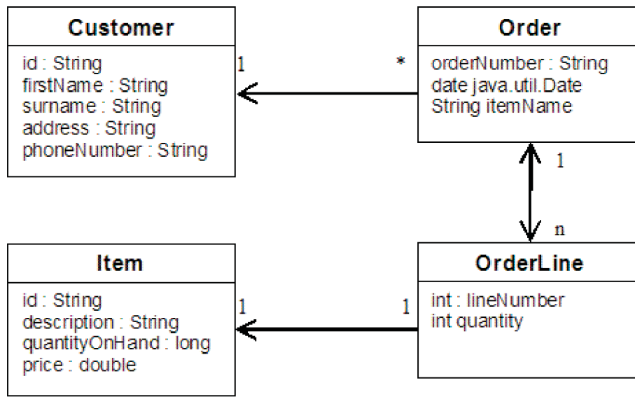
Figura 22. Esquema de entidades Order. Una entidad Order tiene una referencia a un cliente y cero o más OrderLines. Cada entidad OrderLine tiene una referencia a un sólo artículo e incluye la cantidad solicitada.
