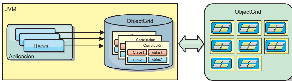
Figura 8. Memoria caché cercana
