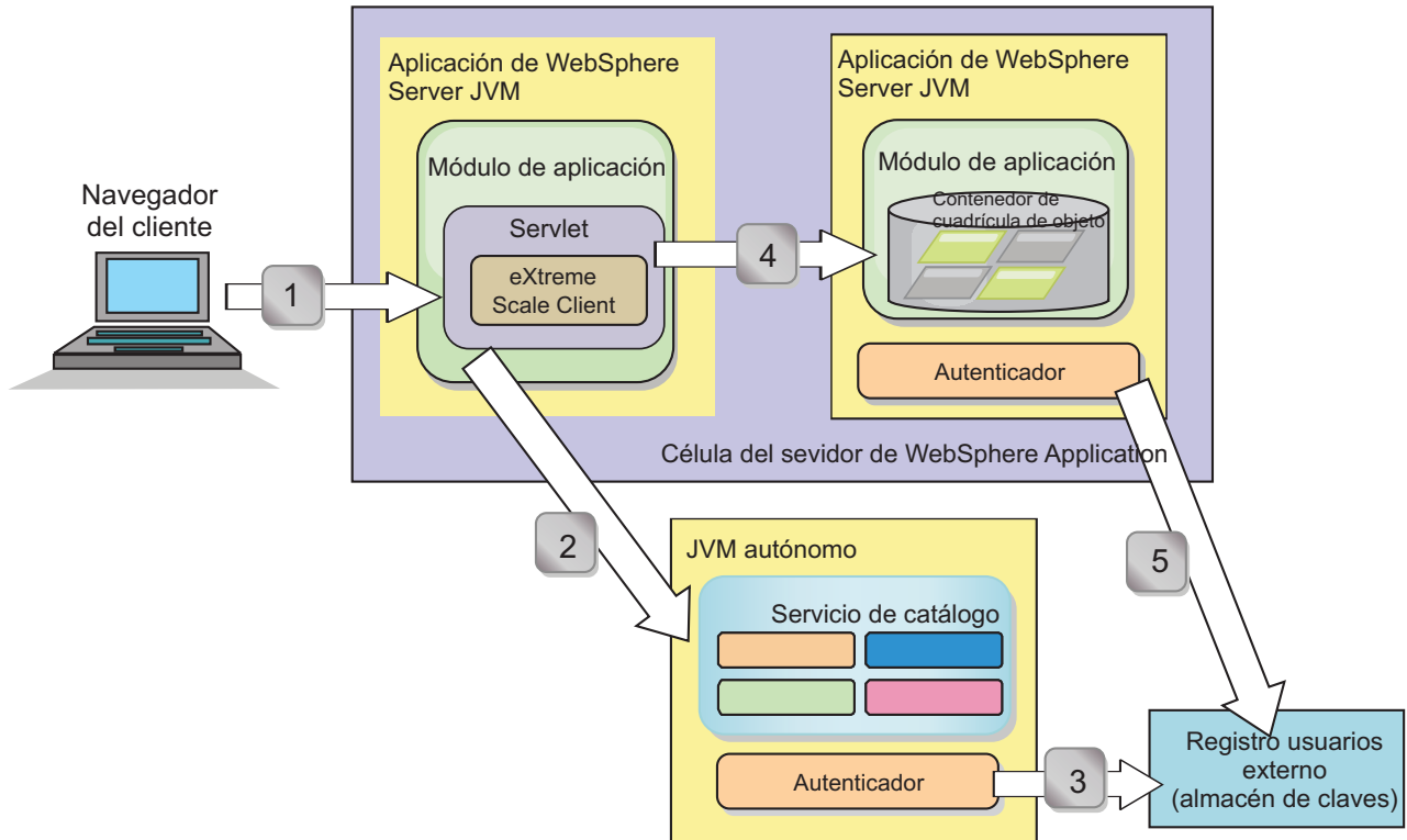
Figura 25. Flujo de autenticación
