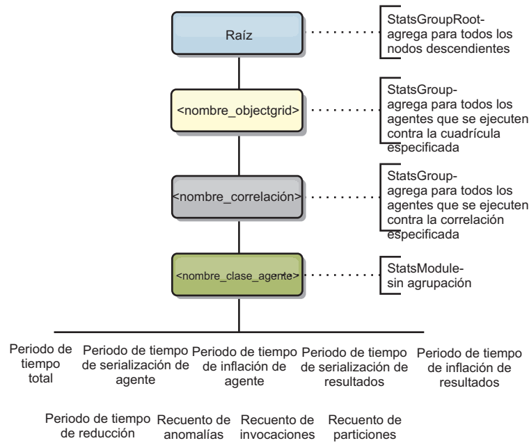
Figura 67. Estructura de agentManagerModule
