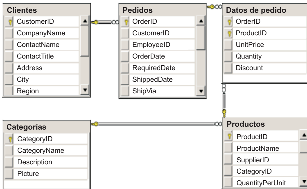
Figura 48. Diagrama del esquema de ejemplo Northwind de Microsoft SQL Server
