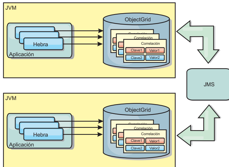
Figura 4. La memoria caché duplicada por un igual con los cambios que se propagan con JMS
