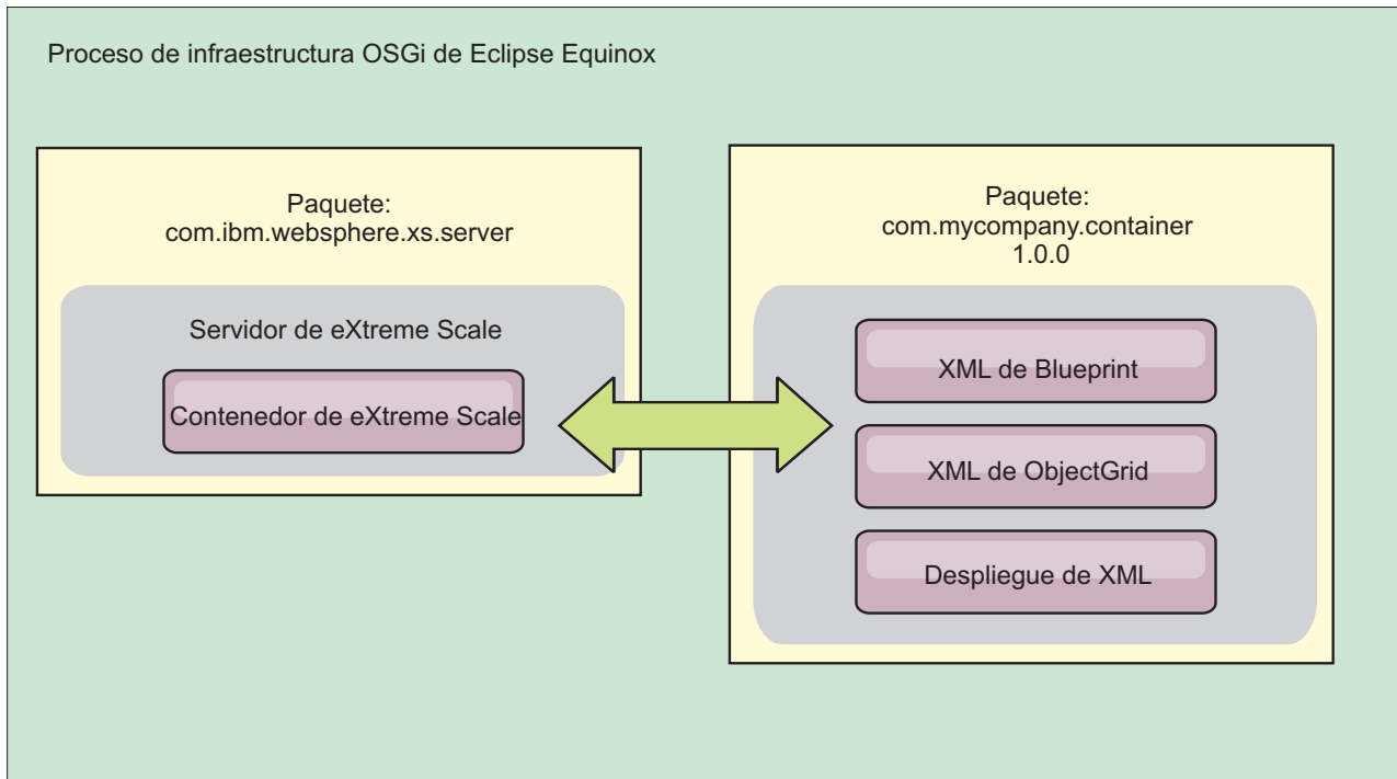
Figura 54. Proceso de Eclipse Equinox para incluir toda la configuración y los metadatos en un paquete OSGi
