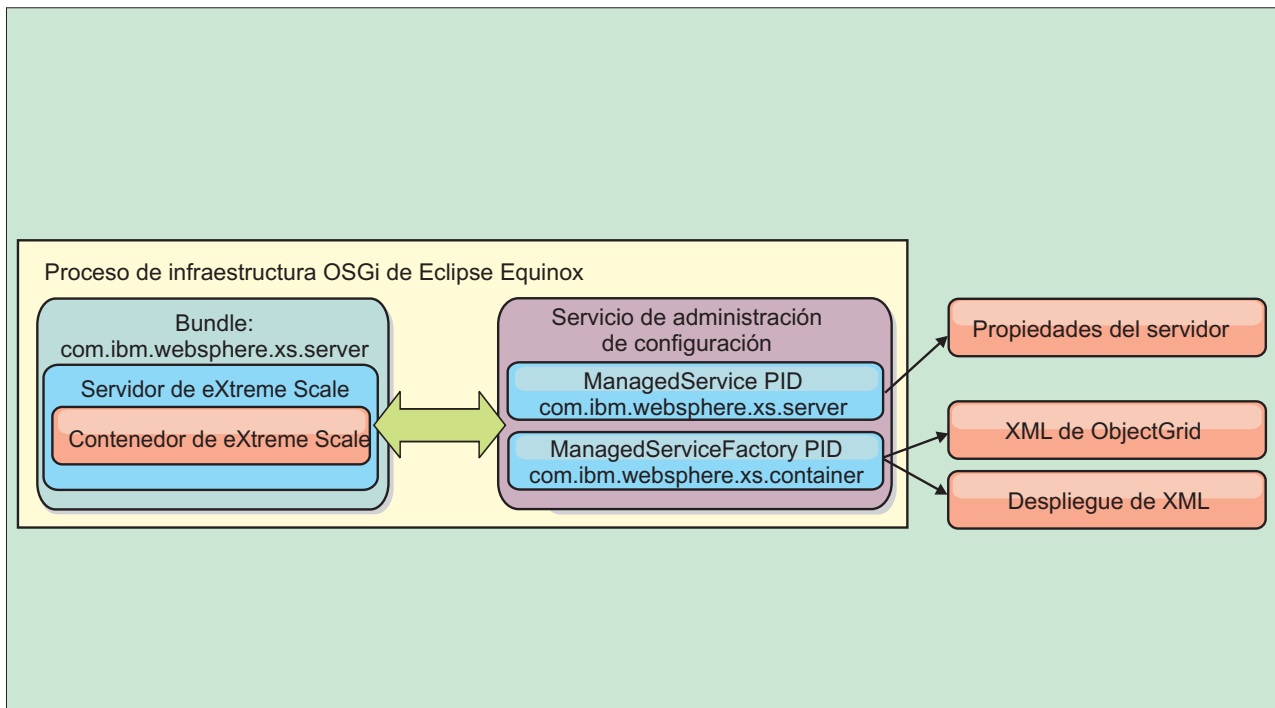
Figura 55. Proceso de Eclipse Equinox para especificar la configuración y los metadatos fuera de un paquete OSGi
