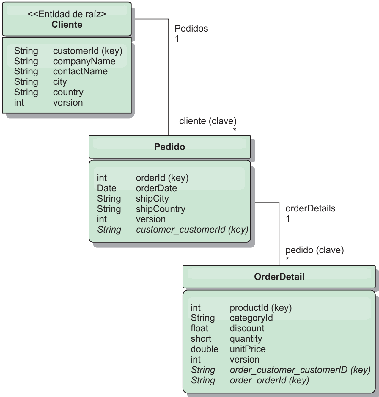
Figura 51. Diagrama del esquema de entidades Customer y Order
