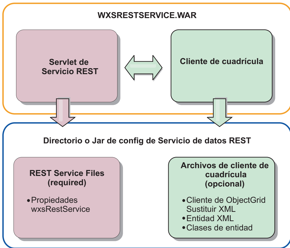
Figura 30. Archivos del servicio de datos REST de WebSphere eXtreme Scale
