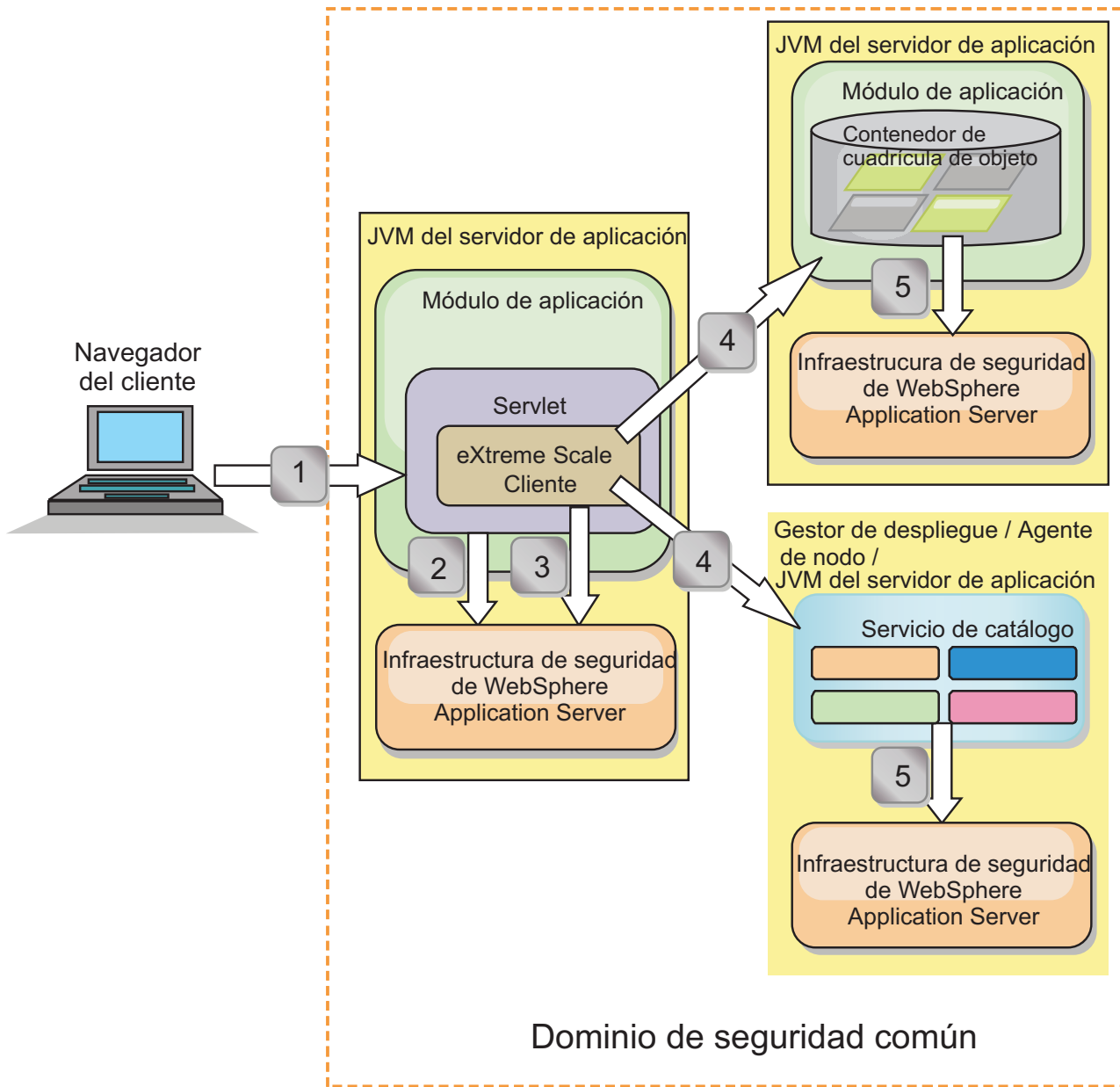
Figura 71. Flujo de autenticación para servidores en el mismo dominio de seguridad
