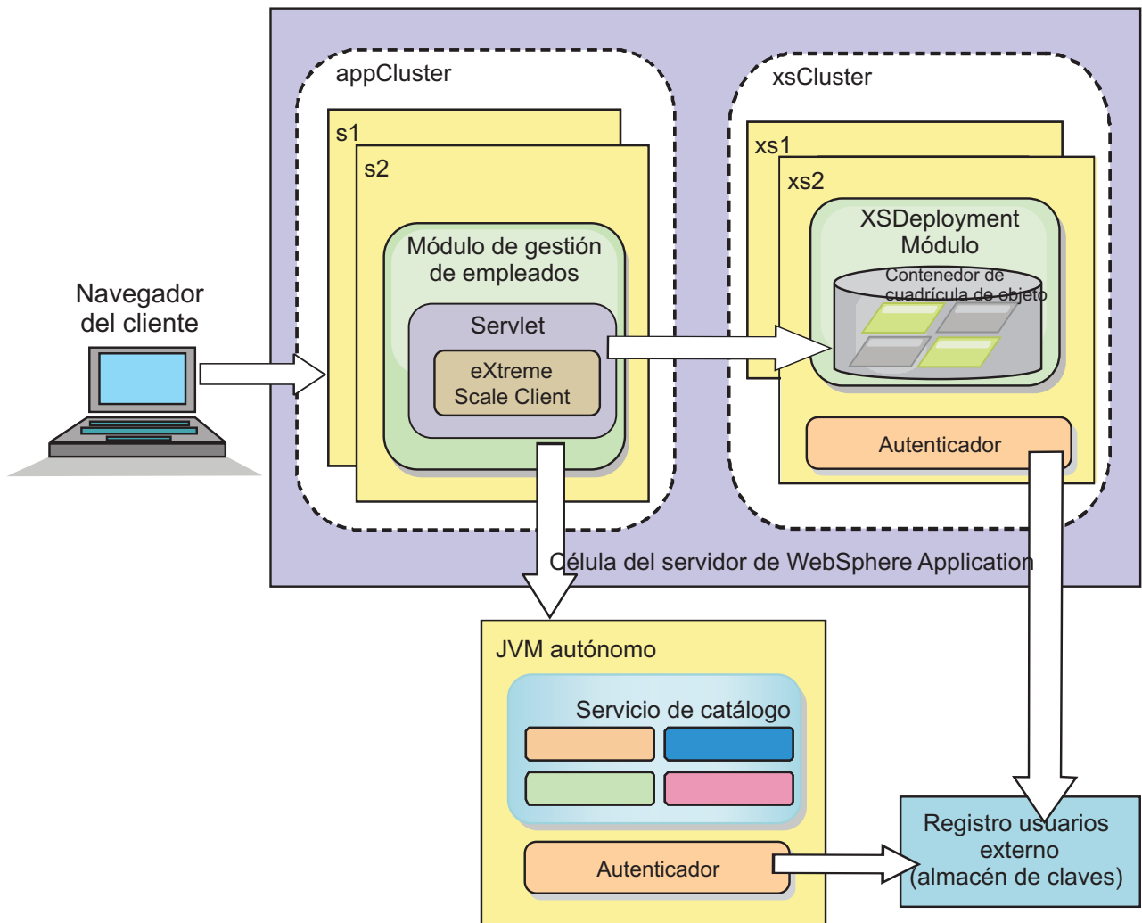
Figura 24. Topología de la guía de aprendizaje
