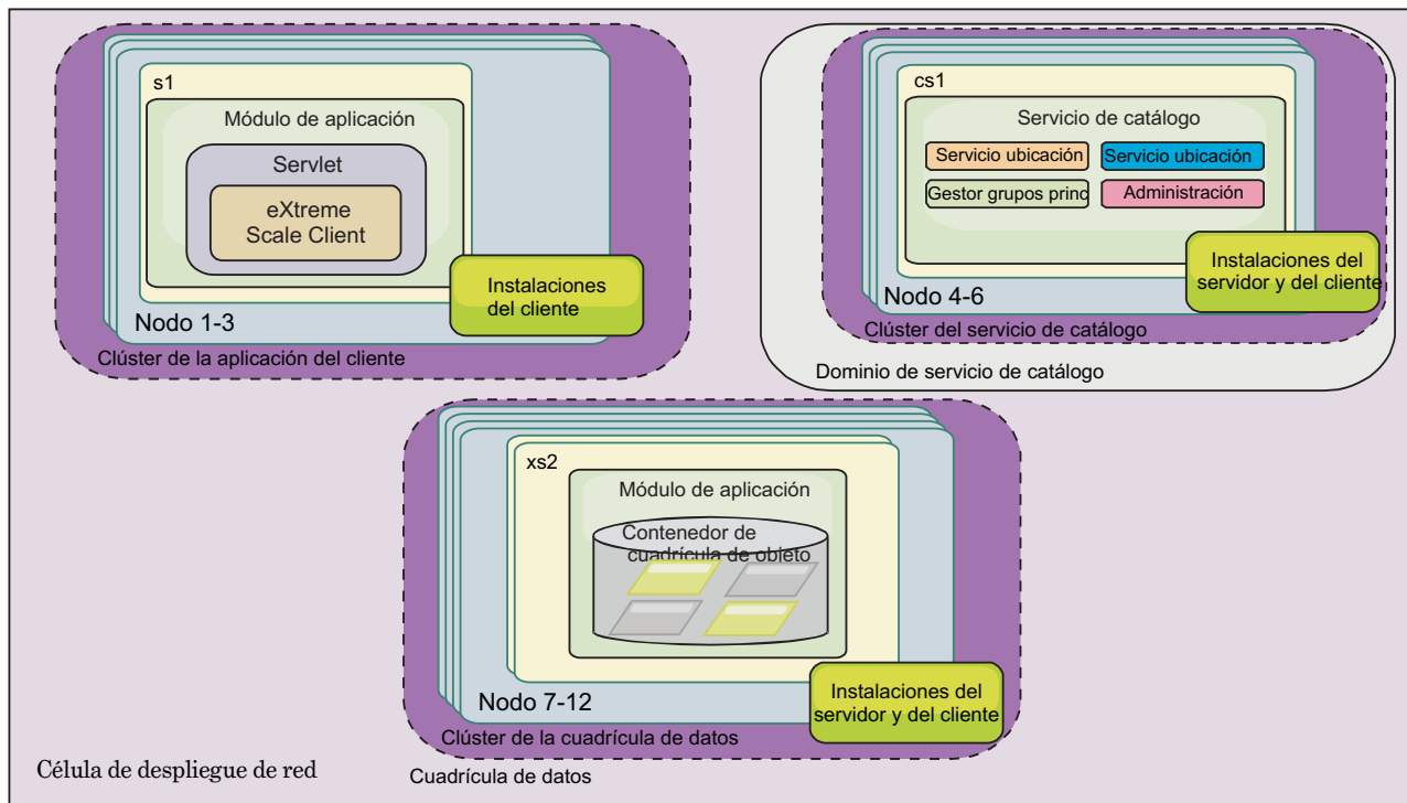
Figura 28. Ejemplo de topología de WebSphere Application Server
