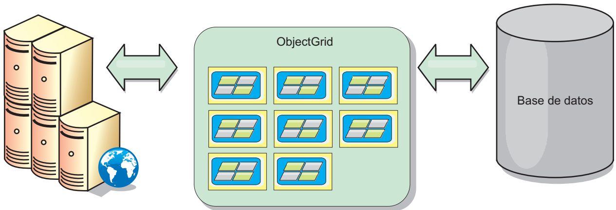
Figura 9. ObjectGrid como un almacenamiento intermedio de base de datos
