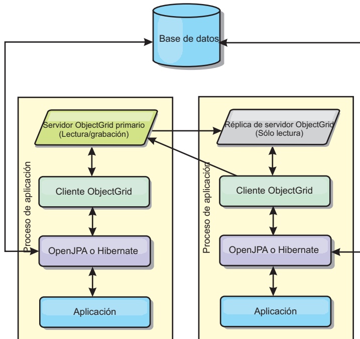
Figura 44. Topología incorporada JPA
