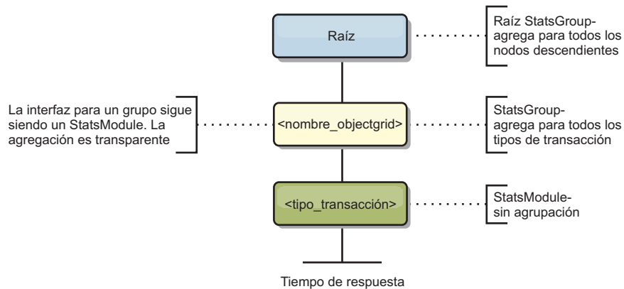
Figura 61. Estructura del módulo ObjectGridModule
