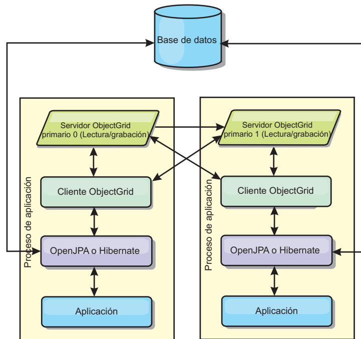
Figura 45. Topología incorporada con particiones JPA
