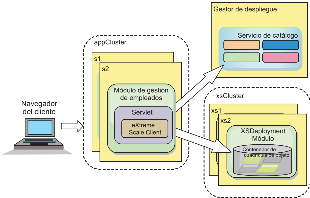
Figura 23. Topología de la guía de aprendizaje
