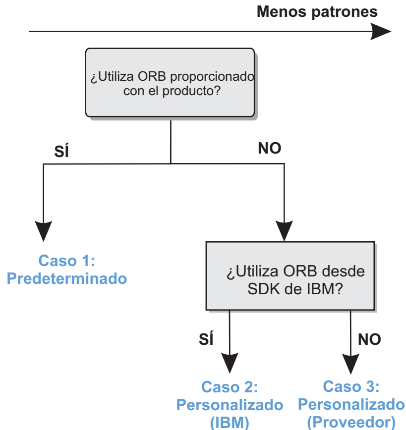
Figura 38. Selección de un ORB
