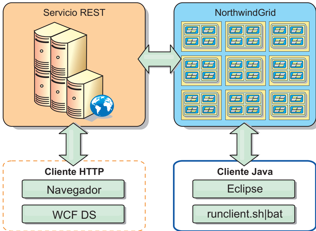
Figura 47. Iniciación a la topología de ejemplo. Los clientes HTTP que utilizan el servicio de datos REST y los clientes Java pueden acceder a la misma cuadrícula de datos.
