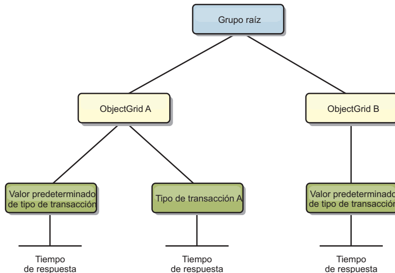
Figura 62. Ejemplo de estructura del módulo ObjectGridModule
