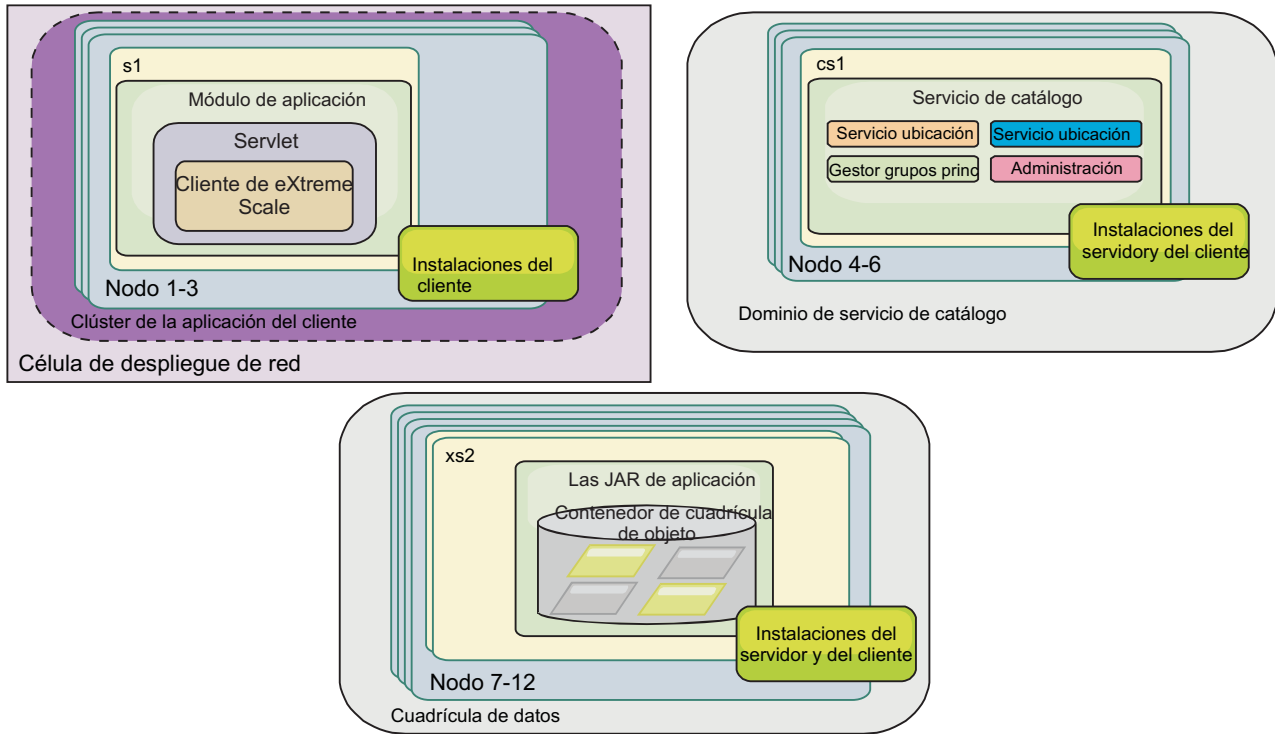
Figura 29. Ejemplo de topología mixta
