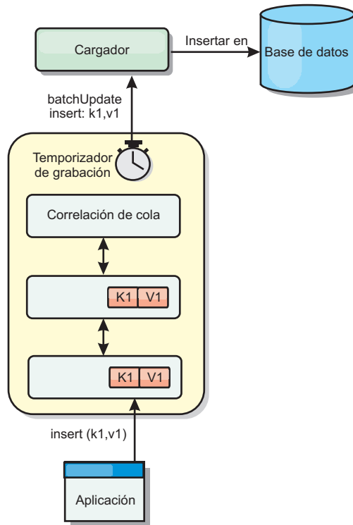
Figura 15. Almacenamiento en memoria caché de grabación diferida
