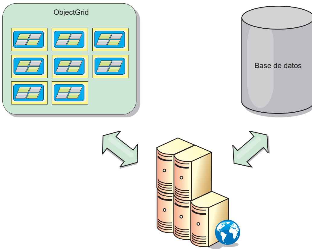
Figura 10. ObjectGrid como una memoria caché secundaria
