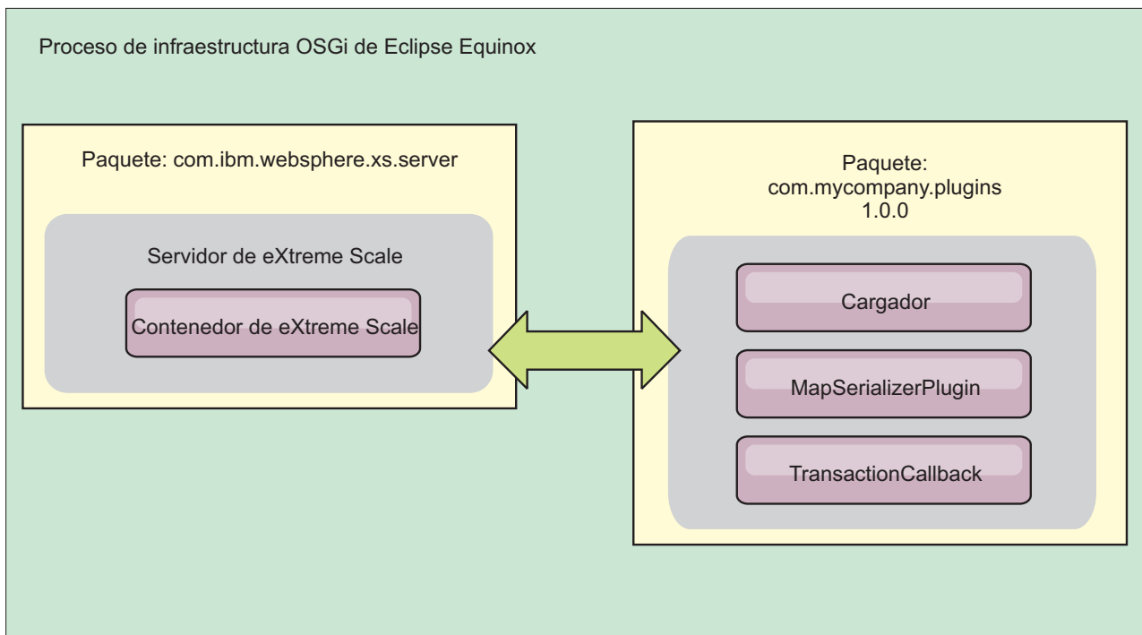
Figura 52. Proceso de Eclipse Equinox para instalar e iniciar paquetes OSGi con plug-ins de eXtreme Scale
