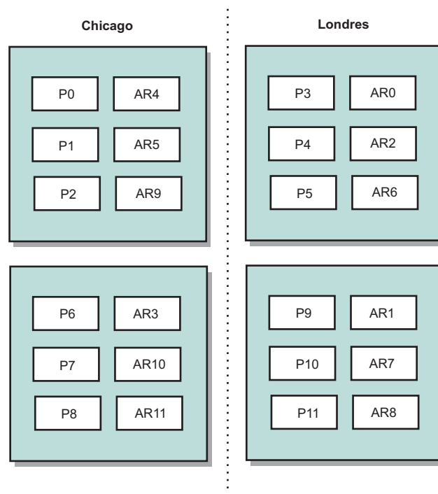
Figura 33. Primarios y réplicas en las zonas
