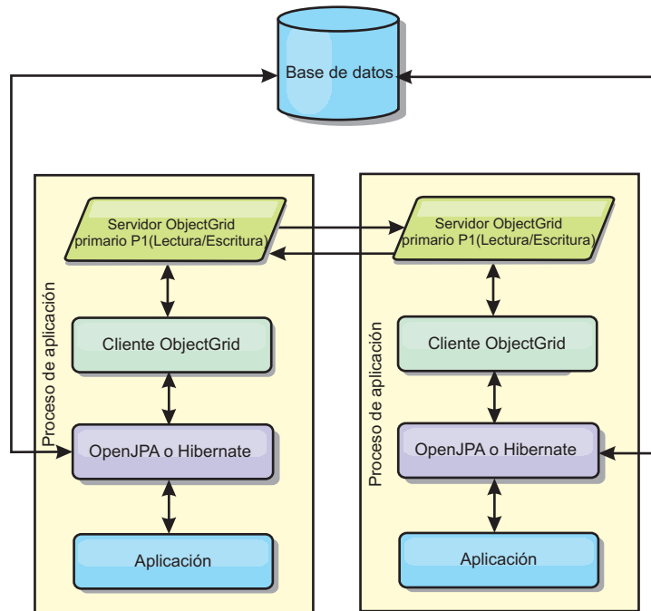
Figura 43. Topología interno del dominio JPA
