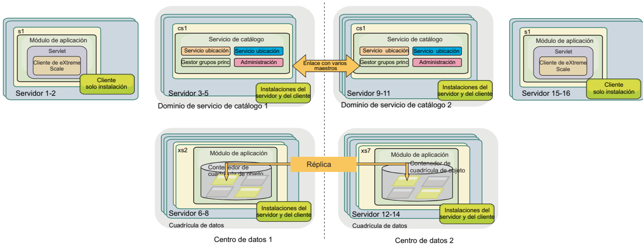
Figura 27. Topología autónoma con dos centros de datos
