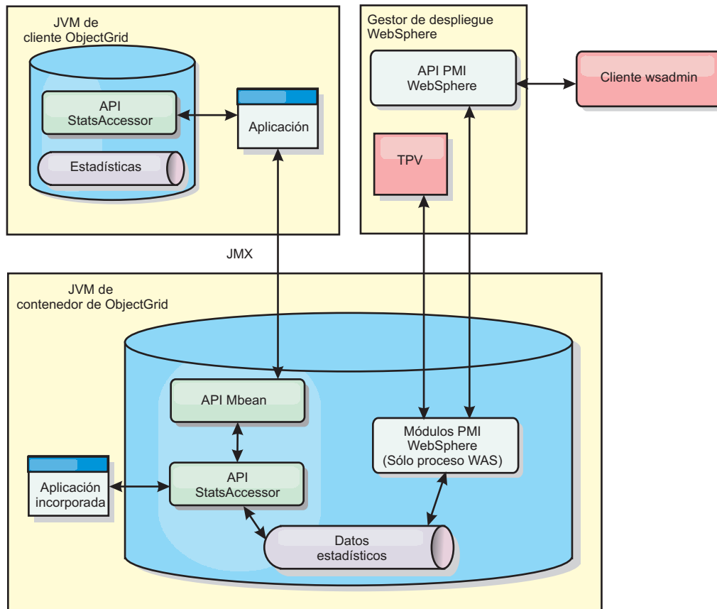
Figura 60. Visión general de MBean
