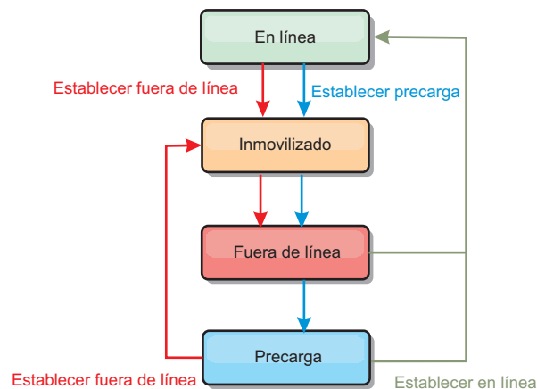
Figura 53. Estados de disponibilidad de una instancia de ObjectGrid
