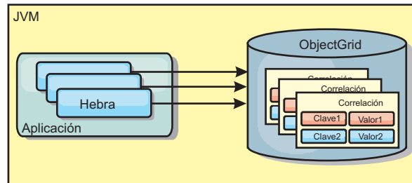
Figura 3. Escenario de memoria caché en memoria local
