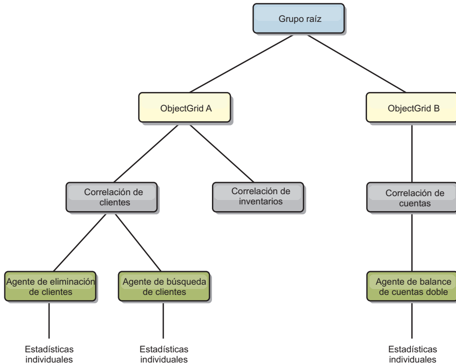
Figura 68. Ejemplo de la estructura de agentManagerModule
