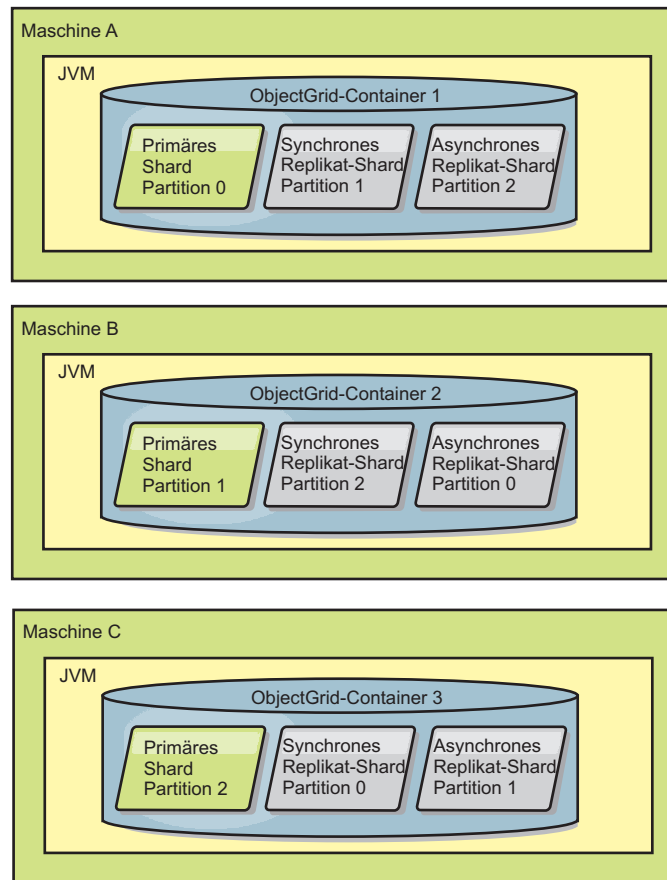
Abbildung 31. Verteilung eines ObjectGrid-MapSets über eine Implementierungsrichtlinie mit 3 Partitionen mit einem minSyncReplicas -Wert von 1, einem maxSyncReplicas -Wert von 1 und einem maxAsyncReplicas -Wert von 1
