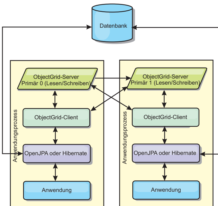
Abbildung 13. Integrierte, partitionierte JPA-Topologie
