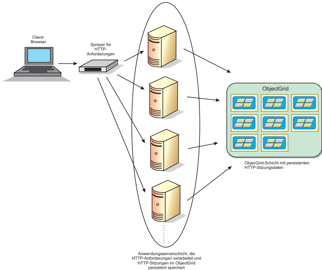
Abbildung 15. Topologie für das HTTP-Sitzungsmanagement mit einer fernen Containerkonfiguration
