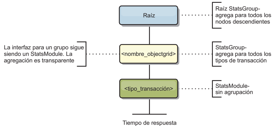
Figura 58. Estructura del módulo ObjectGridModule
