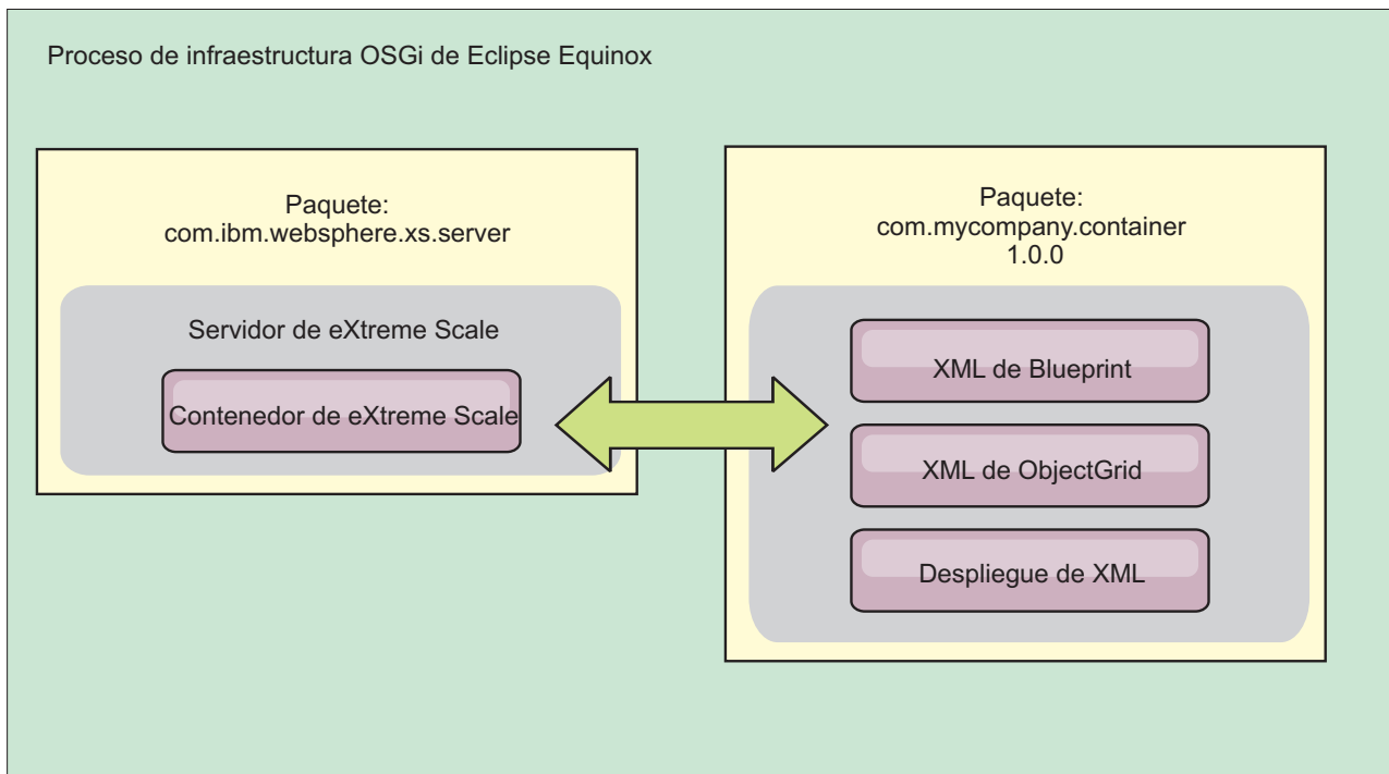
Figura 51. Proceso de Eclipse Equinox para incluir toda la configuración y los metadatos en un paquete OSGi
