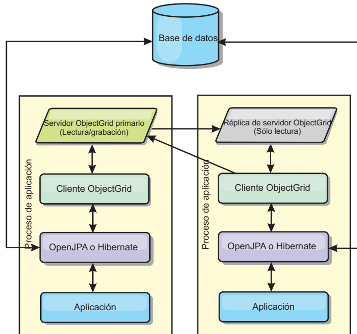
Figura 41. Topología incorporada JPA
