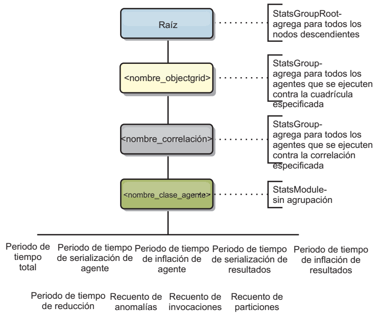
Figura 64. Estructura de agentManagerModule
