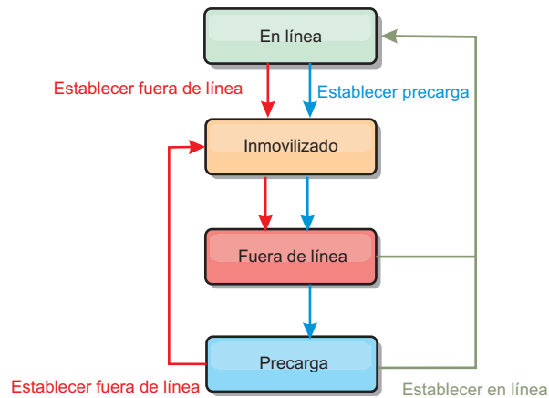
Figura 50. Estados de disponibilidad de una instancia de ObjectGrid
