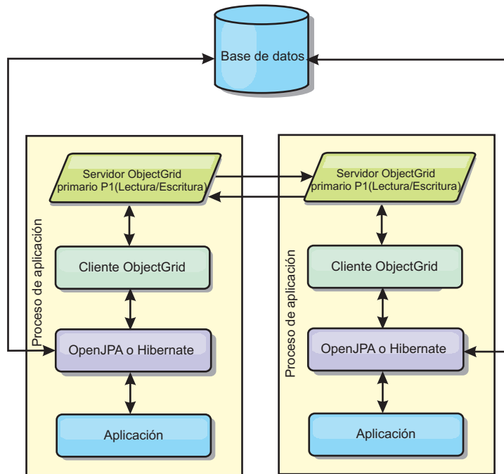
Figura 40. Topología interno del dominio JPA
