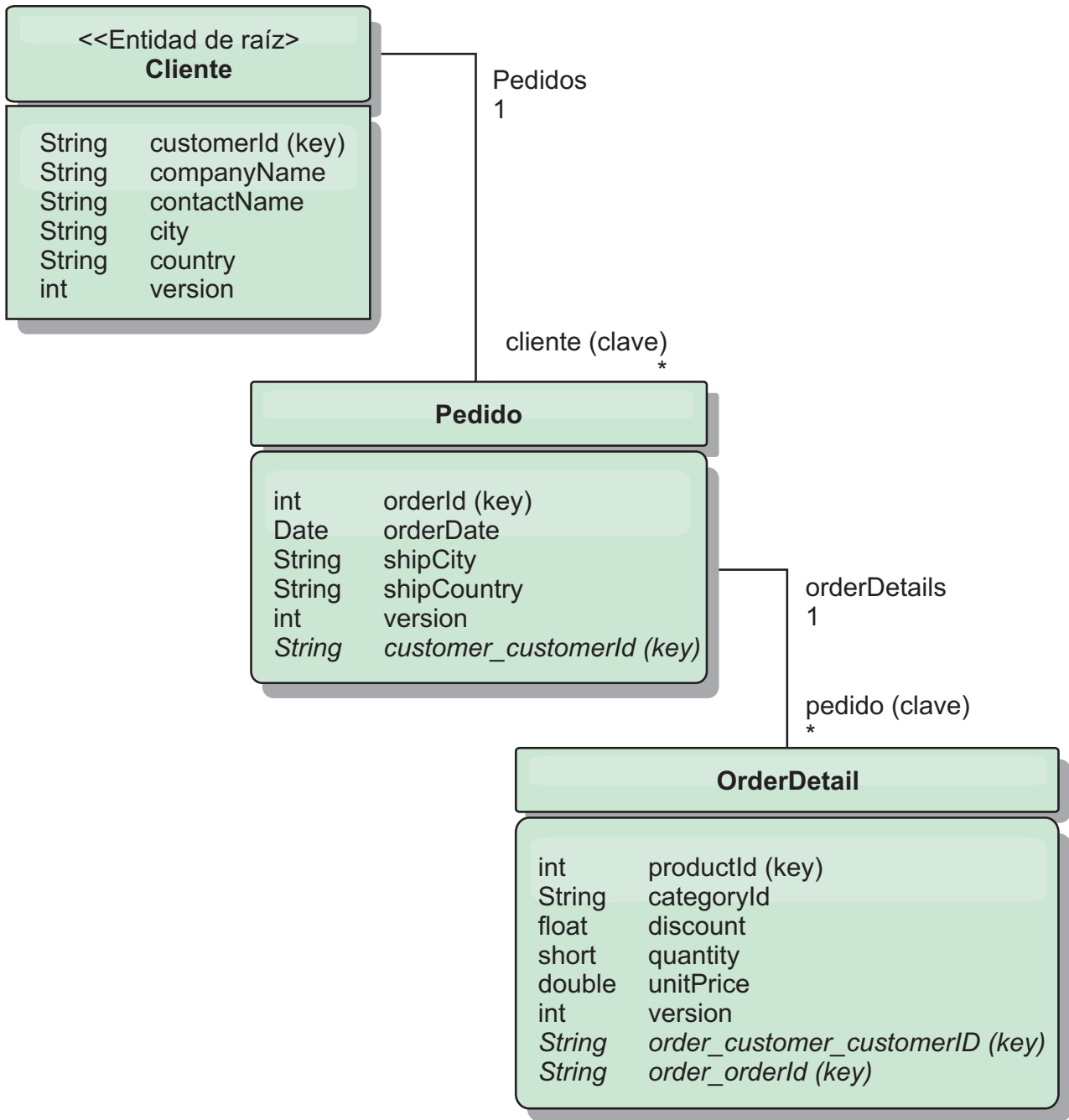
Figura 46. Diagrama del esquema de entidades Customer y Order
