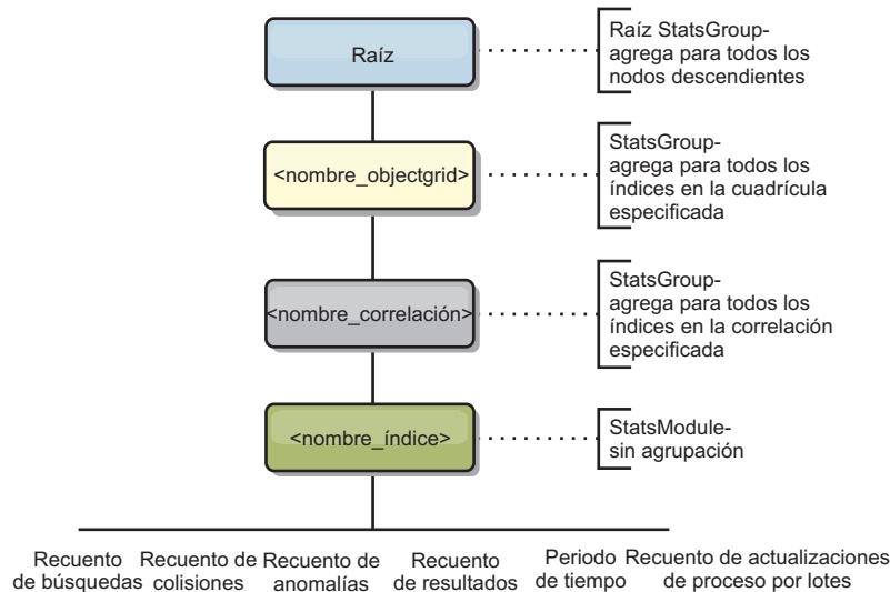
Figura 62. Estructura del módulo hashIndexModule
