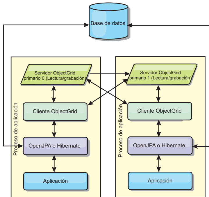
Figura 42. Topología incorporada con particiones JPA
