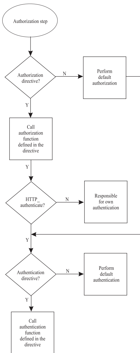
Figura 3. Processo di autorizzazione e autenticazione del server proxy
