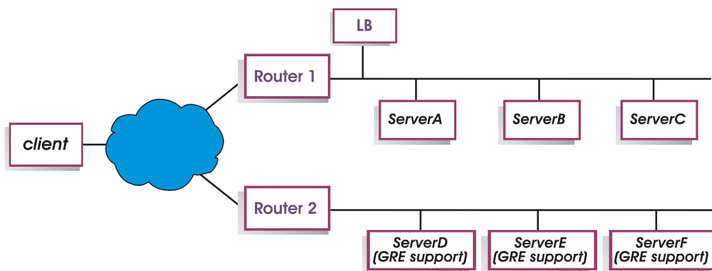
Figure 38. Exemple de configuration en réseau étendu avec une plateforme serveur prenant en charge GRE
