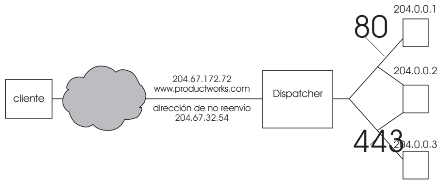
Figura 15. Ejemplo de las direcciones IP necesarias para la máquina Dispatcher
