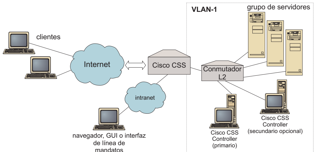
Figura 27. Ejemplo de consultor (con el asociado de alta disponibilidad opcional), configurado detrás del conmutador con la interfaz de usuario delante del conmutador
