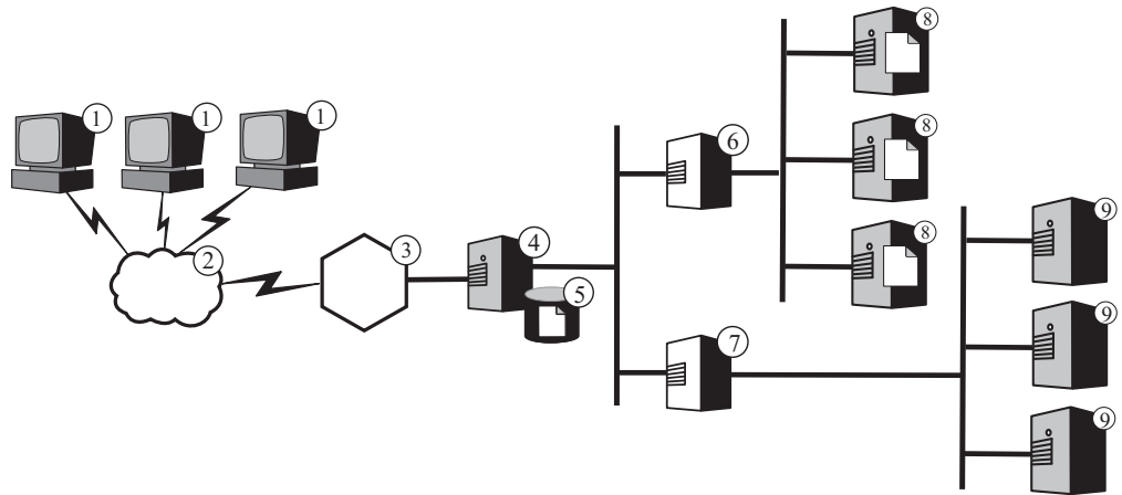
图 8. 对使用 CBR 路由的 HTTP 请求进行负载均衡. 图注: 1—客户机 2—因特网 3—路由器/网关 4—高速缓存代理和 Load Balancer 的 CBR 组件 5—高速缓存 6, 7—Load Balancer 8—内容主机 9—Web 服务器
