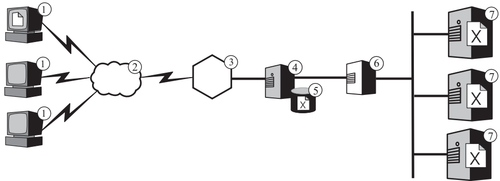
图 2. 高速缓存代理充当负载均衡集群的代理服务器。图注：1—客户机 2—因特网 3—路由器/网关 4—高速缓存代理 5—高速缓存 6—Load Balancer 7—内容主机
