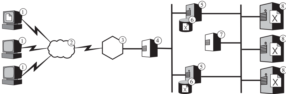
图 4. 负载均衡多个代理服务器和内容主机. 1—客户机 2—因特网 3—路由器/网关 4—分派器 5—高速缓存代理 6—高速缓存 7—分派器 8—内容主机
