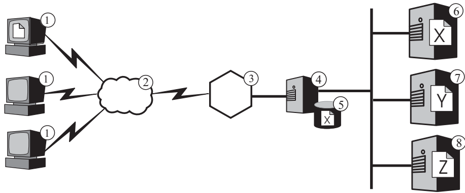
图 7. 使用 CBR 对 HTTP 请求进行路由. 图注: 1—客户机 2—因特网 3—路由器 / 网关 4—高速缓存代理和 Load Balancer 的 CBR 组件 5—高速缓存 6, 7, 8—内容主机
