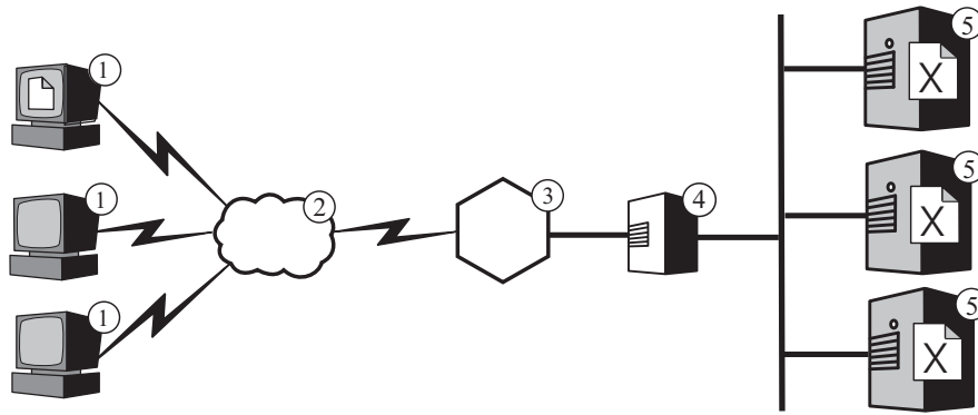
图 3. 对多个内容主机进行负载均衡. 图注: 1—客户机 2—因特网 3—路由器/网关 4—分派器 5—内容主机
