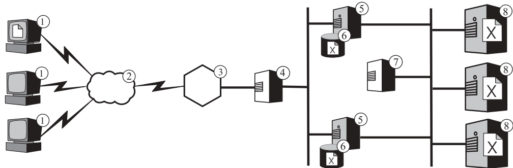
그림 4. 여러 개의 프록시 서버 및 콘텐츠 호스트 로드 밸런싱 1—클라이언트 2—인터넷 3—라우터/게이트웨이 4—Dispatcher 5—Caching Proxy 6—캐시 7—Dispatcher 8—콘텐츠 호스트
