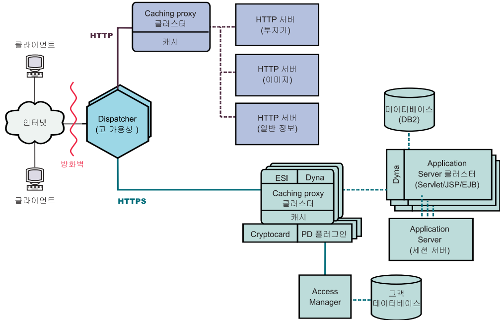
그림 10. B2C 네트워크(2단계)
