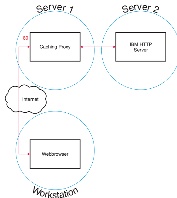
Abbildung 14. Beispiel für ein Caching-Proxy-Netz
