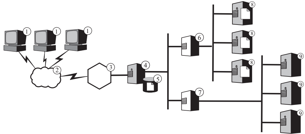
Abbildung 8. Mit CBR weitergeleitete HTTP-Anforderungen verteilen. Legende: 1—Client 2—Internet 3—Router/Gateway 4—Caching Proxy und die Komponente CBR von Load Balancer 5—Cache 6, 7—Load Balancer 8—Inhaltshost 9—Webserver
