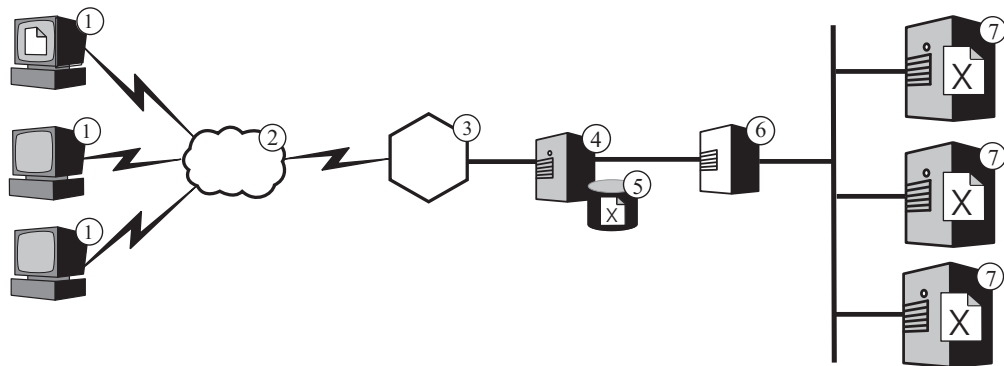
Abbildung 2. Caching Proxy als Proxyserver für einen Cluster mit Lastausgleich. Legende: 1—Client 2—Internet 3—Router/Gateway 4—Caching Proxy 5—Cache 6—Load Balancer 7—Inhaltshost
