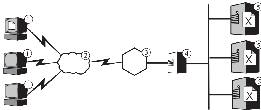
Abbildung 3. Lastausgleich für mehrere Inhaltshosts. Legende: 1—Client 2—Internet 3—Router/Gateway 4—Dispatcher 5—Inhaltshost
