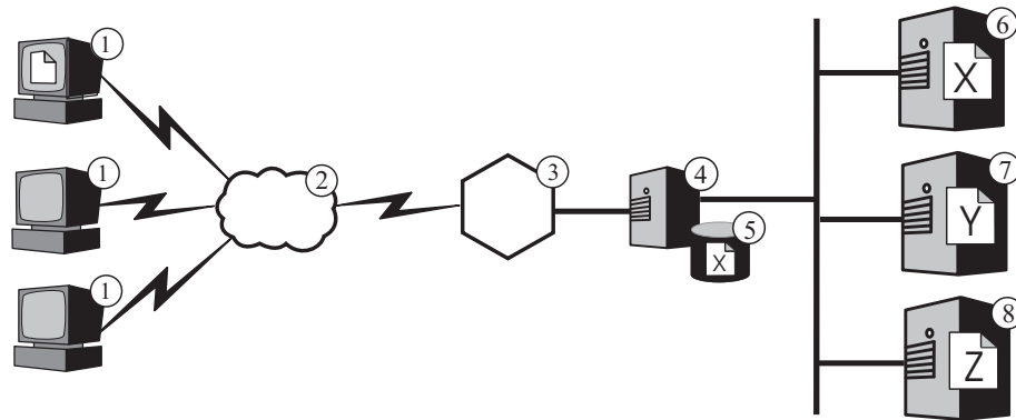
Abbildung 7. Routing von HTTP-Anforderungen mit CBR. Legende: 1—Client 2—Internet 3—Router/Gateway 4—Caching Proxy und die Komponente CBR von Load Balancer 5—Cache 6, 7, 8—Inhaltshost
