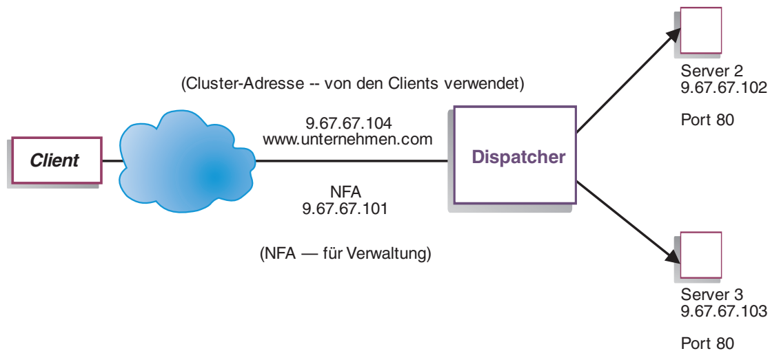
Abbildung 15. Beispiel für ein Load-Balancer-Netz
