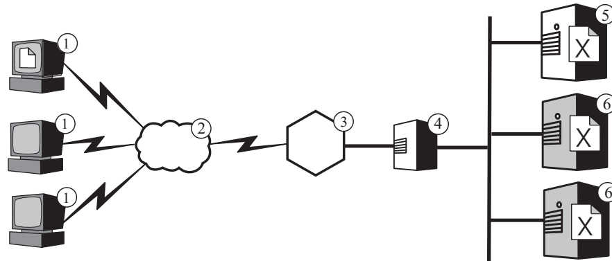
Abbildung 6. Installation eines Backup-Load-Balancer auf einem Inhaltshost. Legende: 1—Client 2—Internet 3—Router/Gateway 4—Primärer Dispatcher 5—Backup-Dispatcher und Inhaltshost 6—Inhaltshost
