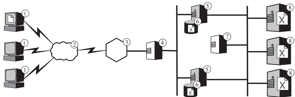
Abbildung 4. Lastausgleich für mehrere Proxyserver und Inhaltshosts. Legende: 1—Client 2—Internet 3—Router/Gateway 4—Dispatcher 5—Caching Proxy 6—Cache 7—Dispatcher 8—Inhaltshost
