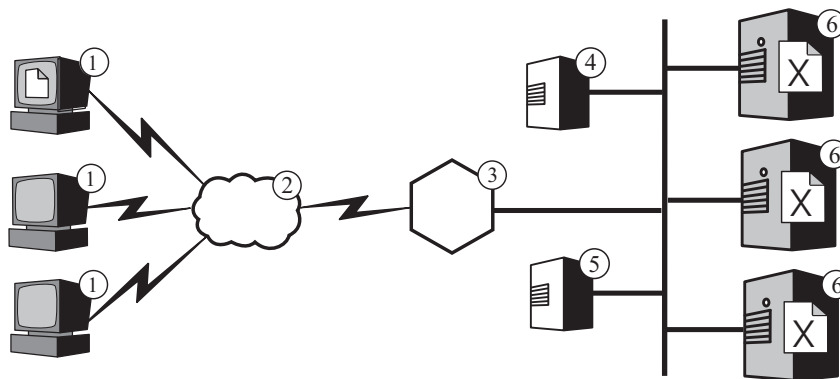
Abbildung 5. Verwendung eines primären und eines Backup-Load-Balancer, um die Verfügbarkeit von Webinhalten zu erhöhen. Legende: 1—Client 2—Internet 3—Router/Gateway 4—Primärer Dispatcher 5—Backup-Dispatcher 6—Inhaltshost
