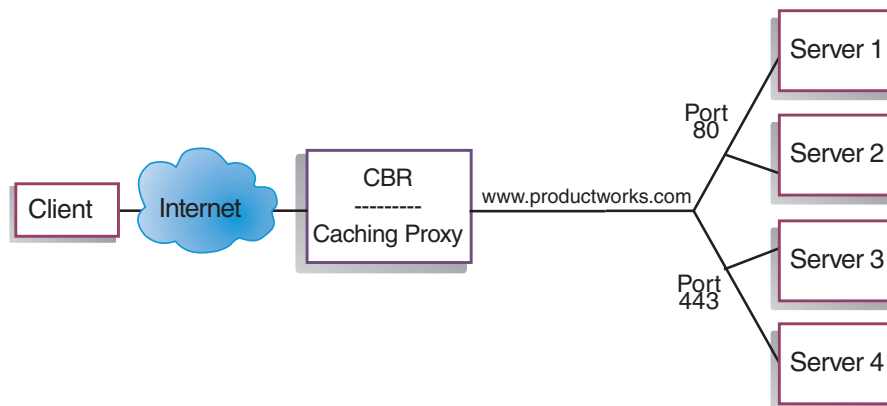
Abbildung 17. CBR-Beispielkonfiguration mit einem Cluster und zwei Ports
