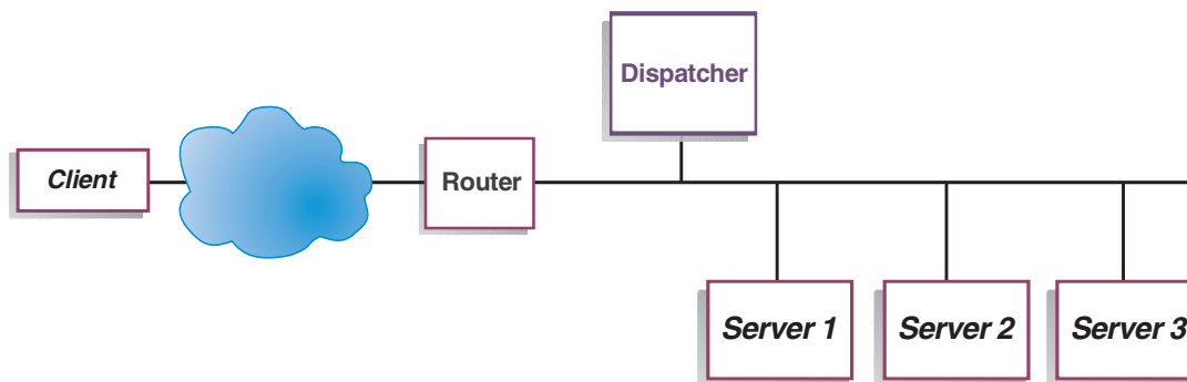
Abbildung 35. Beispiel einer Konfiguration mit einem LAN-Segment
