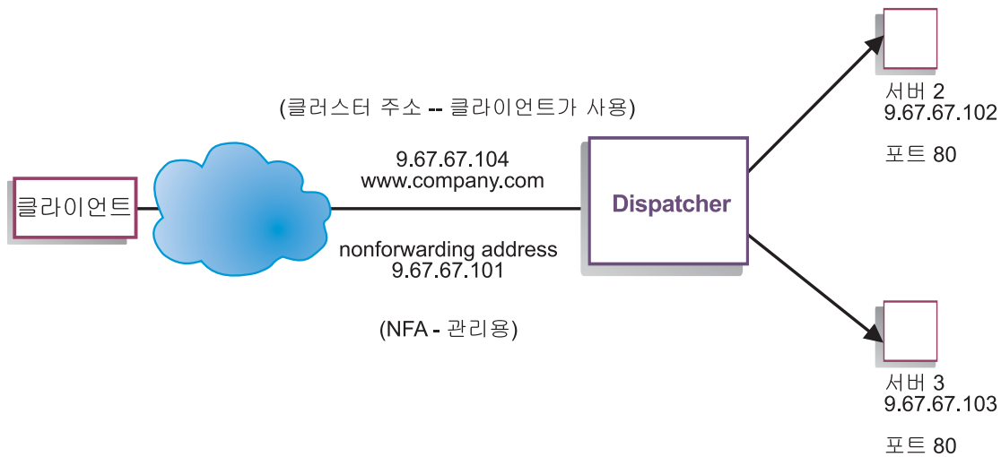
그림 15. Load Balancer 데모 네트워크
