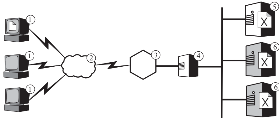
그림 6. 콘텐츠 호스트에서 백업 Load Balancer 찾기. 범례: 1—클라이언트 2—인터넷 3—라우터/게이트웨이 4—1차 Dispatcher 5—백업 Dispatcher 및 콘텐츠 호스트 6—콘텐츠 호스트
