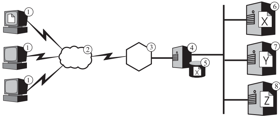
그림 7. CBR로 HTTP 요청 경로 지정. 범례: 1—클라이언트 2—인터넷 3—라우터/게이트웨이 4—Caching Proxy 및 Load Balancer의 CBR 구성요소 5—캐시 6, 7, 8—콘텐츠 호스트
