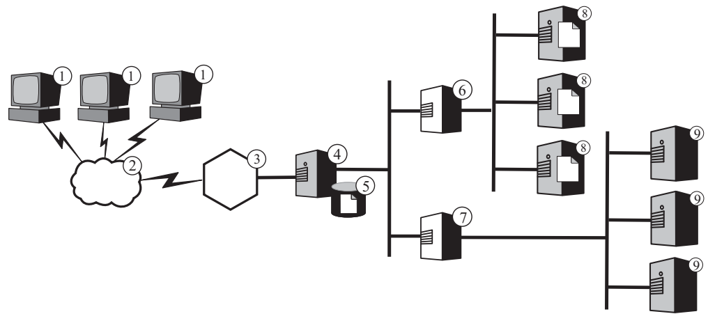
그림 8. CBR로 라우트된 HTTP 요청의 로드 밸런스 범례: 1—클라이언트 2—인터넷 3—라우터/게이트웨이 4—Caching Proxy 및 Load Balancer의 CBR 구성요소 5—캐시 6, 7—Load Balancer 8—콘텐츠 호스트 9—웹 서버
