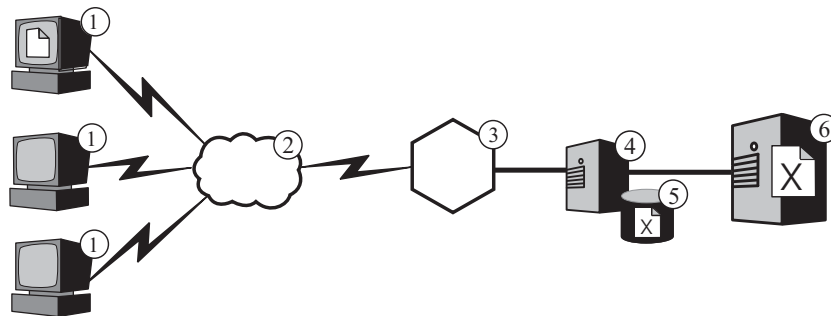
그림 1. 기본 프록시 구성. 범례: 1—클라이언트 2—인터넷 3—라우터/게이트웨이 4—Caching Proxy 5—캐시 6—콘텐츠 호스트
