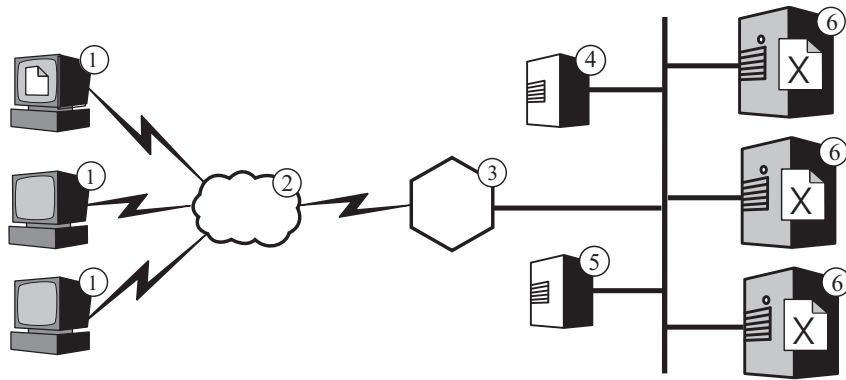
그림 5. 웹 콘텐츠를 고도로 사용 가능하게 하기 위한 기본 및 백업 Load Balancer 사용법. 범례: 1—클라이언트 2—인터넷 3—라우터/게이트웨이 4—1차 Dispatcher 5—백업 Dispatcher 6—콘텐츠 호스트
