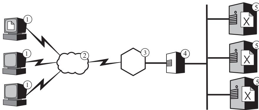
그림 3. 여러 개의 콘텐츠 호스트 로드 밸런싱 범례: 1—클라이언트 2—인터넷 3—라우터/게이트웨이 4—Dispatcher 5—콘텐츠 호스트
