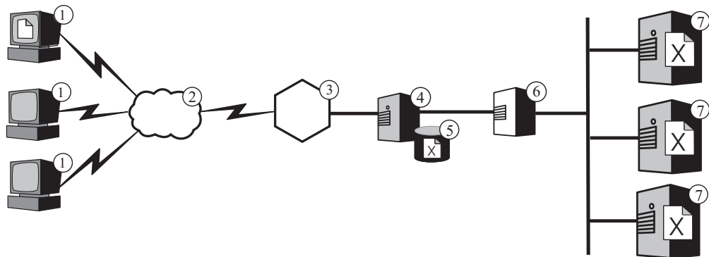
그림 2. 로드 밸런스 클러스터에 대해 프록시 서버의 역할을 하는 Caching Proxy. 범례: 1—클라이언트 2—인터넷 3—라우터/게이트웨이 4—Caching Proxy 5—캐시 6—Load Balancer 7—콘텐츠 호스트
