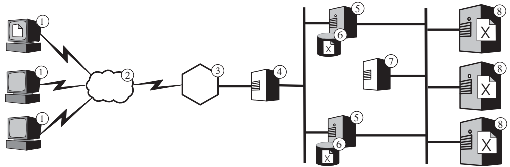
그림 4. 여러 개의 프록시 서버 및 콘텐츠 호스트 로드 밸런스 1—클라이언트 2—인터넷 3—라우터/게이트웨이 4—Dispatcher 5—Caching Proxy 6—캐시 7—Dispatcher 8—콘텐츠 호스트
