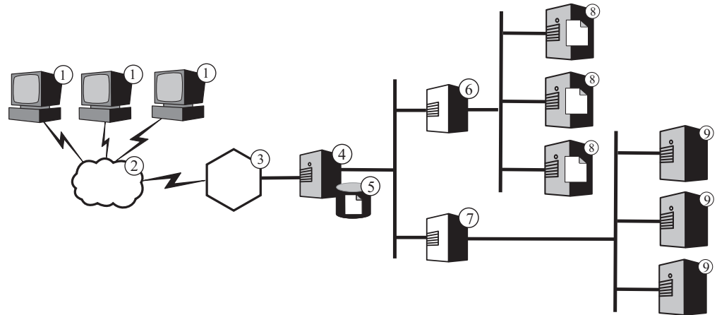
図8. CBR により経路指定された HTTP 要求のロード・バランシング：(凡例: 1—クライアント 2—インターネット 3—ルーター / ゲートウェイ 4—Caching Proxy と Load Balancer の CBR コンポーネント 5—キャッシュ 6, 7—Load Balancer 8—コンテンツ・ホスト 9—Web サーバー)
