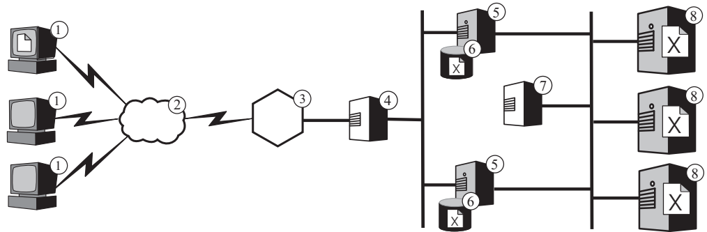
図4. 複数のプロキシ・サーバーおよびコンテンツ・ホストのロード・バランスング：(1—クライアント 2—インターネット 3—ルーター / ゲートウェイ 4—Dispatcher 5—Caching Proxy 6—キャッシュ 7—Dispatcher 8—コンテンツ・ホスト)
