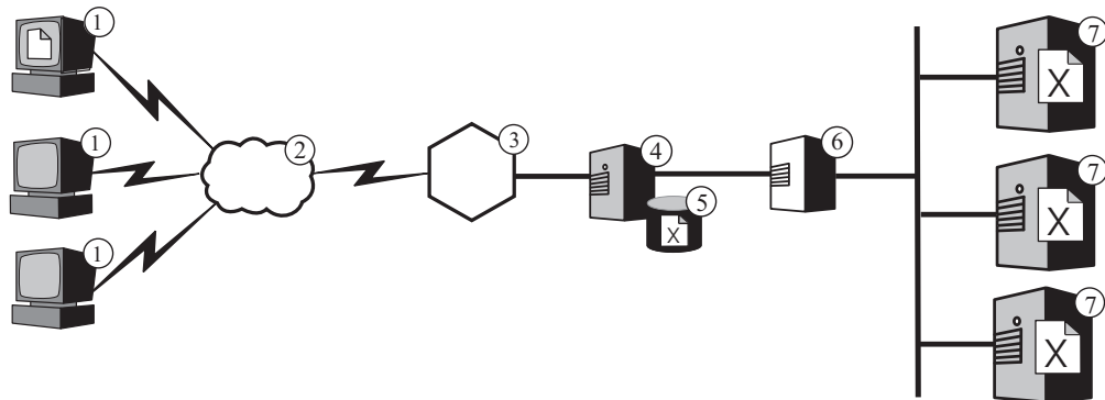
図2. ロード・balancingの対象となるクラスターのプロキシー・サーバーとして機能する Caching Proxy : (凡例: 1—クライアント 2—インターネット 3—ルーター / ゲートウェイ 4—Caching Proxy 5—キャッシュ 6—Load Balancer 7—コンテンツ・ホスト)
