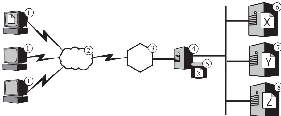
図7. CBR による HTTP 要求の経路指定：(凡例: 1—クライアント 2—インターネット 3—ルーター / ゲートウェイ 4—Caching Proxy と Load Balancer の CBR コンポーネント 5—キャッシュ 6、7、8—コンテンツ・ホスト)
