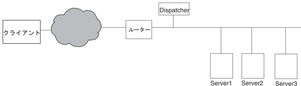
図 35. 単一の LAN セグメントから構成される構成の例
