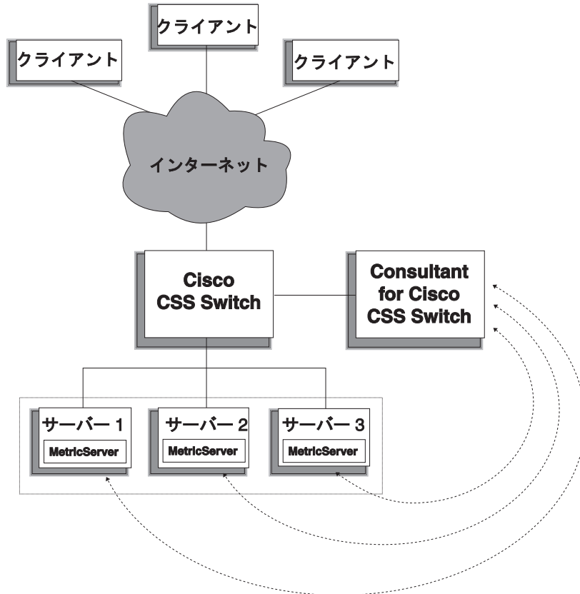
図6. Cisco CSS Controller および Metric Server を使用してローカル・サービスを管理するサイトの例
