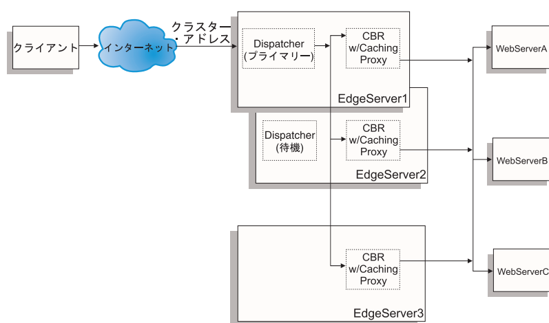
図 46. Dispatcher、CBR、および Caching Proxy を使用する 2 層ハイ・アベイラビリティ構成例
