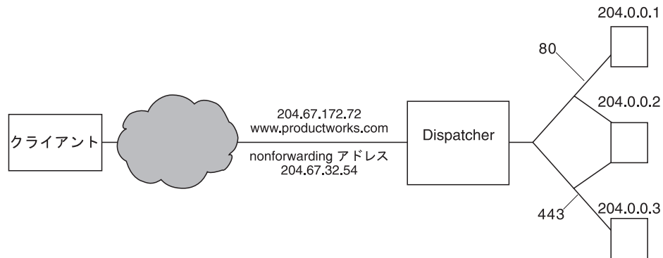
図 15. Dispatcher マシンに必要な IP アドレスの例
