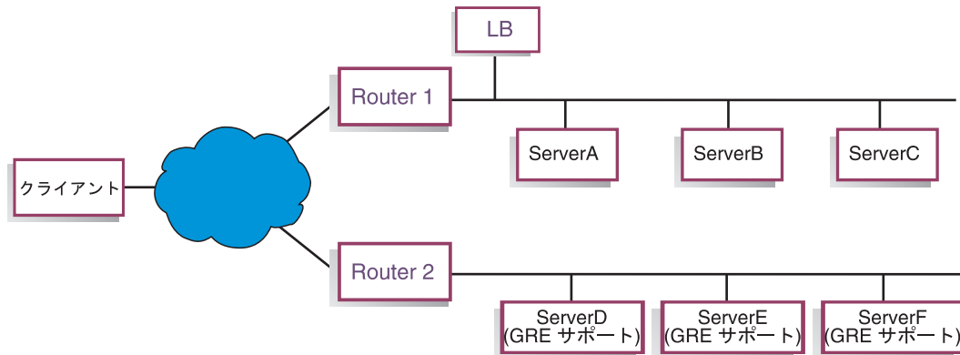
図 38. GRE をサポートするサーバー・プラットフォームがある広域の例の構成
