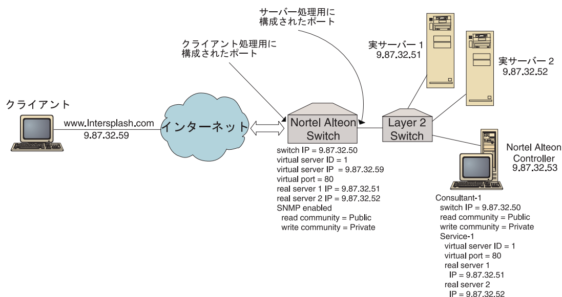
図 28. 単純な Nortel Alteon Controller 構成
