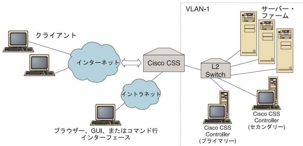
図 27. ユーザー・インターフェースはスイッチの前方にして、スイッチの背後で構成されたコンソルタント (オプションのハイ・アベイラビリティ・パートナーと共に) の例
