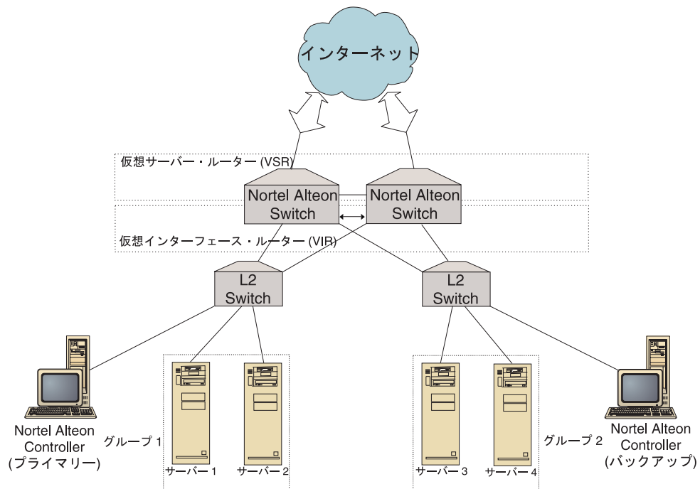
図 33. Nortel Alteon Controller および Nortel Alteon Web Switch ハイ・アベイラビリティの例
